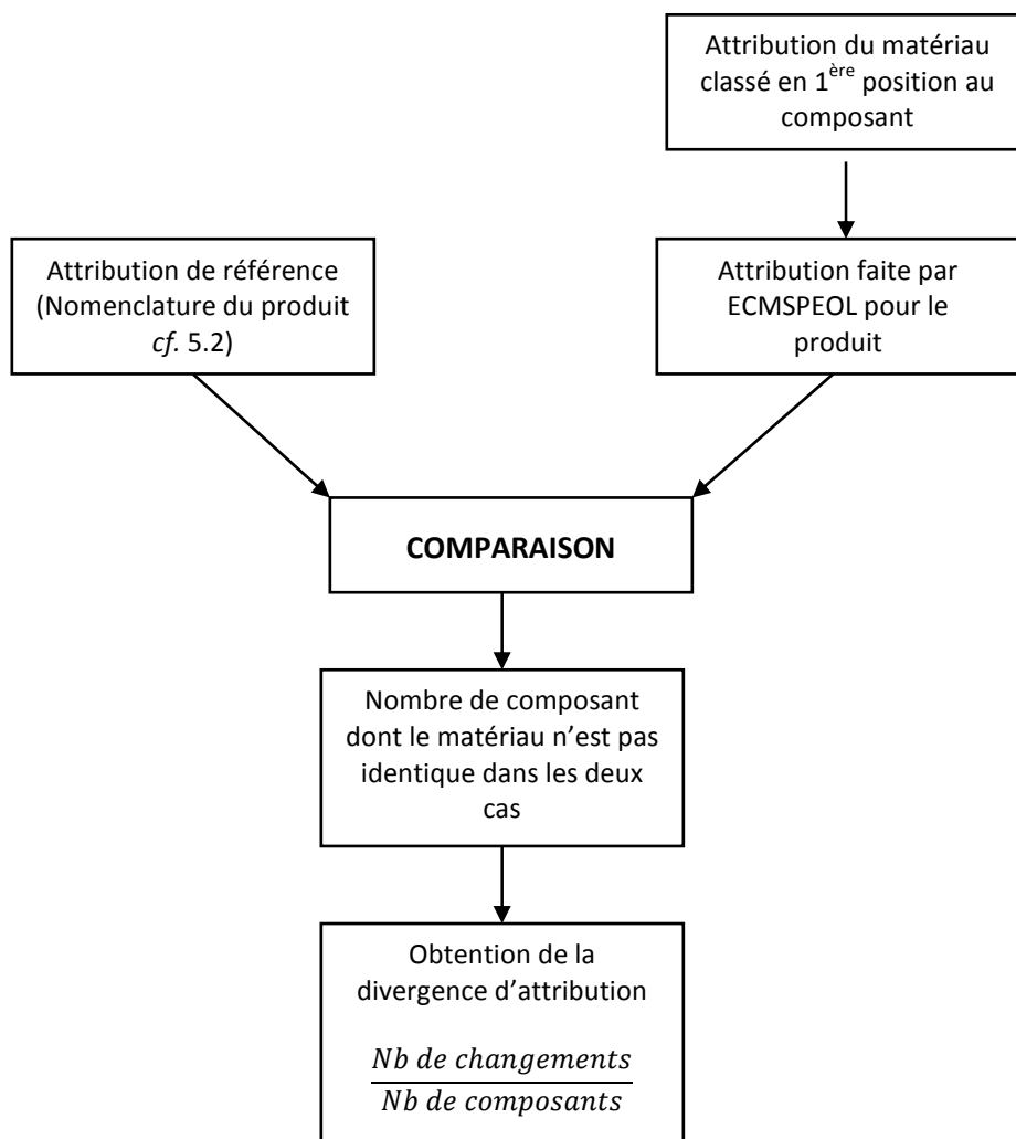
Figure 5.7 : Principe d'évaluation de la divergence d'attribution des matériaux
