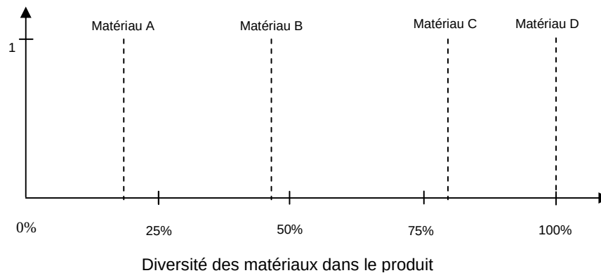
Figure 3.5 : Représentation graphique de la fonction d'appartenance de la diversité des matériaux
