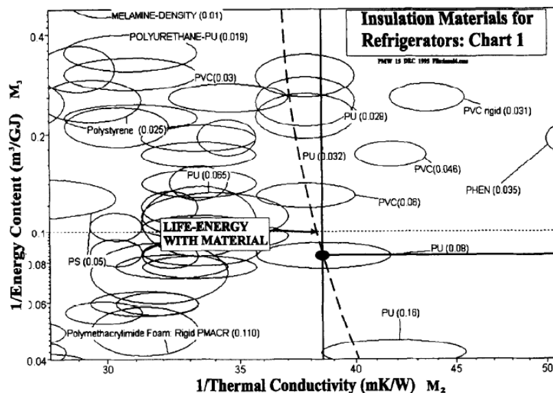
Figure 1.6 : Graphe d'Ashby de sélection des matériaux, [12]
