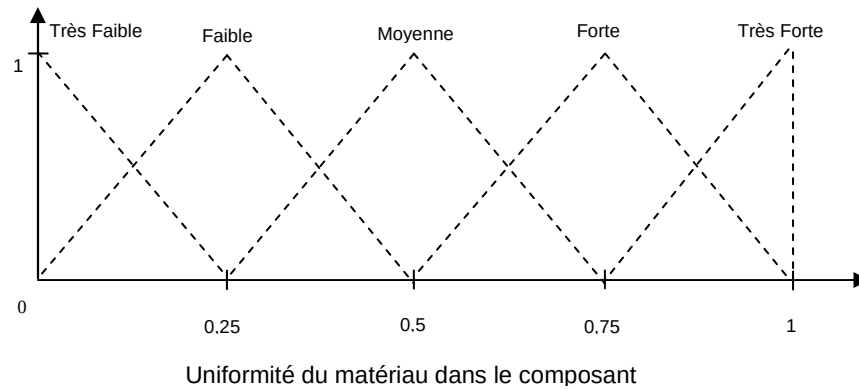
Figure 3.4 : Représentation graphique de la fonction d'appartenance de l'uniformité du matériau dans le composant
