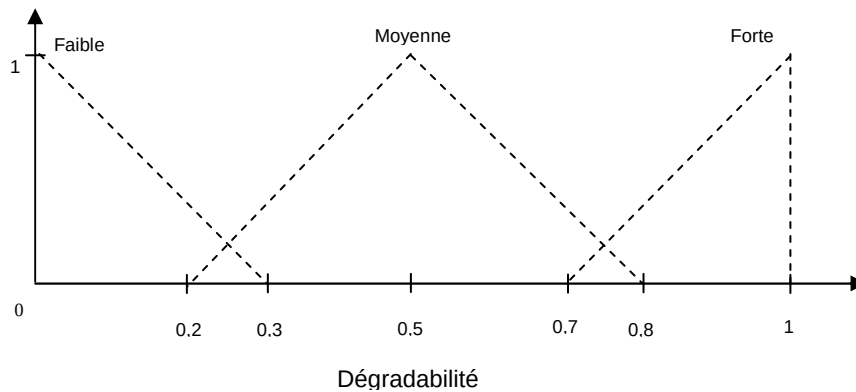
Figure 3.3 : Représentation graphique de la fonction d'appartenance de la dégradabilité
