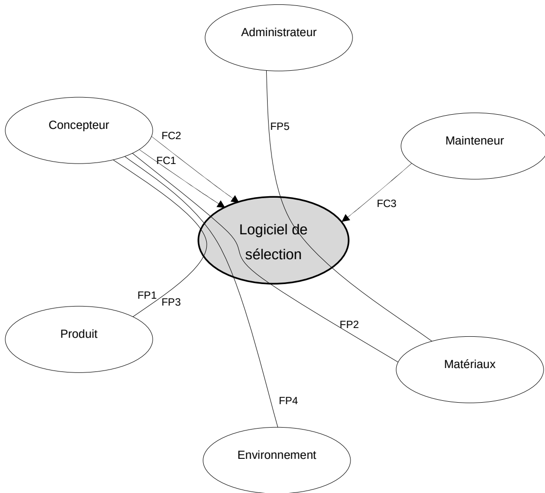
Figure 4.2 : Diagramme des interacteurs du logiciel de sélection des matériaux
