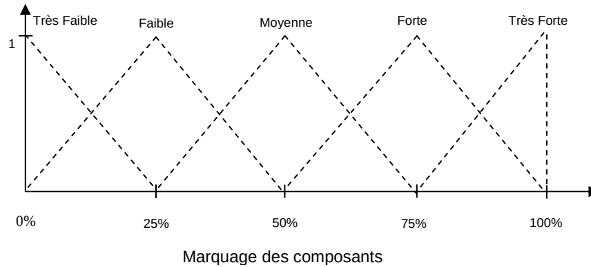
Figure 3.6 : Représentation graphique de la fonction d'appartenance du marquage des composants
