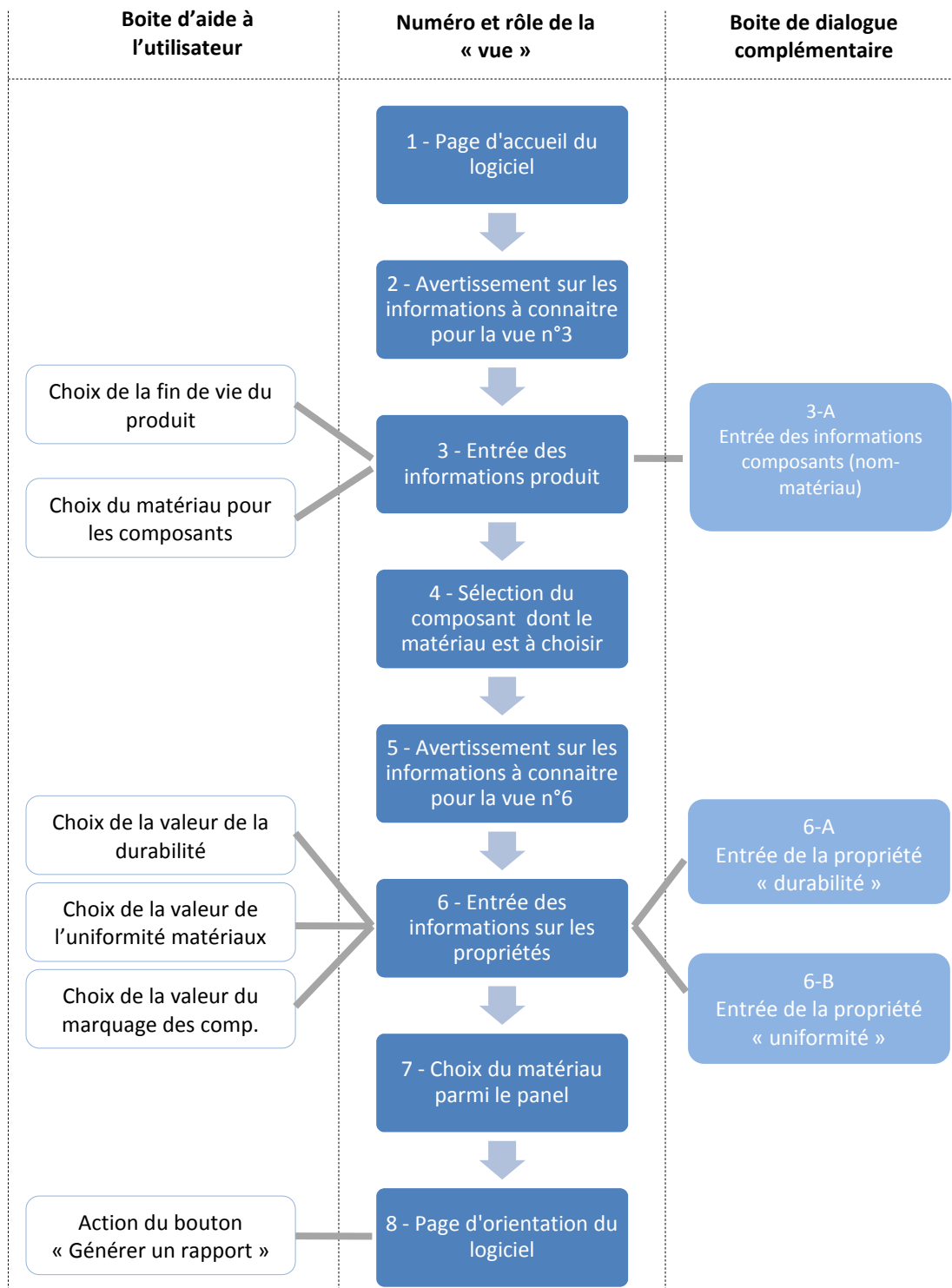
Figure 4.4 : Organigramme des différentes vues et boites de dialogue d'ECMSPEOL
