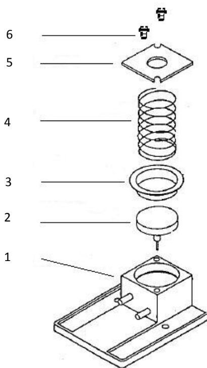
Figure 5.1 : Vérin monostable étudié
