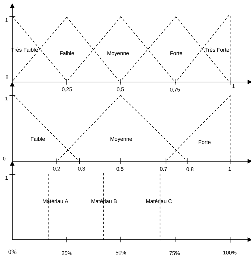
Figure 3.2 : Fonctions d'appartenance typiques utilisée pour la méthode proposée.
