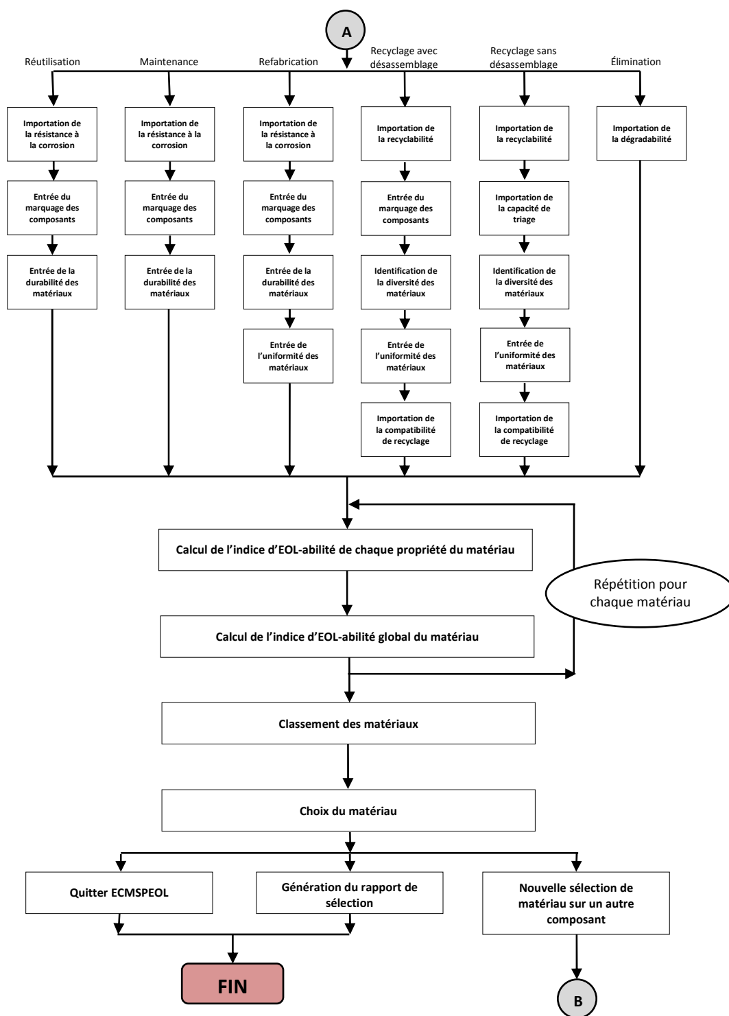
Figure 4.3 : Diagrammes des actions réalisées par ECMSPEOL
