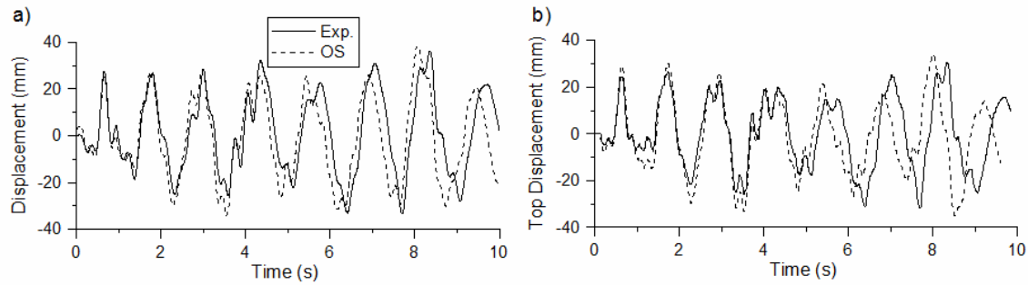
Fig. A.9 : Historique des déplacements du haut des spécimens W1 et W2 sous 100% EQ (a) OS vs essai pour le spécimen W1; (b) OS vs essai pour le spécimen W2
