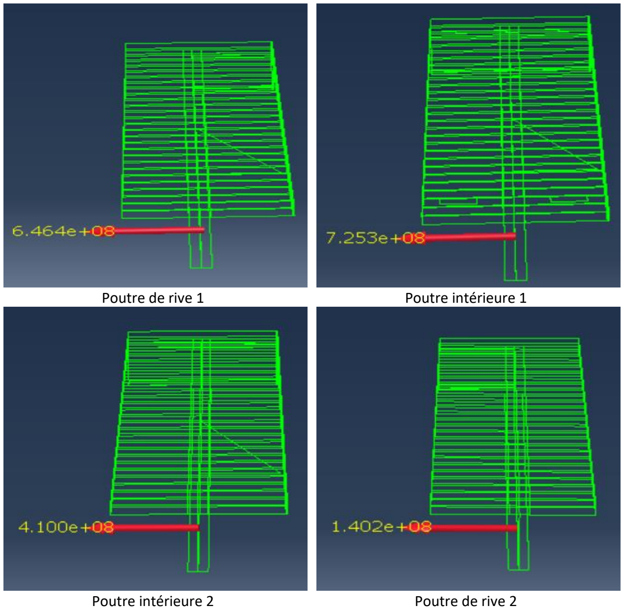
Figure B.16 – Moment fléchissant pour le modèle de pont avec tablier non mixte à platelage transversal
