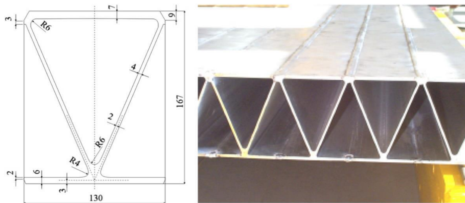
Figure 2.8 : Extrusion développée à l'université de Rzeszow (Burgelin, 2017)
