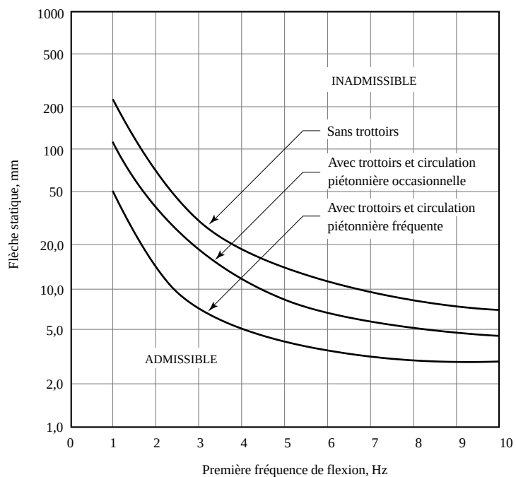
Figure 2.27 : Flèche limite en fonction de la première fréquence de vibration (CSA, S6-14)
