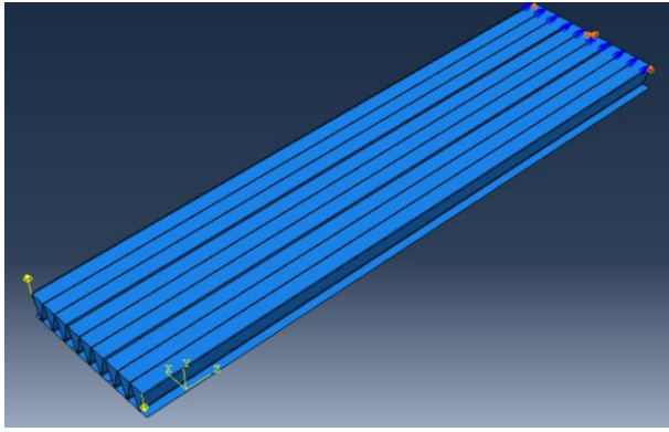
a) Modèle E – Rigidité torsionnelle longitudinale
