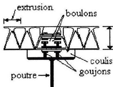
Figure 2.12 : Action mixte (Roy, 1999)
