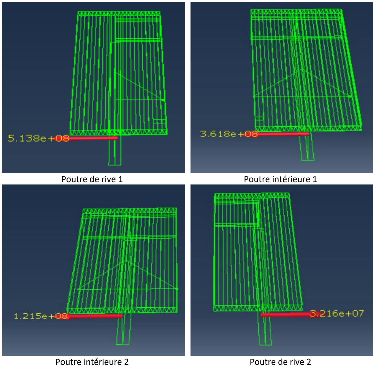
Figure B.11 – Moment fléchissant pour le modèle de pont avec tablier non mixte à platelage longitudinal
