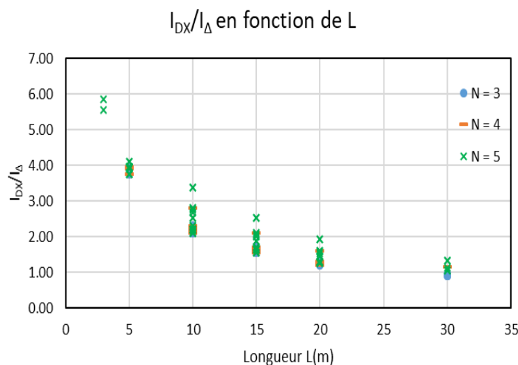
Figure 3.35 : Variation du ratio I_{DX}/I_A en fonction de L
