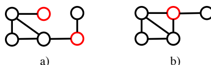
Figure 2.4 Exemple de contraction de nœuds
