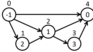
Figure 5.4 Quatrième étape de la construction du graphe sans pertes du fichier log 3.3
