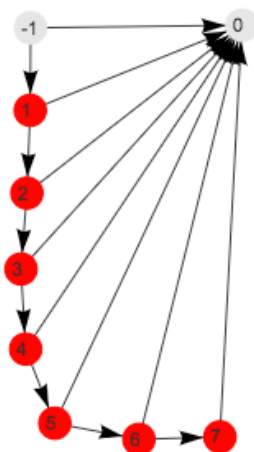
Figure 5.8 Graphe sans pertes du fichier log 5.1
