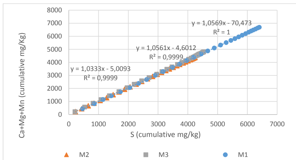
Figure 5.6 : Charges cumulatives normalisées du Ca, Mg et Mn en fonction du S des matériels M1 : Alimentation ; M2 : Rejet (T6) et M3 : Rejet (T9)
