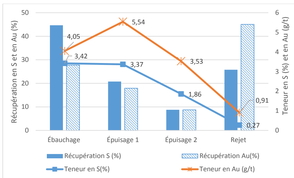
Figure 6.8 : Distribution de l'or et du soufre
