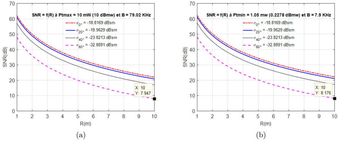
Figure 3.14 SNR en fonction de la distance : (a) à P_{tmax} = 10 \text{ dBmW} , (b) à P_{tmin} = 0.2278 \text{ dBmW}
