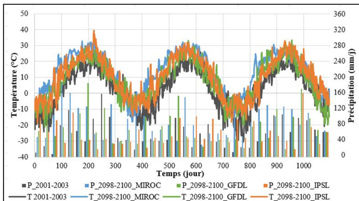
Figure 3.14 : Evolution de la température et des précipitations entre 2001 et 2003 pour le scénario climatique historique et entre 2098 et 2100 pour les trois scénarios de changements climatiques utilisés dans les simulations numériques
