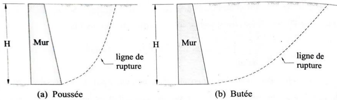
Figure 2-19 : Schéma de rupture verticales (Silvestri, 2011)
