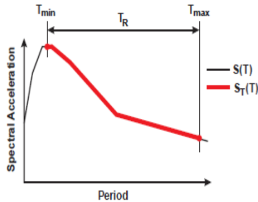
Figure 2-5 : Spectre cible selon la méthode A (Tremblay et al., 2015)
