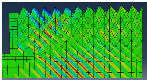
a) Mode 1 ( T=0.132 s) Facteur de participation 0.58%
