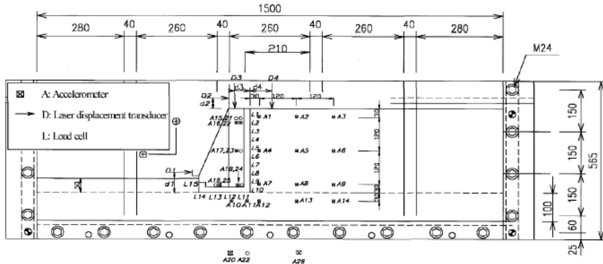
Figure 2-9 : Configuration des tests de Nakumara (2006) (Geraili et Sitar, 2013).
