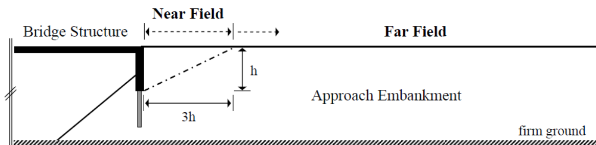
Figure 3-19 : Géométrie de sol à considérer (Carvajal Uribe, 2011)
