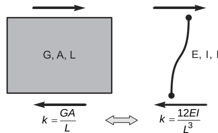
Figure 3-53 : Équivalence entre modèle de sol réel et de celui de poutre en cisaillement
