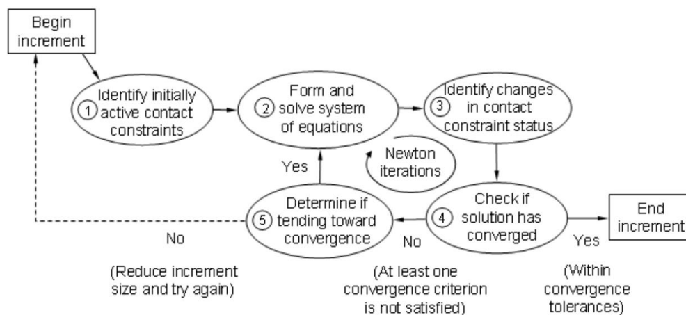
Figure 2-29 : Logique de contact dans ABAQUS/Standard (Simulia, 2011)
