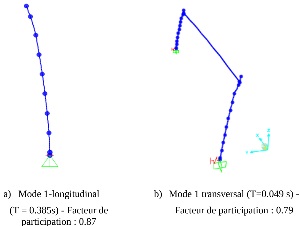
Figure 5-3 : Modes fondamentaux dans la direction longitudinale et transversale du pont sans remblai.
