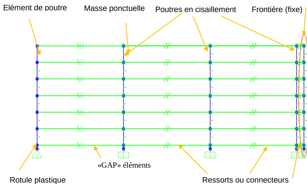
Figure 3-54 : Modèle simplifié du mur et du sol sans contrainte en translation longitudinale à l'interface.
