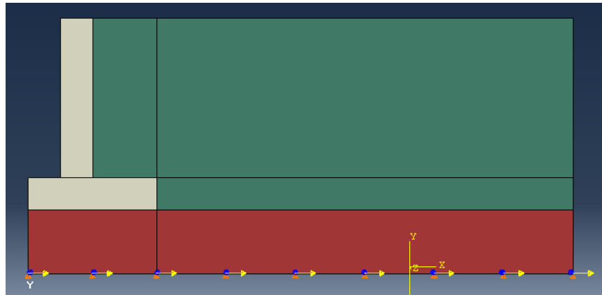
Figure 3-27 : Condition limite de type accélération à la base de la fondation rocheuse
