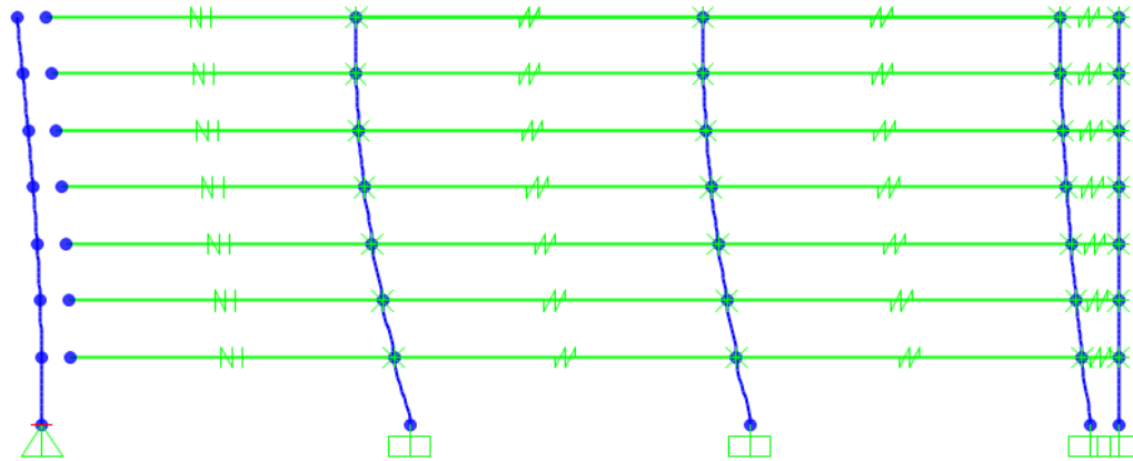
Figure 3-60 : Mode fondamental de la structure
