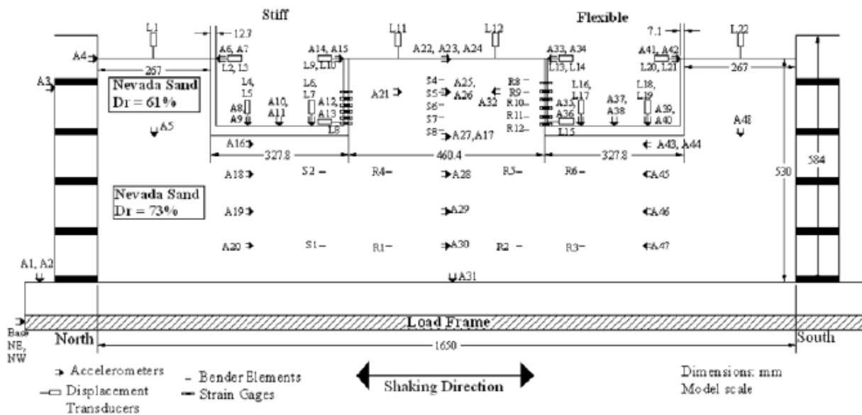
Figure 2-10 : Configuration des tests Al-Atik et Sitar (2008) (Geraili et Sitar, 2013).
