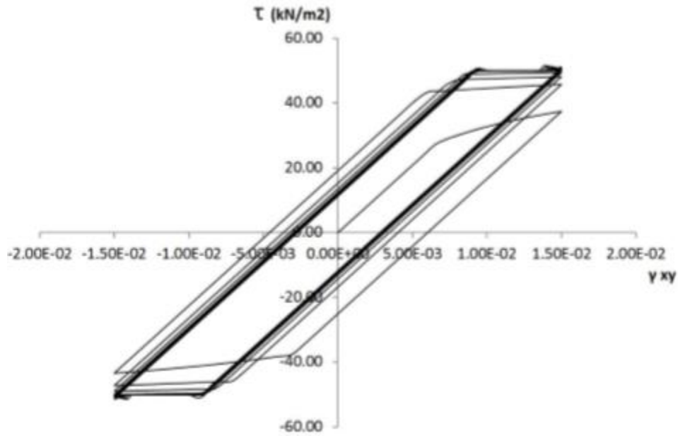
Figure 2-36 : Courbe contrainte-déformation en cisaillement sur un test réalisé avec un modèle de durcissement (Pinto, 2012)
