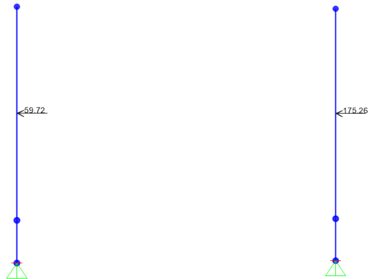
a) Force d'inertie du sol au-dessus de la semelle ( k_h W )
