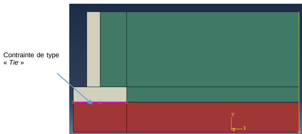
Figure 3-25 : Contrainte de type Tie entre la base du mur et la fondation rocheuse.
