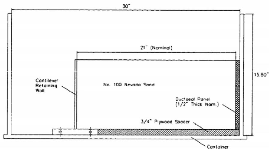
Figure 2-8 : Configuration type des essais de Stadler (1996) (Geraili et Sitar, 2013).
