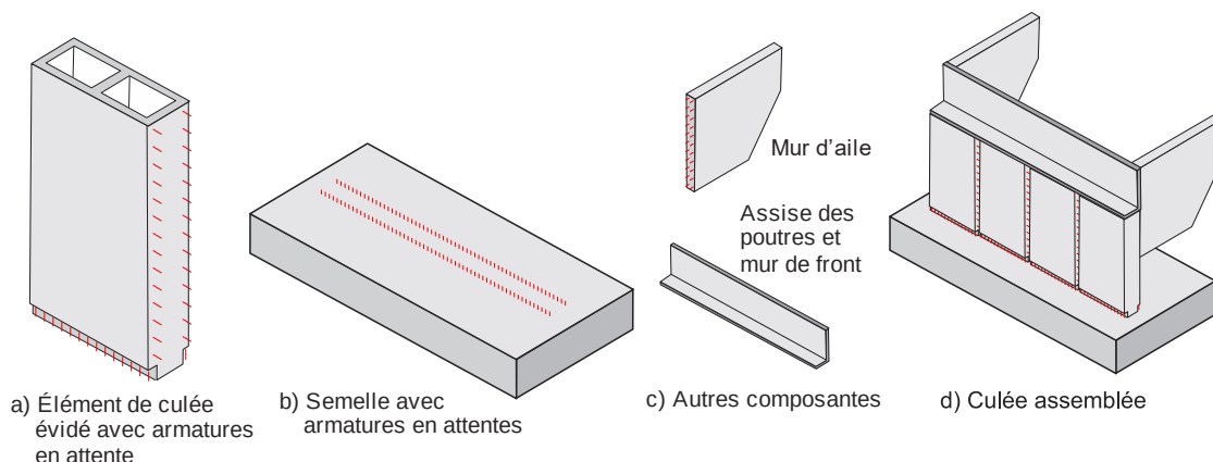
Figure 1-1 : Culée préfabriquée évidée type
