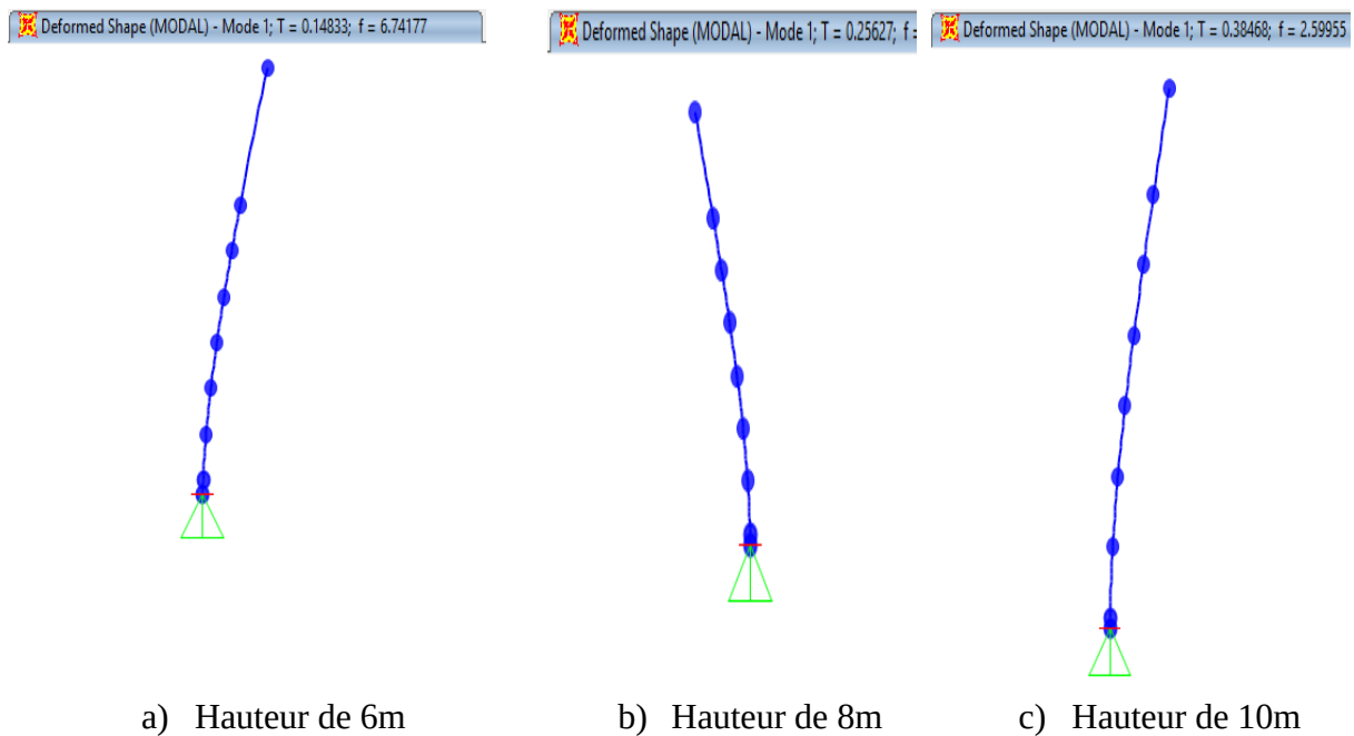
Figure 4-6 : Mode fondamental pour les hauteurs de 6m, 8m et 10 m
