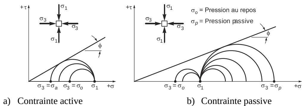
Figure 2-17 : Détermination des contraintes actives et passives sur le cercle Mohr (adapté de ASCE (1994))
