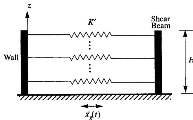
Figure 2-25 : Modèle de Scott (Veletsos et Younan, 1995)
