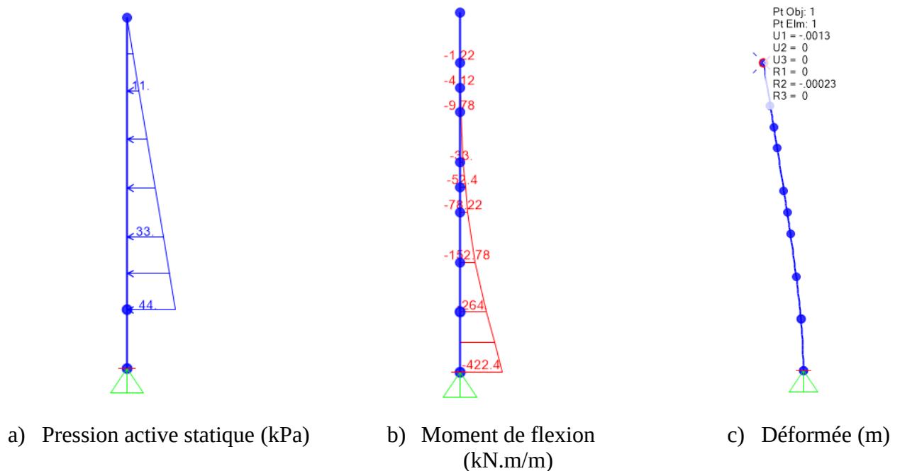
Figure 3-47 : Résultats de l'analyse statique avec SAP2000
