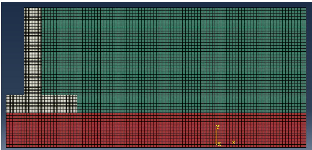
Figure 3-23 : Modèle maillé
