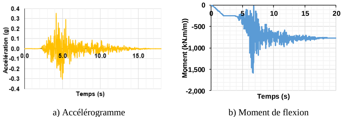
Figure 3-36 : Évolution dans le temps du moment et du déplacement pour le séisme MC7
