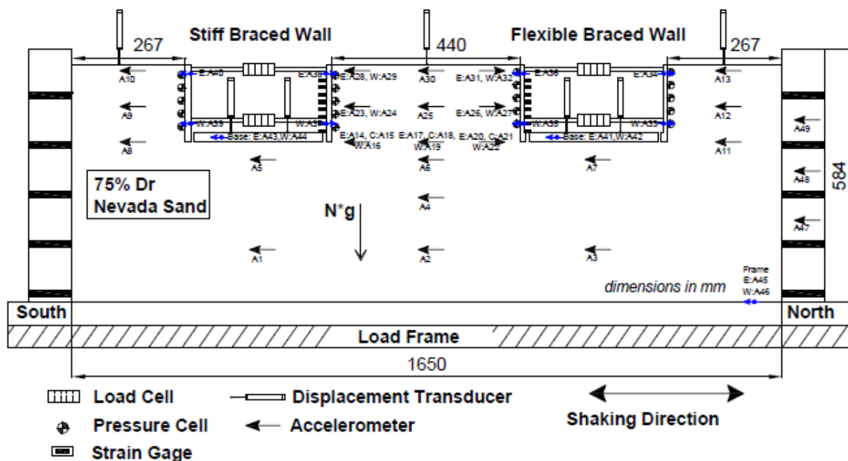
Figure 2-11 : Configuration du modèle ROOZ01, vue de profil (Geraili et Sitar, 2013).
