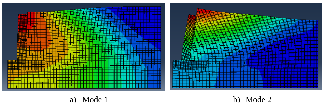
Figure 3-32 : Les deux premiers modes de la structure
