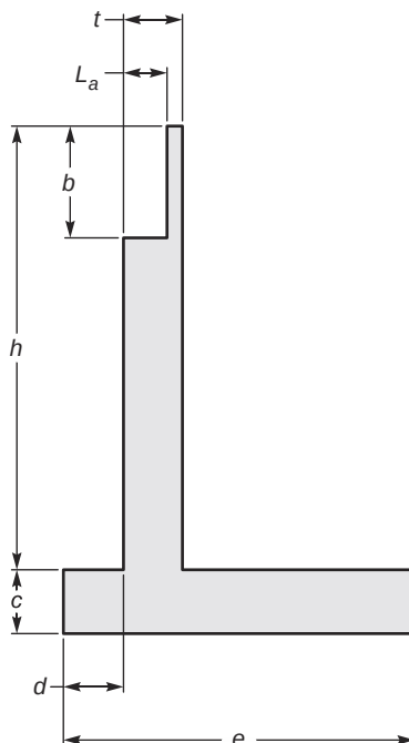
Figure 4-2 : Paramètres définissant la géométrie d'une culée type
