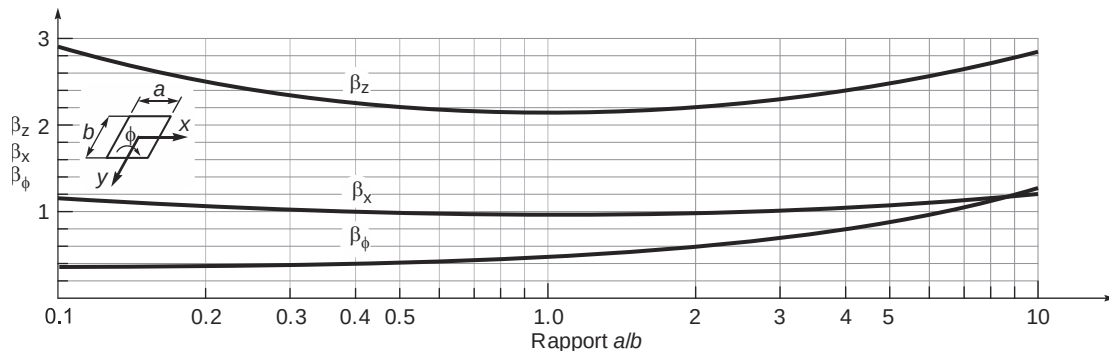
Figure 3-42 : Abaques présentant les coefficients de Newmark selon Davidovici, 1999 (Massicotte, 2019)
