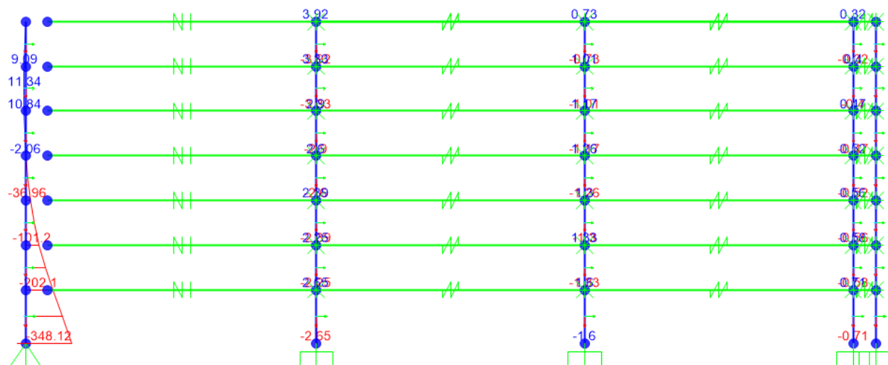
Figure 3-59 : Diagramme du moment de flexion dû à la pression active statique.
