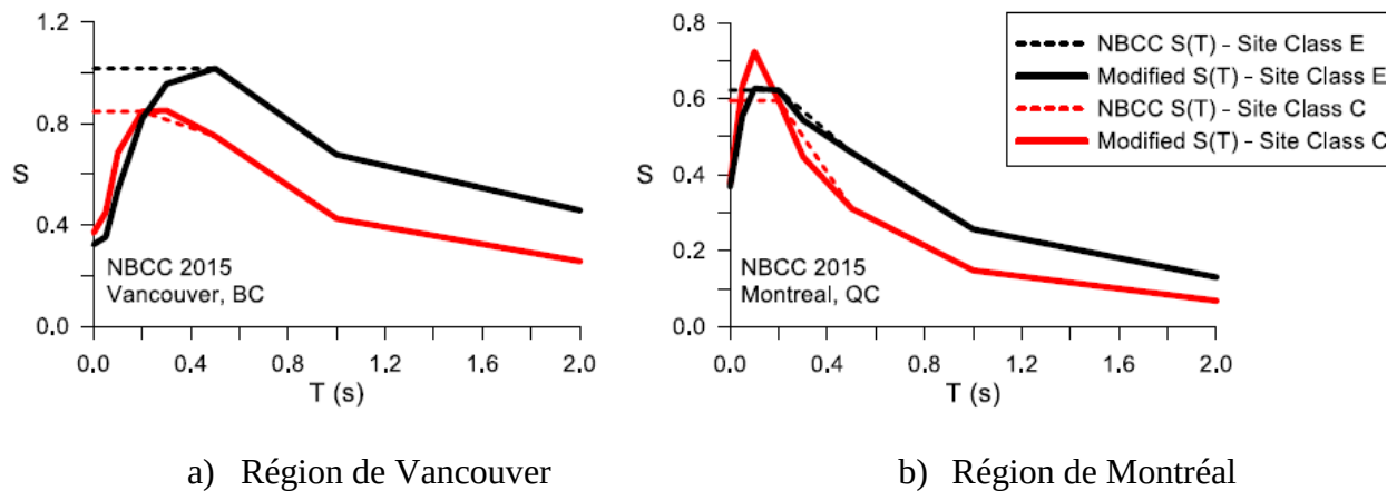
Figure 2-4 : Exemples de spectre de conception et de spectre de conception modifié du CNBC (2015) (Tremblay et al., 2015)
