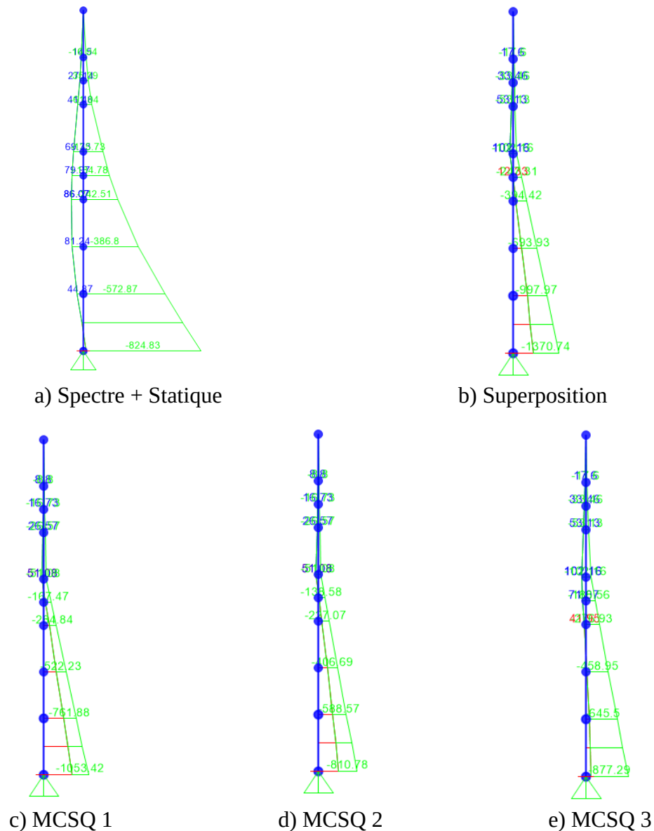
Figure 3-50 : Résultats de l'analyse statique avec SAP2000
