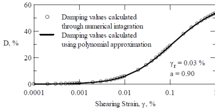
Figure 2-38 : Courbe d'amortissement basée sur le comportement de Masing (Darendeli, 2001).
