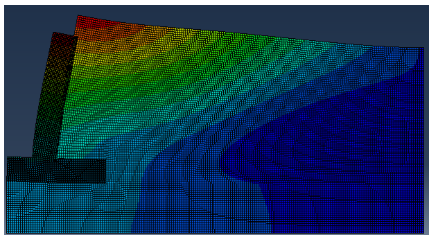
b) Mode 2 ( T=0.086 s) Facteur de participation 57%
