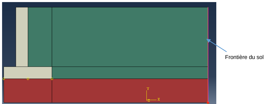
Figure 3-24 : Couplage cinématique dans la direction longitudinale (axe X) de la frontière du sol.
