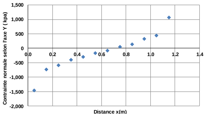
Figure 3-31 : Évolution de la contrainte normale selon l'axe Y le long de la section
