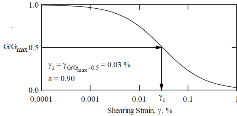
Figure 2-37 : Courbe normalisée du module sécant (sable silteux à une pression de confinement de 1 atm) représentée utilisant un modèle hyperbolique (Darendeli, 2001).
