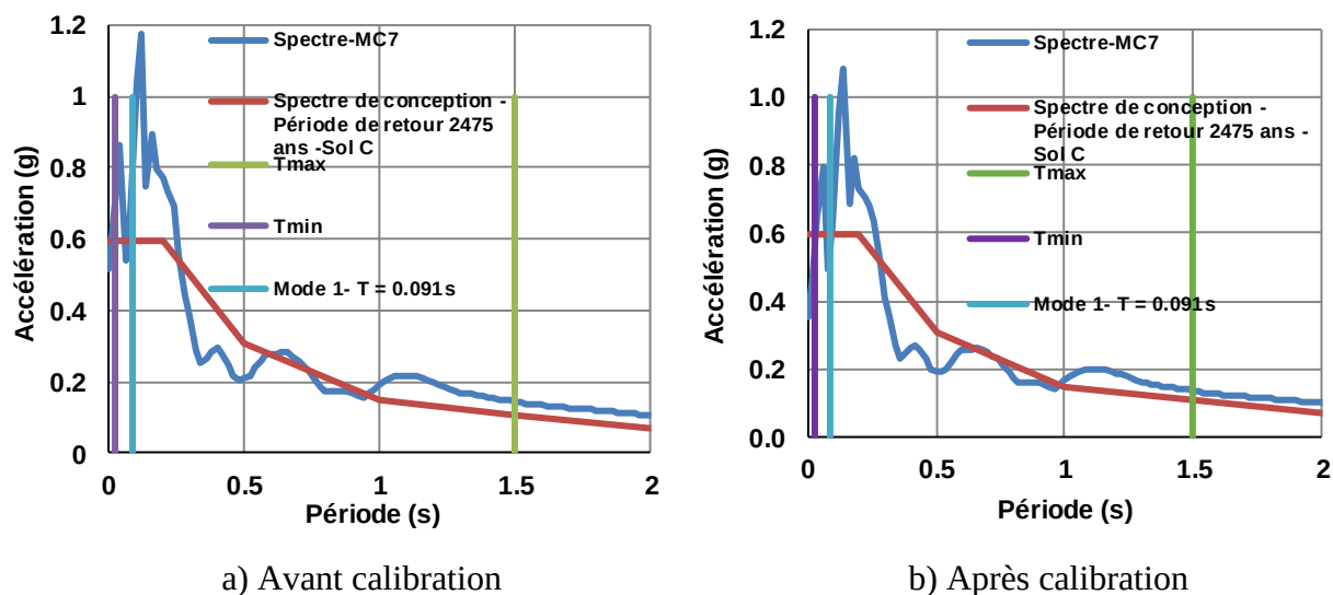
Figure 3-33 : Modification du spectre de réponse du séisme MC7 suite à la calibration
