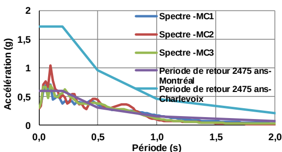
a) Spectre des séismes de MC1 à MC3
