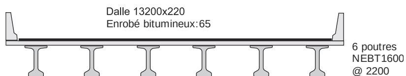
Figure 4-1 : Section transversale du tablier
