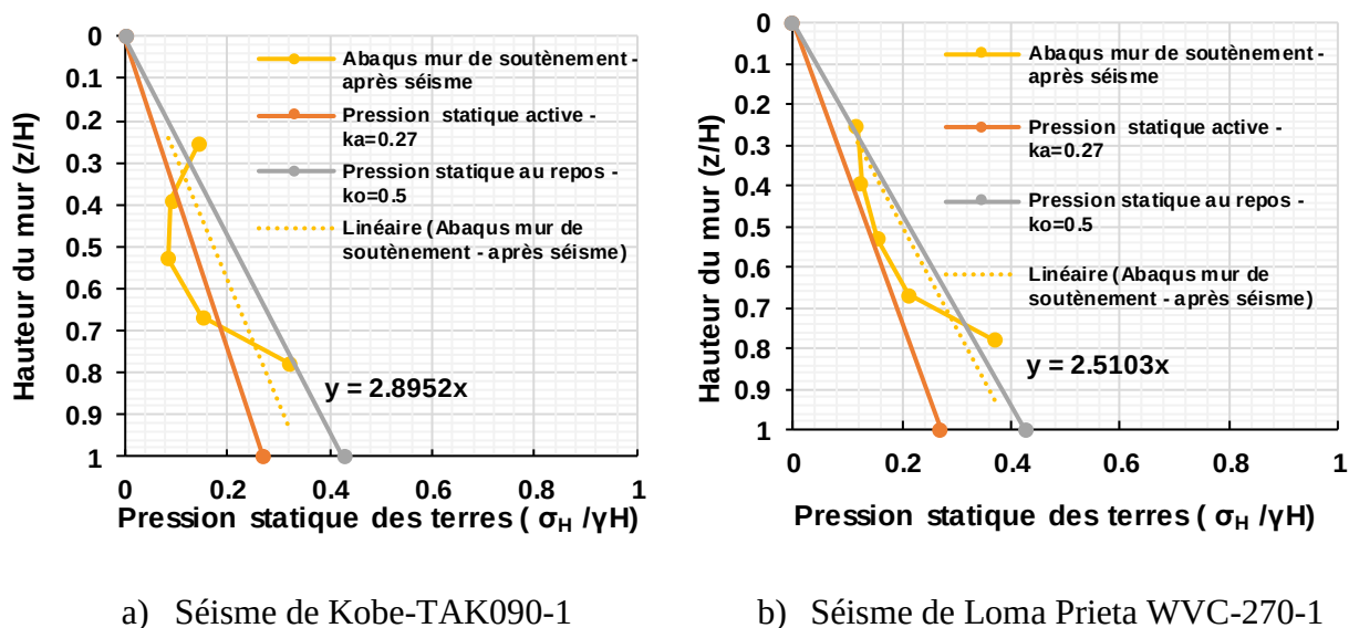
Figure 3-12 : Courbe de tendance issue des profils de pression statique avec ABAQUS
