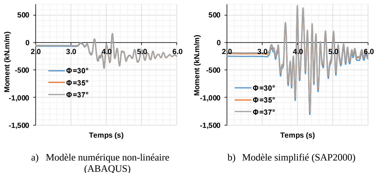
Figure 4-13 : Variation du moment à la base de la culée de 6 m pour le séisme MC1 en fonction de l'angle de frottement interne \phi
