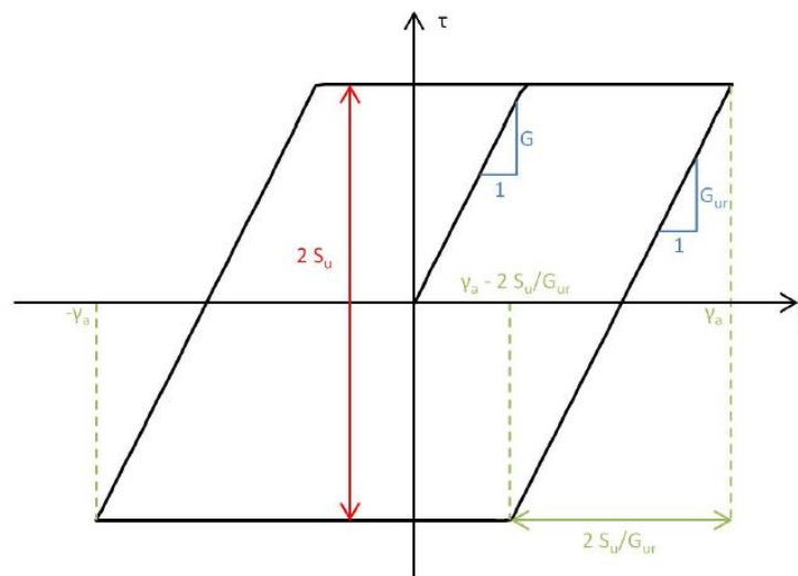
Figure 2-35 : Représentation de la boucle d'hystérésis en conditions non drainées (Pinto, 2012)
