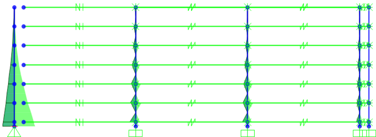
Figure 3-57 : Diagramme du moment de flexion du modèle avec contrainte en translation longitudinale à l'interface.
