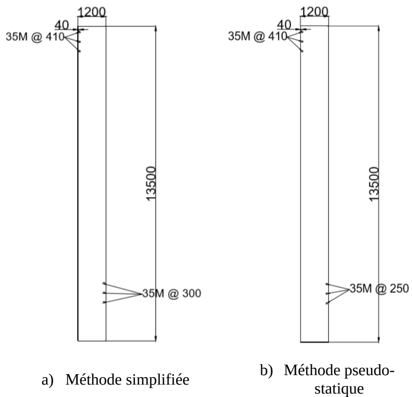
Figure 5-4: Plan des sections ductiles pour la région de Montréal
