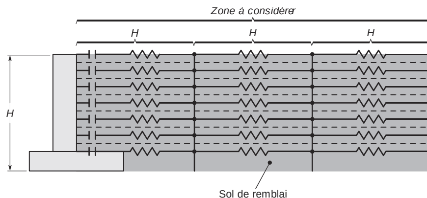
Figure 3-51 : Représentation du volume de sol par 3 poutres en cisaillement
