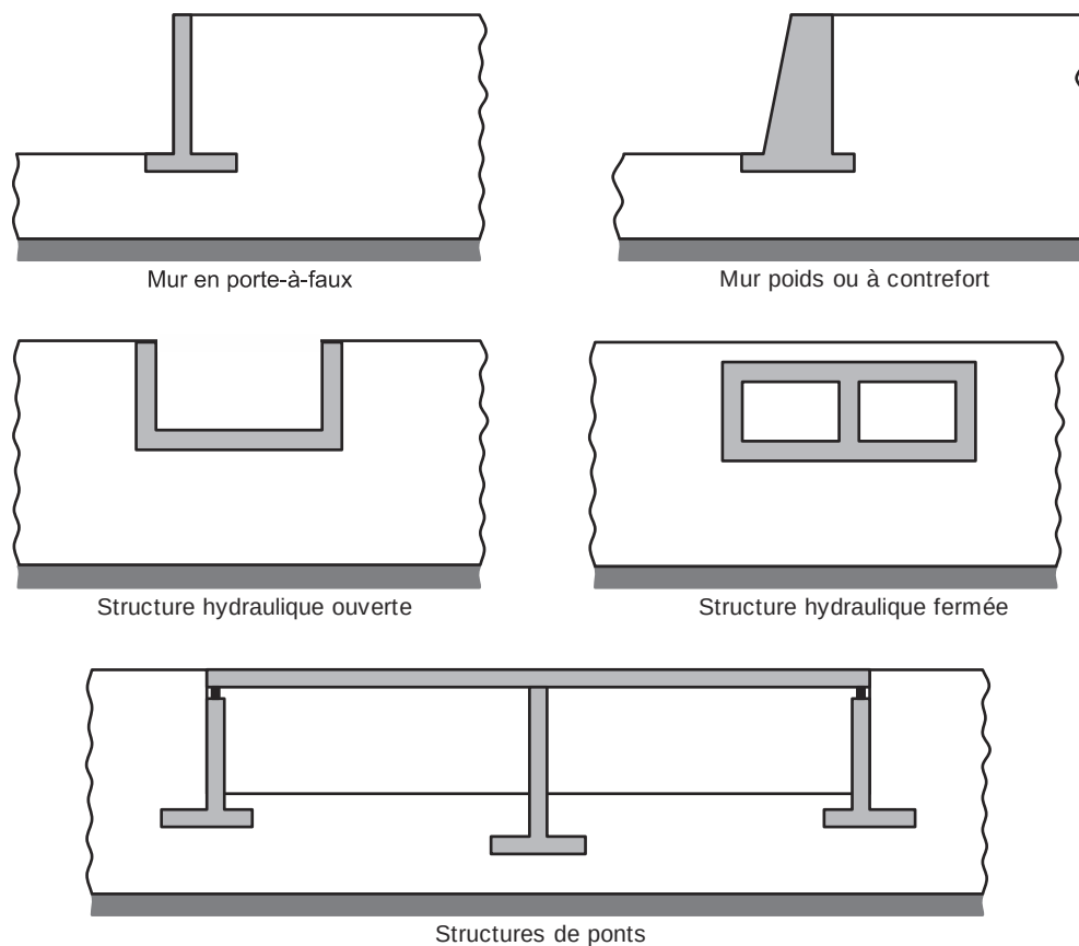
Figure 2-13 : Les principaux ouvrages de soutènement (Massicotte, 2019)
