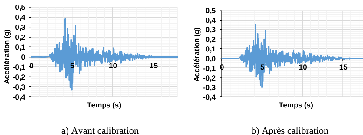
Figure 3-34 : Modification de l'accélérogramme du séisme MC7 suite à la calibration
