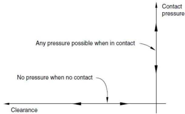
Figure 2-30 : Relation pression-distance normale de contact utilisée par défaut dans ABAQUS (Simulia, 2011)
