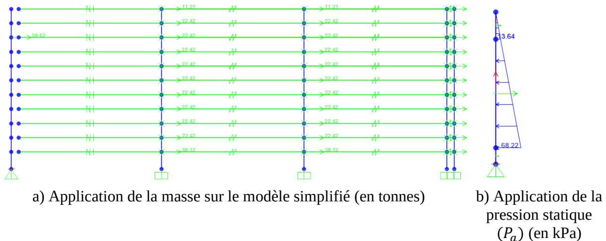
Figure 4-5 : Modèle de pont simplifié dans la direction longitudinale
