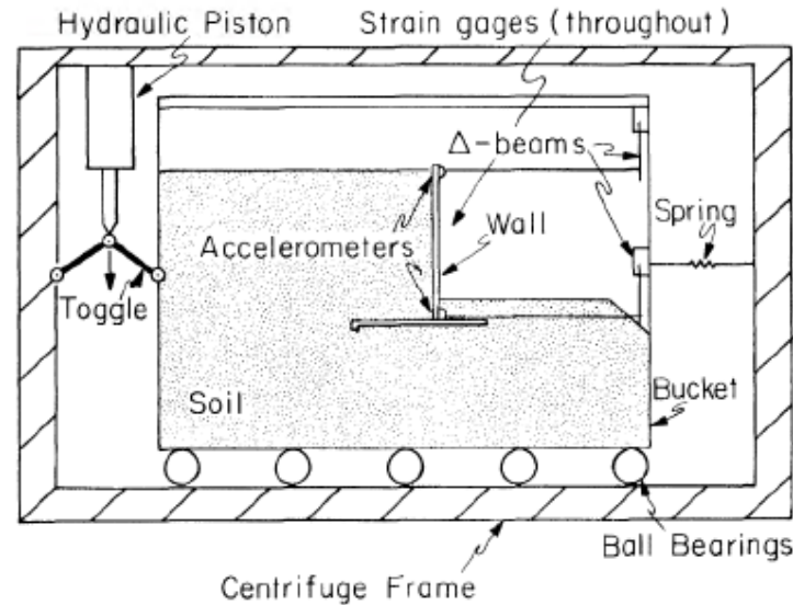
Figure 2-7 : Configuration expérimentale de Ortiz (1983) (Geraili et Sitar, 2013).
