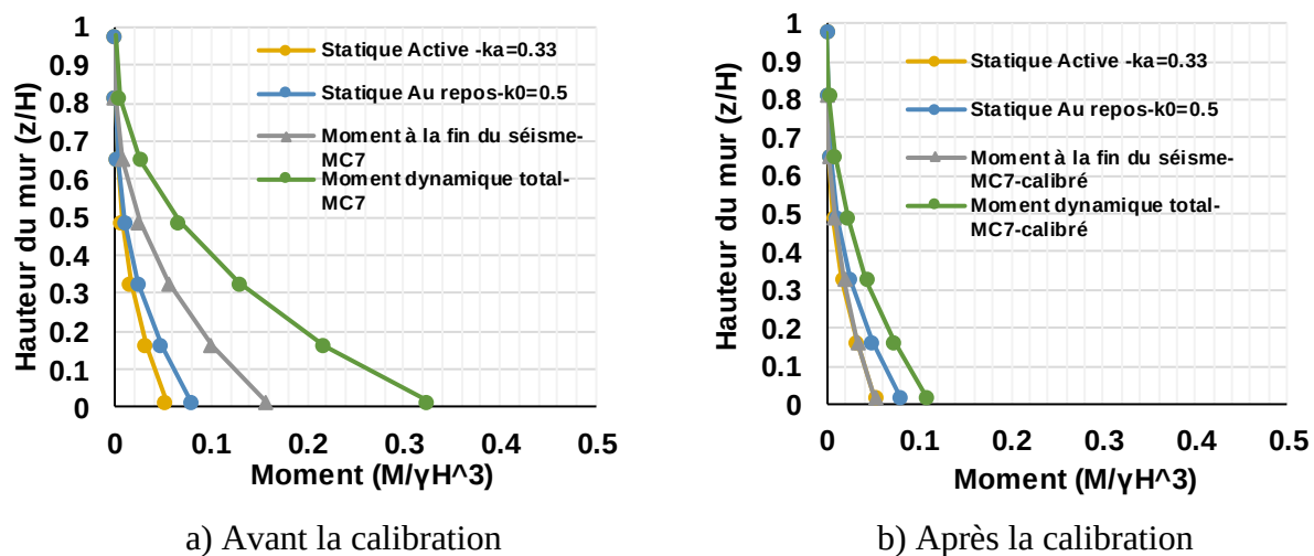
Figure 3-38 : Distribution du moment selon la hauteur du mur pour le séisme MC7
