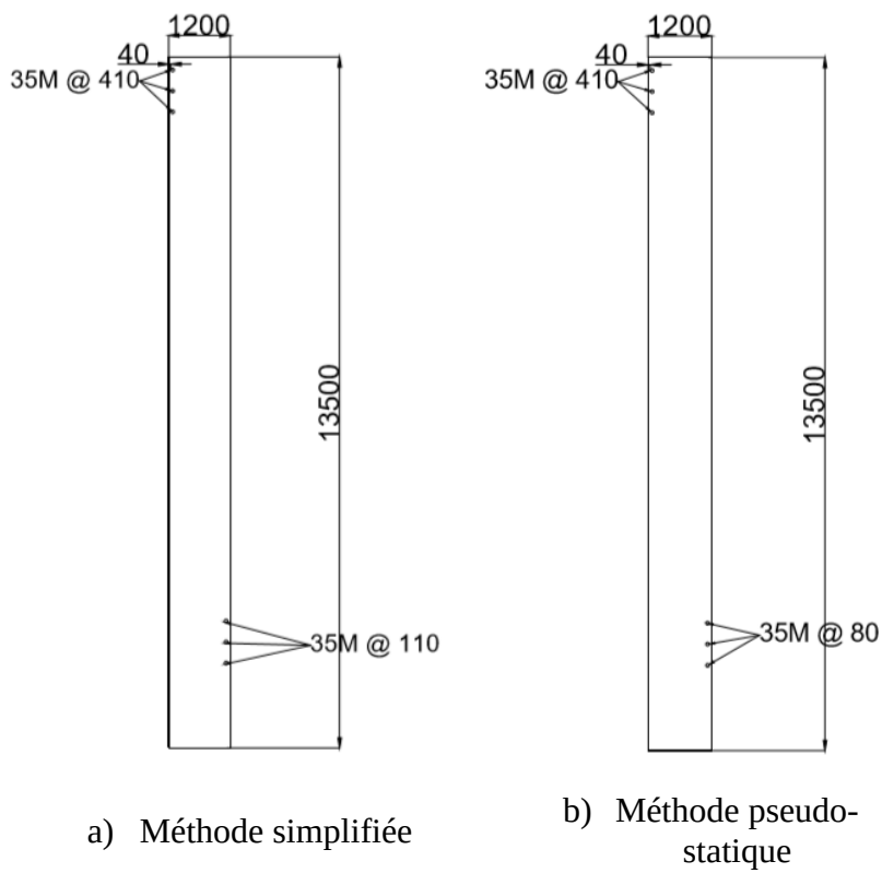
Figure 5-5 : Plan des sections ductiles pour la région de Charlevoix
