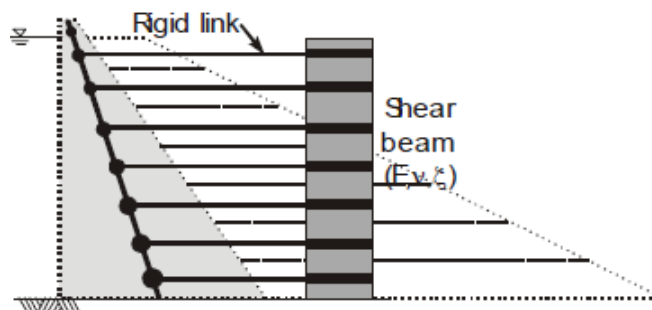
Figure 2-24 : Modèle de poutre en cisaillement et de connecteurs rigides. (Léger et Javanmardi, 2006)
