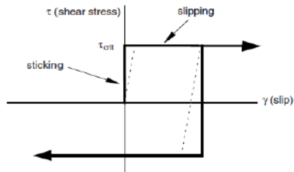
Figure 2-31 : Comportement de frottement (Simulia, 2011)
