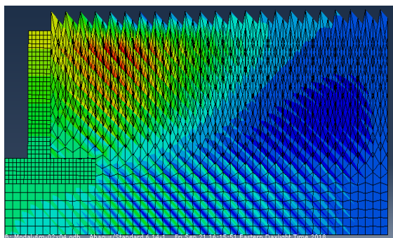
a) Mode 1 ( T=0.094 s) Facteur de participation 0.14%
