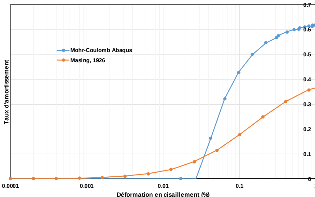
Figure 3-7 : Courbes du taux d'amortissement pour l'élément de sol.
