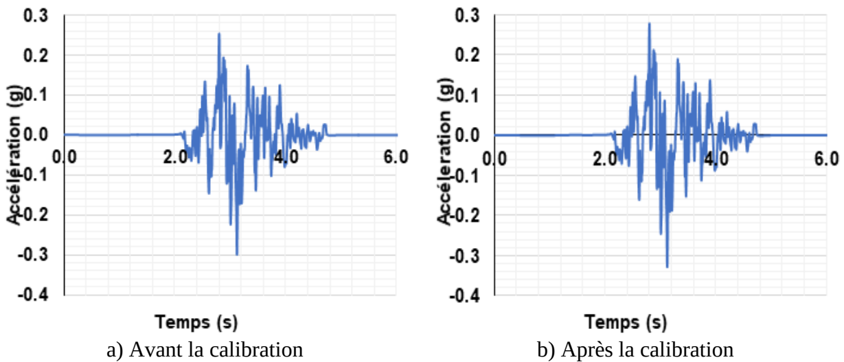
Figure 2-6 : Accélérogramme du séisme MC1
