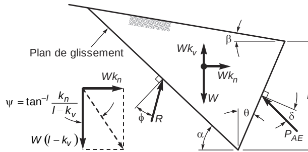
Figure 2-21 : Poussée active - Méthode de Mononobe-Okabe selon ASCE, 1994 (Massicotte, 2019)
