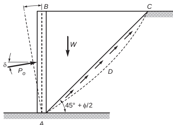
Figure 2-16 : État de poussée du sol ou poussée active (Massicotte, 2019)
