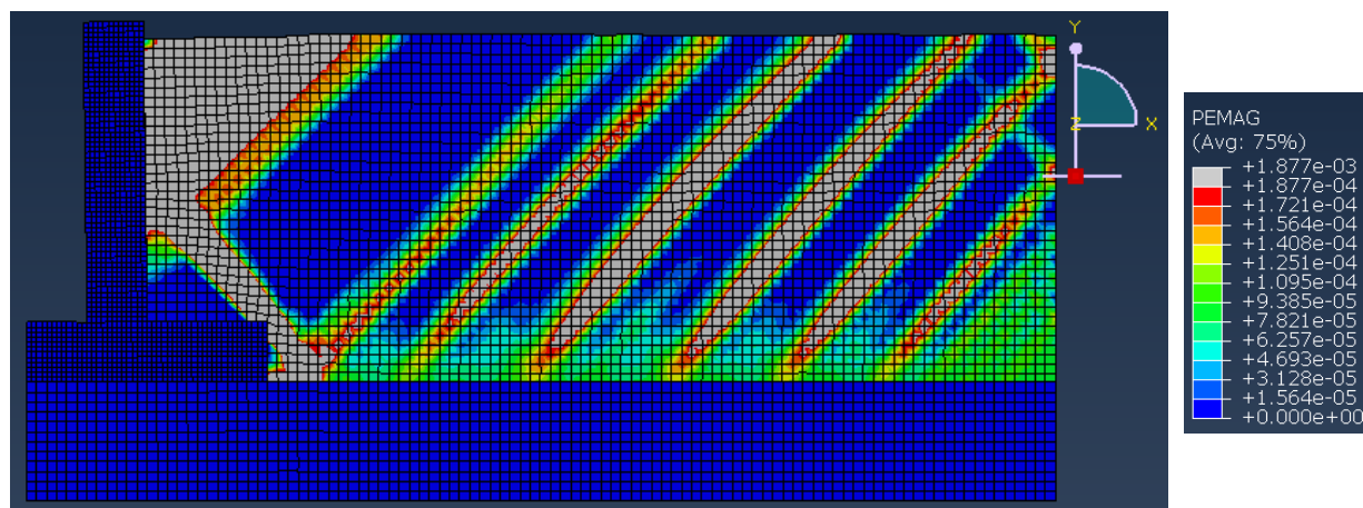
Figure 3-30 : Déformée de la structure avec superposition des contours des déformations plastiques (PEMAG) sous l'application du poids propre de la structure. Facteur d'échelle 100
