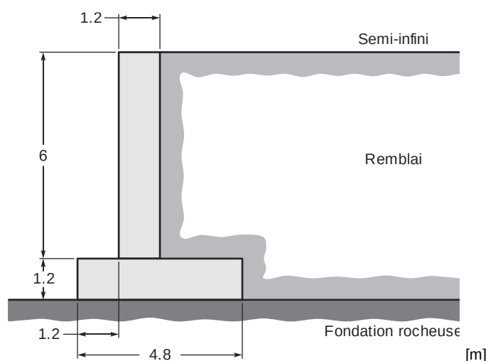
Figure 3-18 : Géométrie du système à l'étude
