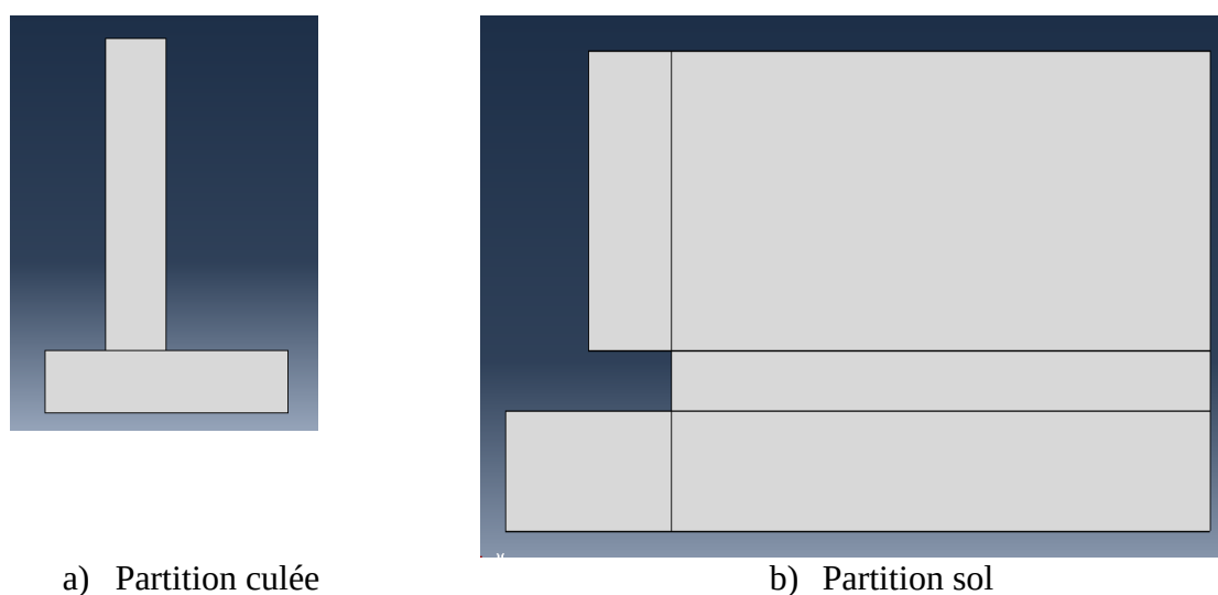
Figure 3-21: Les deux partitions créées dans ABAQUS
