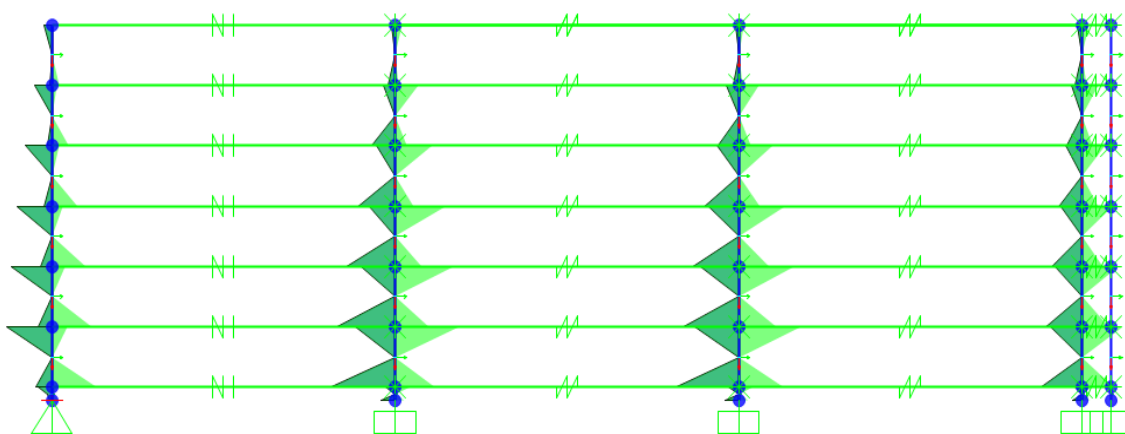
Figure 3-55 : Diagramme du moment de flexion pour le modèle simplifié sans contrainte en translation longitudinale à l'interface.
