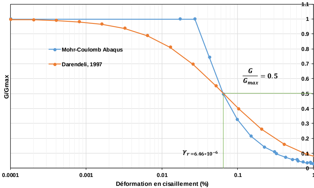
Figure 3-6 : Courbes normalisées de réduction du module sécant G
