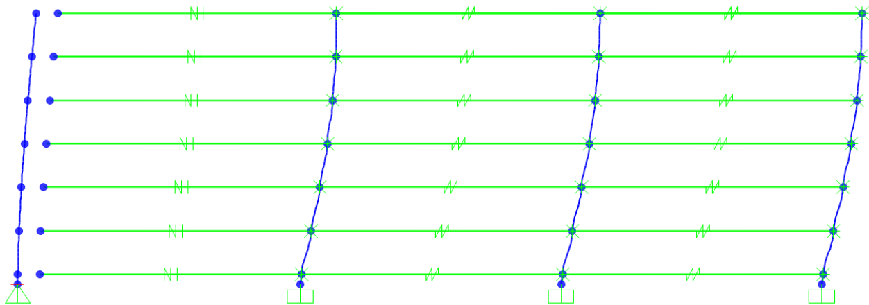
a) Mode fondamental-Sans frontière - T=0.135 s
