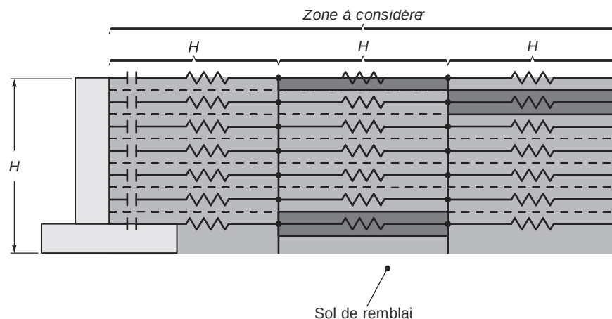
Figure 3-52 : Distinction des aires tributaires nécessaires au calcul de la rigidité axiale des ressorts
