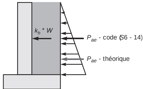
Figure 3-45 : Représentation des charges dynamiques dues au sol de remblai selon la norme CSA/CAN-S6-14
