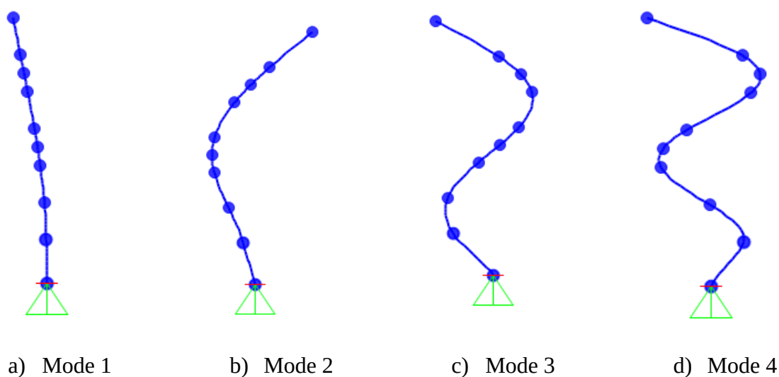
Figure 3-48 : Principaux modes de la structure
