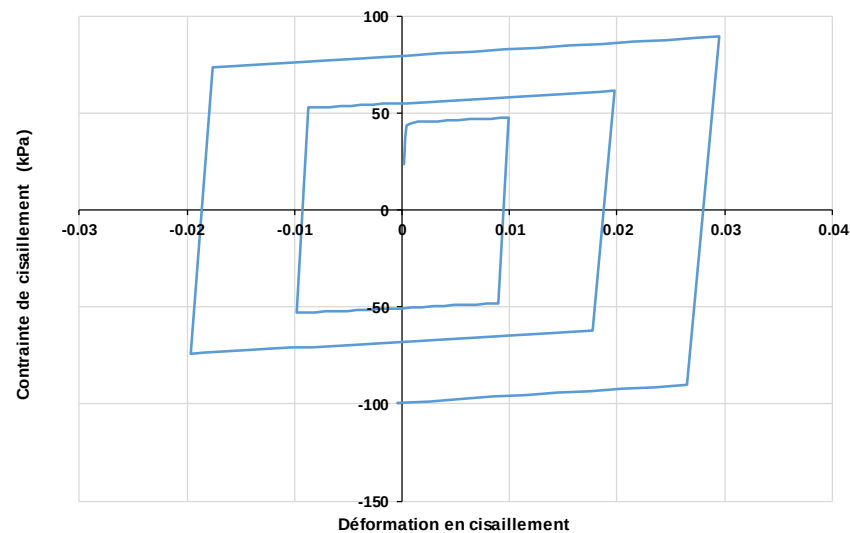
Figure 3-5 : Représentation de la boucle d'hystérésis pour la loi de Mohr-Coulomb dans ABAQUS
