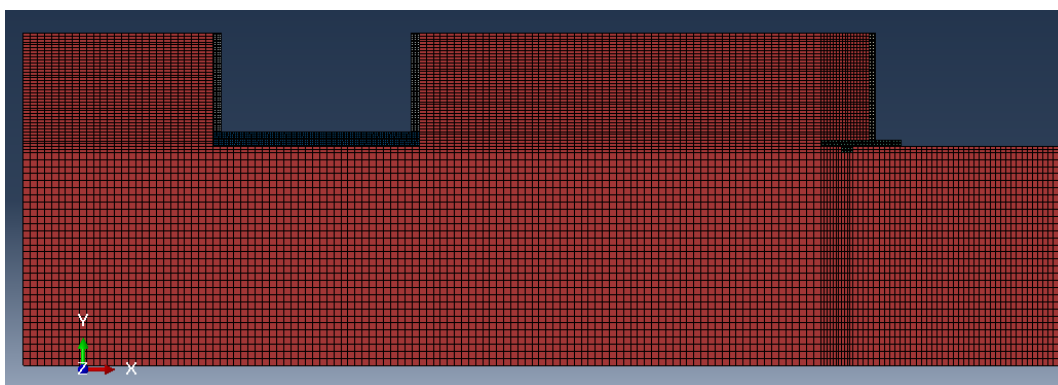
Figure 3-9 : Modèle ROOZ02 sur ABAQUS maillé
