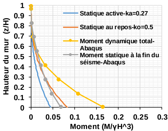
a) Kobe-TAK090-1-ABAQUS
