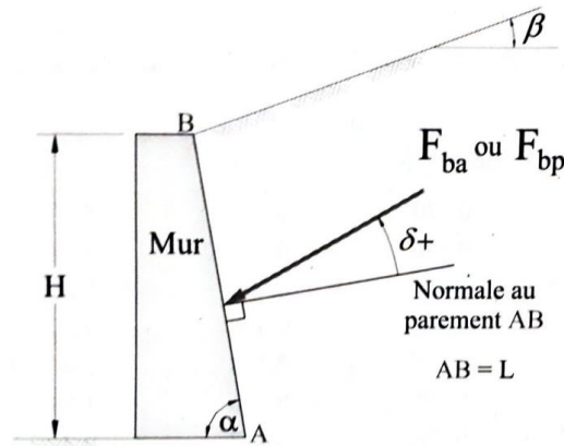
Figure 2-20 : Convention de signe pour \delta (Silvestri, 2011)
