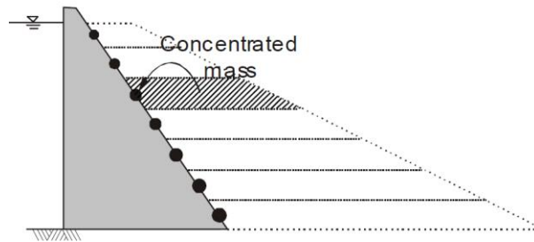
Figure 2-23 : Modèle simplifié avec des masses concentrées sur l'interface (Léger et Javanmardi, 2006)
