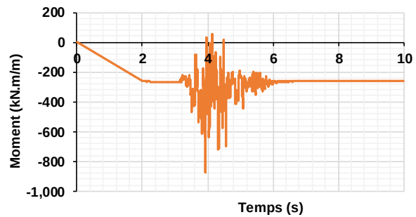
b) Moment de flexion
