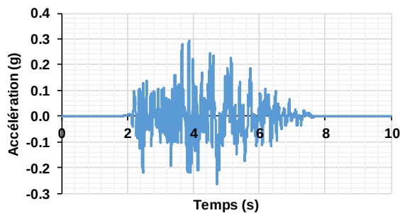
a) Accélérogramme
