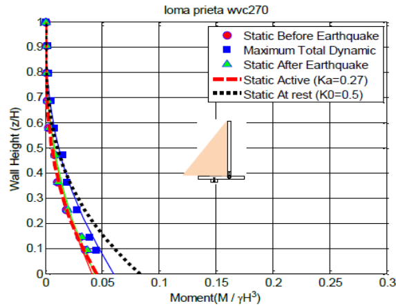
c) Centrifugeuse (Geraili et Sitar, 2013)
