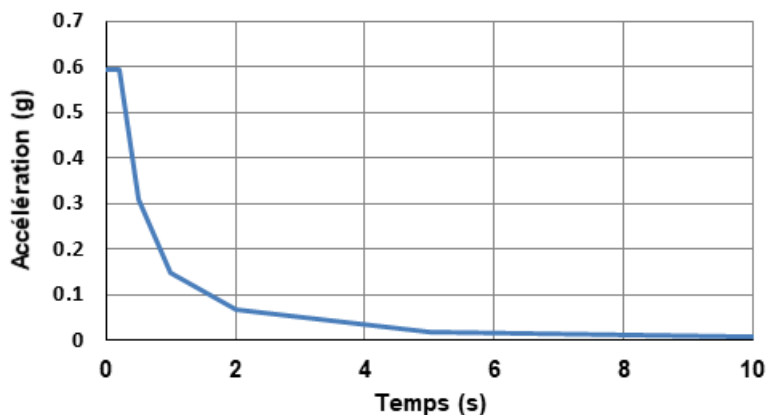
Figure 3-49 : Spectre de conception région de Montréal pour une période de retour de 2475 ans.
