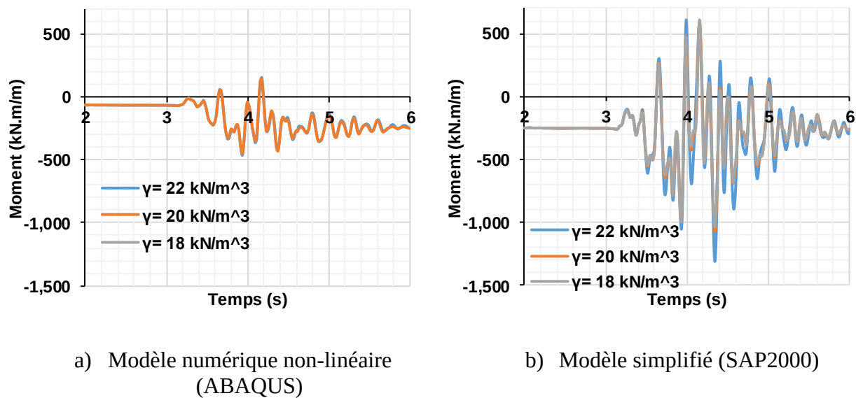
Figure 4-14 : Variation du moment à la base de la culée de 6 m pour le séisme MC1 en fonction du poids volumique \gamma .
