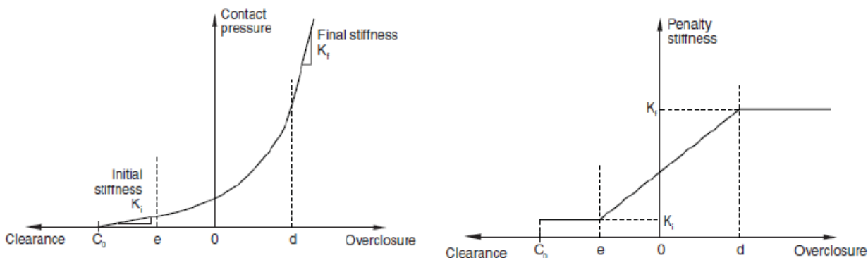
Figure 2-28 : Relation non linéaire de pénalisation entre la pression et la distance normale de contact (Simulia, 2011).
