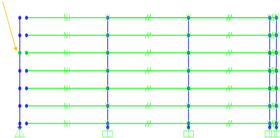
Figure 3-56 : Modèle simplifié du mur et du sol avec contrainte en translation longitudinale à l'interface.
