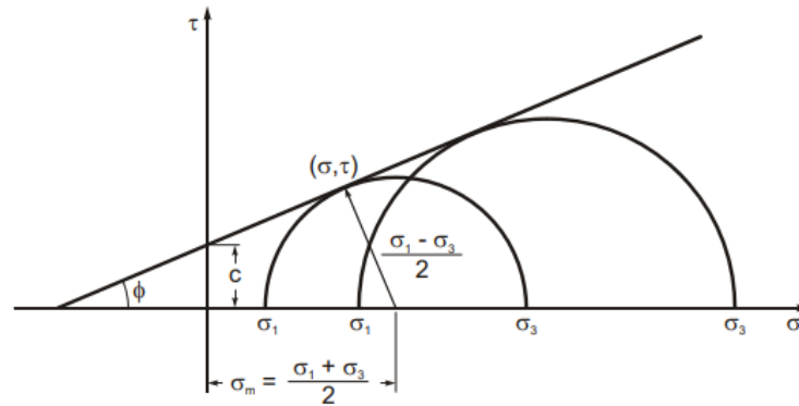
Figure 2-32: Ligne de rupture de Mohr-Coulomb (Simulia, 2011)
