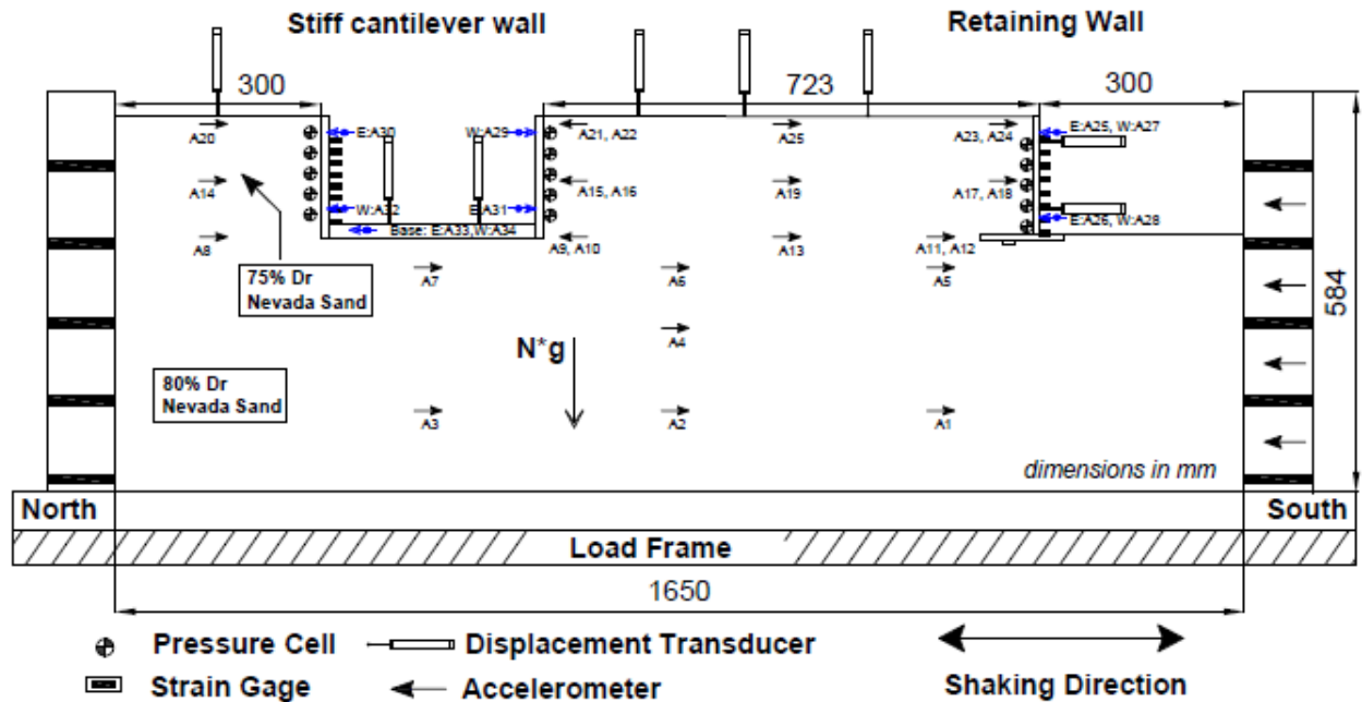
Figure 2-12 : Configuration du modèle ROOZ02, vue de profil (Geraili et Sitar, 2013).
