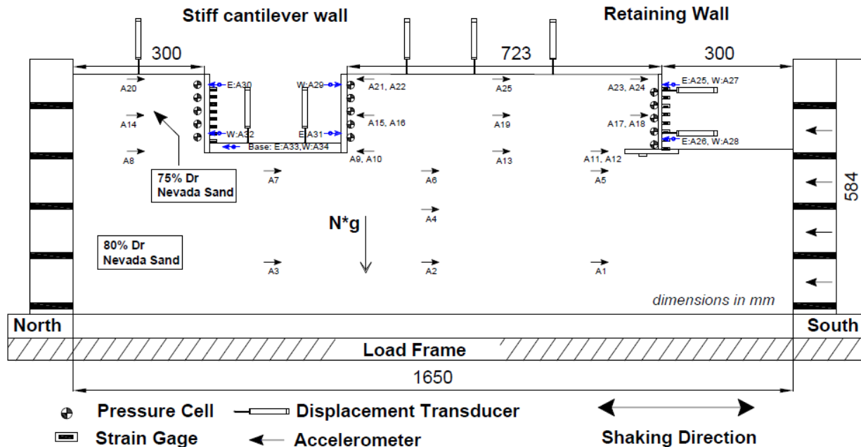
Figure 3-1: Configuration du modèle ROOZ02 vue de profil (Geraili et Sitar, 2013) (dimensions en mm).
