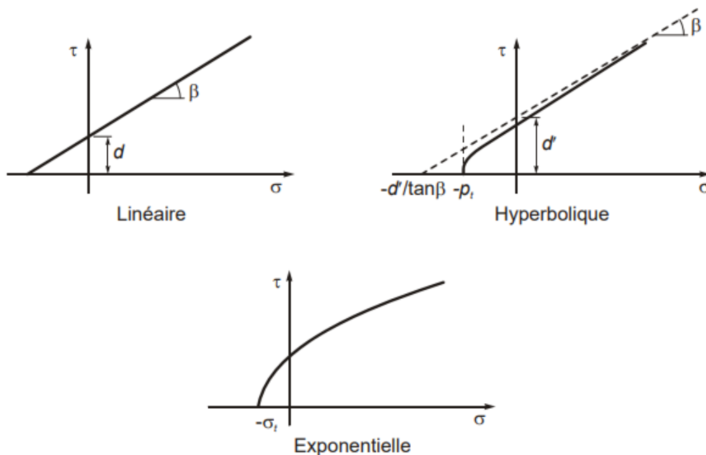
Figure 2-33 : Les choix de ligne de rupture de la loi "Extended Drucker-Prager" (Helwany, 2007)
