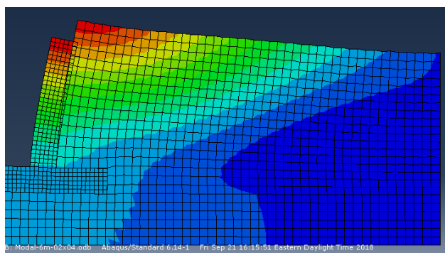
c) Mode 3 ( T=0.088 s) Facteur de participation 59.76%
