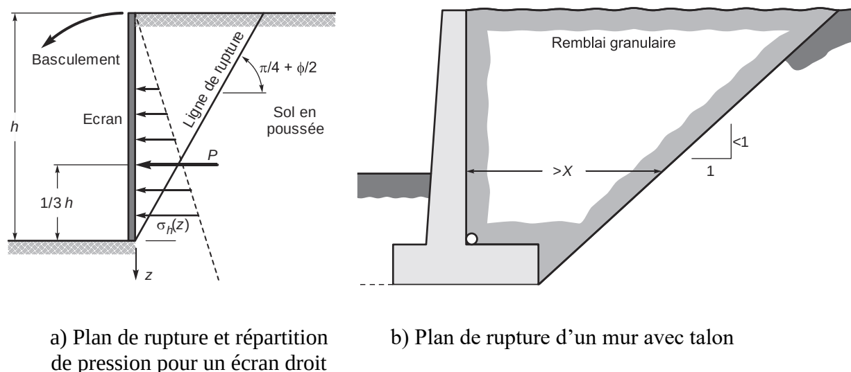
Figure 3-28 : Différents plans de rupture selon la théorie de Rankine
