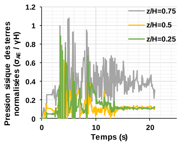
c) ABAQUS
