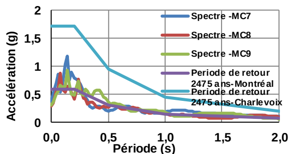
c) Spectre des séismes de MC7 à MC9
