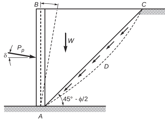
Figure 2-18 : État de butée dans le sol ou poussée passive (Massicotte, 2019)
