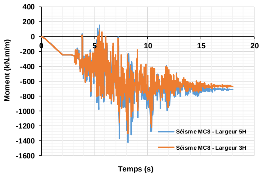
Figure 3-35 : Évolution dans le temps du moment à la base d'un mur de 6m pour différentes largeurs de remblai.
