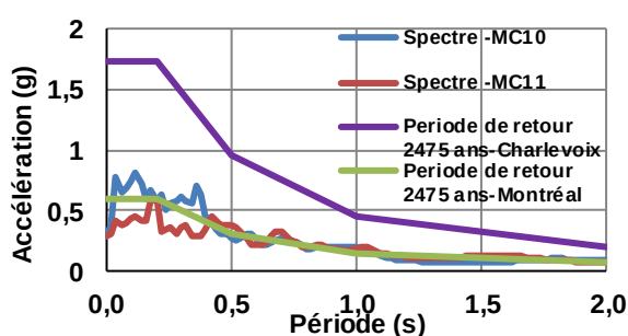
d) Spectre des séismes de MC10 et MC11
