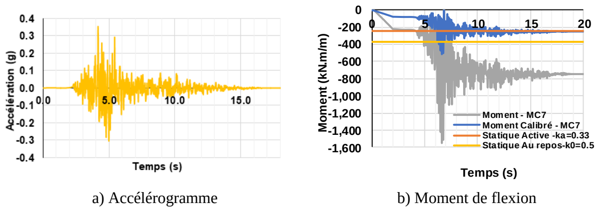
Figure 3-40 : Évolution dans le temps du moment après la calibration pour le séisme MC7
