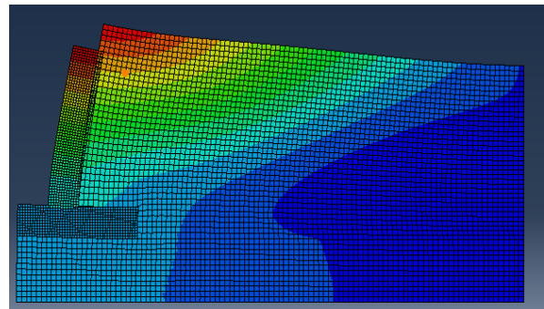
b) Mode 2 ( T=0.088 s) Facteur de participation 61.3%
