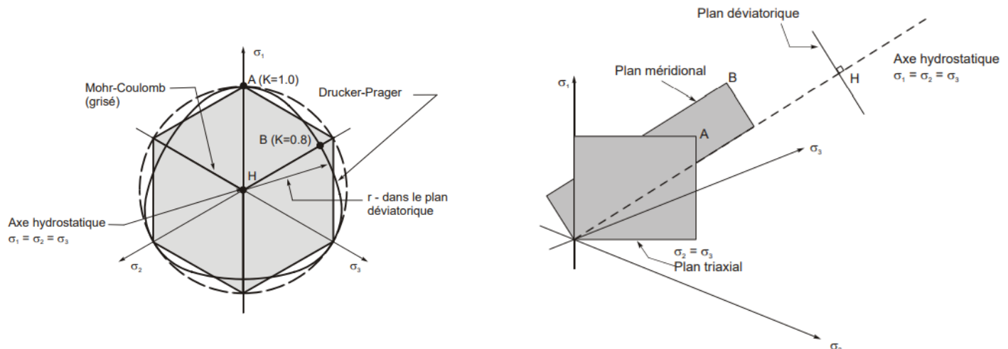
Figure 2-34 : Axe dans le repère triaxial selon Simulia, 2011 (Massicotte, 2019)
