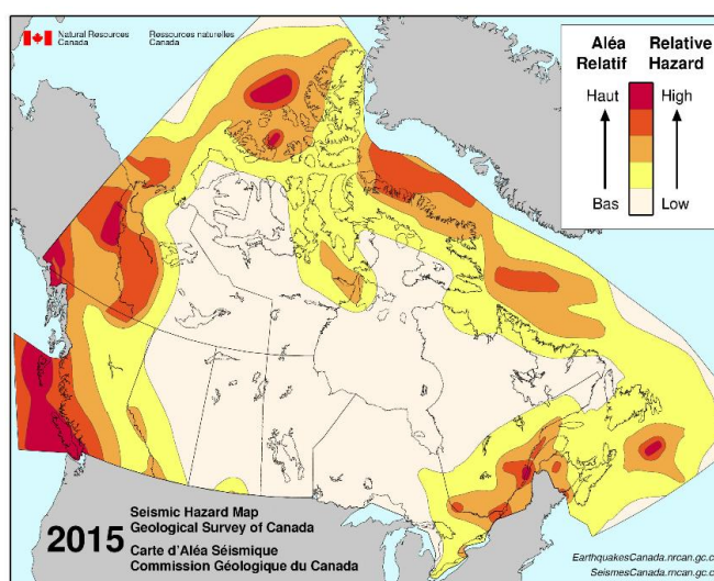
Figure 2-1 : Zones et aléa sismique du Canada (Commission géologique du Canada, 2015)
