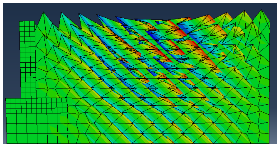
b) Mode 2 ( T=0.107 s) Facteur de participation 2.86%
