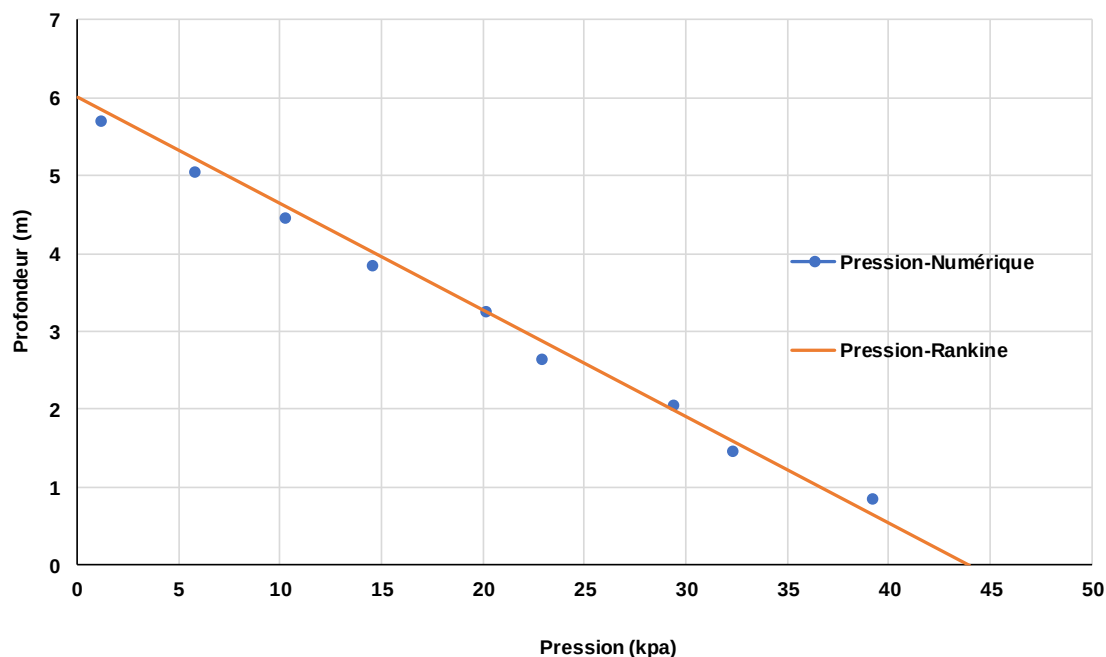
Figure 3-29 : Distribution de la pression statique à l'interface mur-sol
