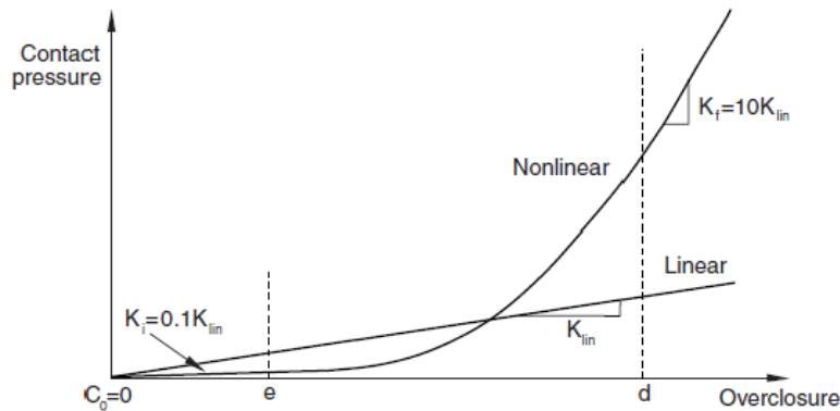
Figure 2-27 : Comparaison entre le comportement linéaire et non linéaire de la relation pression-distance normale de contact (Simulia, 2011)
