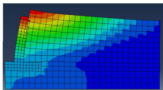
b) Mode 4 ( T=0.089 s) Facteur de participation 43.47%
