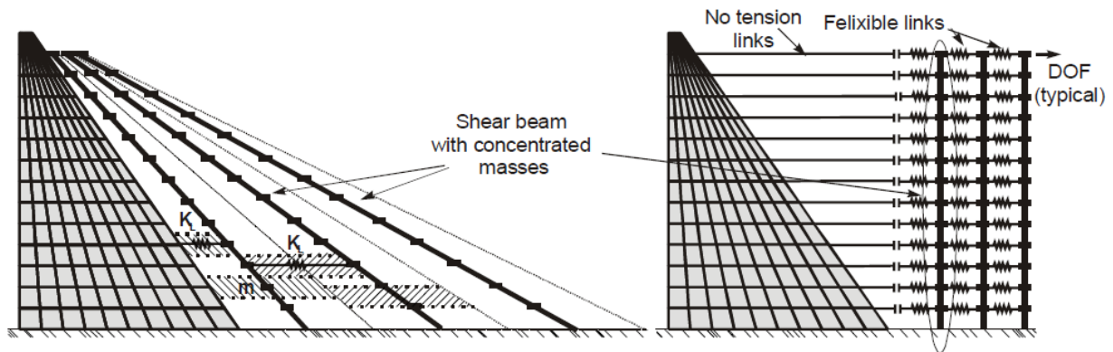
Figure 2-26 : Amélioration de la méthode simplifiée pour le cas d'un barrage (Léger et Javanmardi, 2006)
