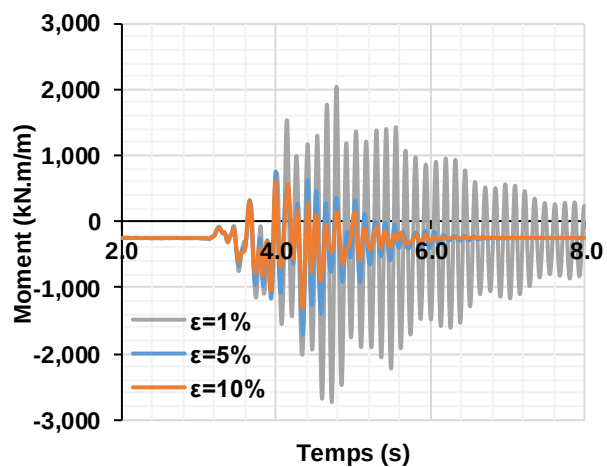
b) Modèle simplifié (SAP2000)
