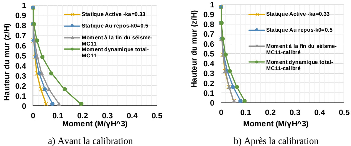
Figure 3-39 : Distribution du moment selon la hauteur du mur pour le séisme MC11
