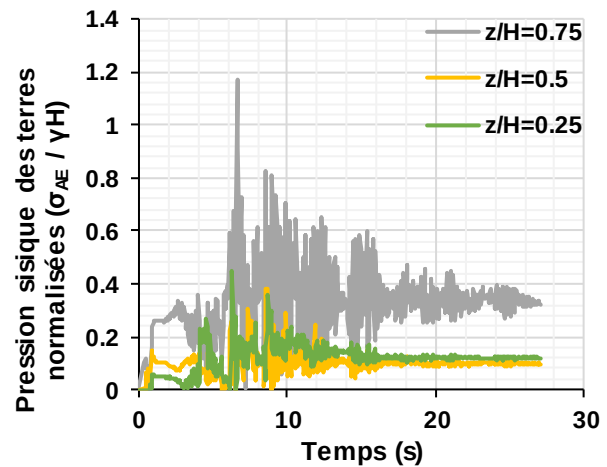
b) ABAQUS
