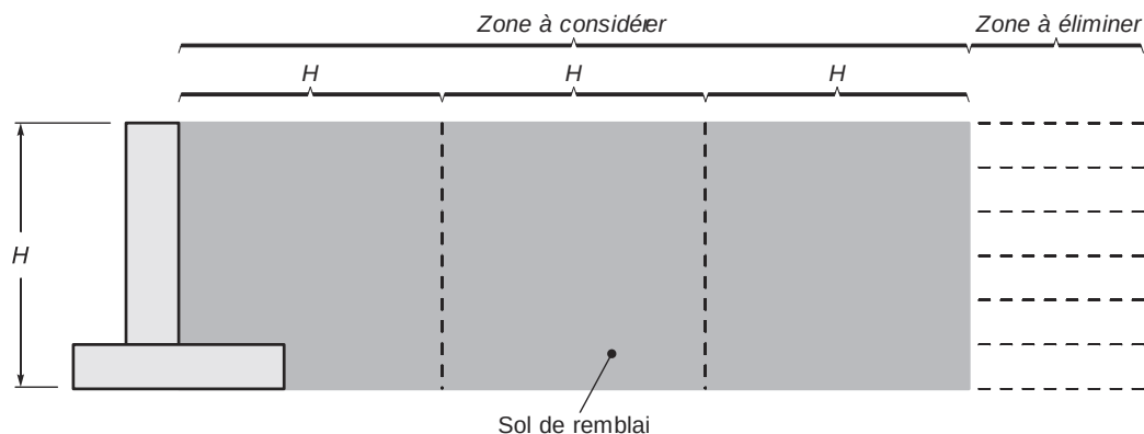
Figure 3-20 : Délimitation du volume de remblai compacté à considérer dans la modélisation.
