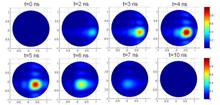
Fig. 9. Campo eléctrico normalizado radiado por la agrupación de antenas de la Fig. 8 obtenido con la técnica propuesta. Un pulso Gaussiano con modulación chirp es utilizado como excitación.
