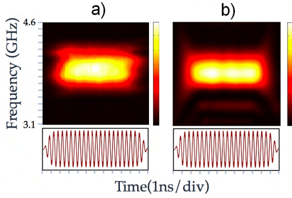
Fig. 7. Espectrogramas obtenidos de forma experimental (a) y con el método propuesto (b) cuando la CRLH LWA es alimentada por un pulso modulado rectangular.
