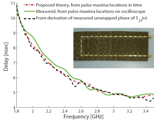
Fig. 2. Retardo de grupo obtenido con el método propuesto midiendo la diferencia temporal entre el máximo del pulso Gaussiano a la entrada y a la salida de la línea CRLH, en función de la frecuencia de modulación. Resultados experimentales, obtenidos tanto en el dominio temporal como frecuencial, son incluidos como validación.
