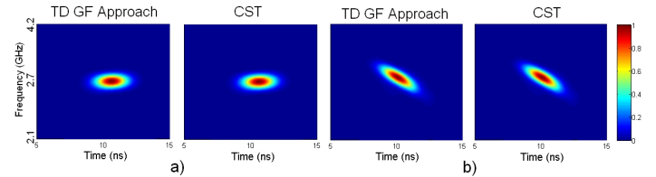
Fig. 6. Espectrogramas obtenidos con el método propuesto y con el software comercial CST® cuando la CRLH LWA es excitada por un pulso Gaussiano modulado por onda continua (a) y con una modulación chirp (b).
