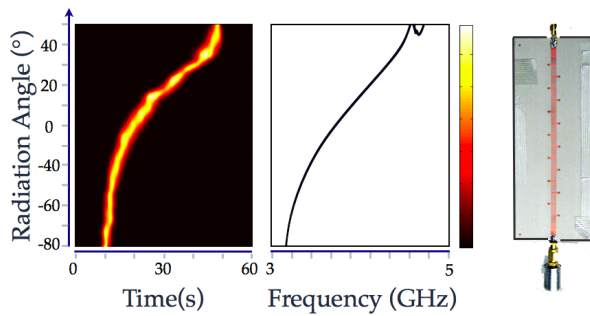
Fig. 4. Resultados experimentales obtenidos con 27 medidas en campo lejano separadas de forma uniforme ( 5^\circ ) en el plano de radiación de la antena. Respuesta ante una rampa frecuencial lineal (izquierda), y relación frecuencia-espacial de la ecuación 7 (derecha).
