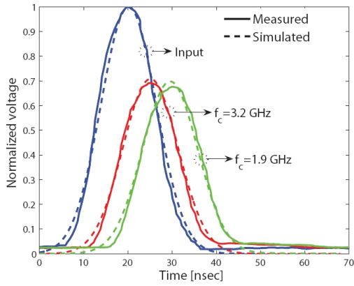
Fig. 3. Envolventes de un pulso Gaussiano usado para excitar una línea CRLH, a la entrada y salida de la misma, para dos frecuencias de modulación diferentes. Resultados experimentales son incluidos como validación.
