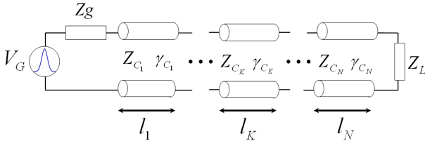
Fig. 1. Línea de transmisión general, compuesta por N -líneas de diferentes características, excitada por una fuente puntual.
