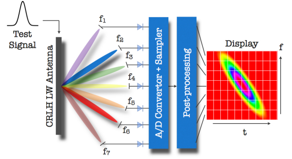
Fig. 5. Esquema del analizador de espectros en tiempo real propuesto. Los receptores se encargan de captar la señal en función del tiempo en distintas regiones del espacio, donde sólo estarán presentes frecuencias discretas.
