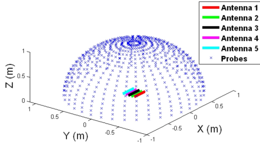
Fig. 8. Agrupación de 5 CRLH LWA empleadas para obtener un haz tipo ‘lápiz’ en cualquier posición del espacio. 1369 receptores son utilizados para analizar el campo radiado en el espacio.
