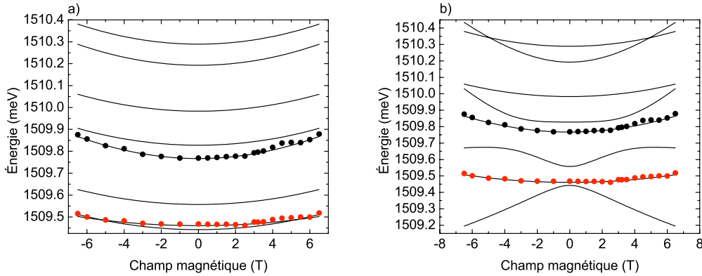
FIGURE 5.9 Photoluminescence en fonction du champ magnétique pour la dyade D_3 . Les points représentent les deux raies excitoniques mesurées, la couleur indique la polarisation. Les huit lignes représentent le calcul fait à partir des hamiltoniens 4.2 et 4.24 en faisant la régression sur les états à plus basse énergie (cas #2). Les paramètres utilisés sont en notation [g_e; K; L; g_h] a) [0.09; 0.72; -0.30; -0.05] b) [1.05; -0.48; 0.39; 0.4] .
