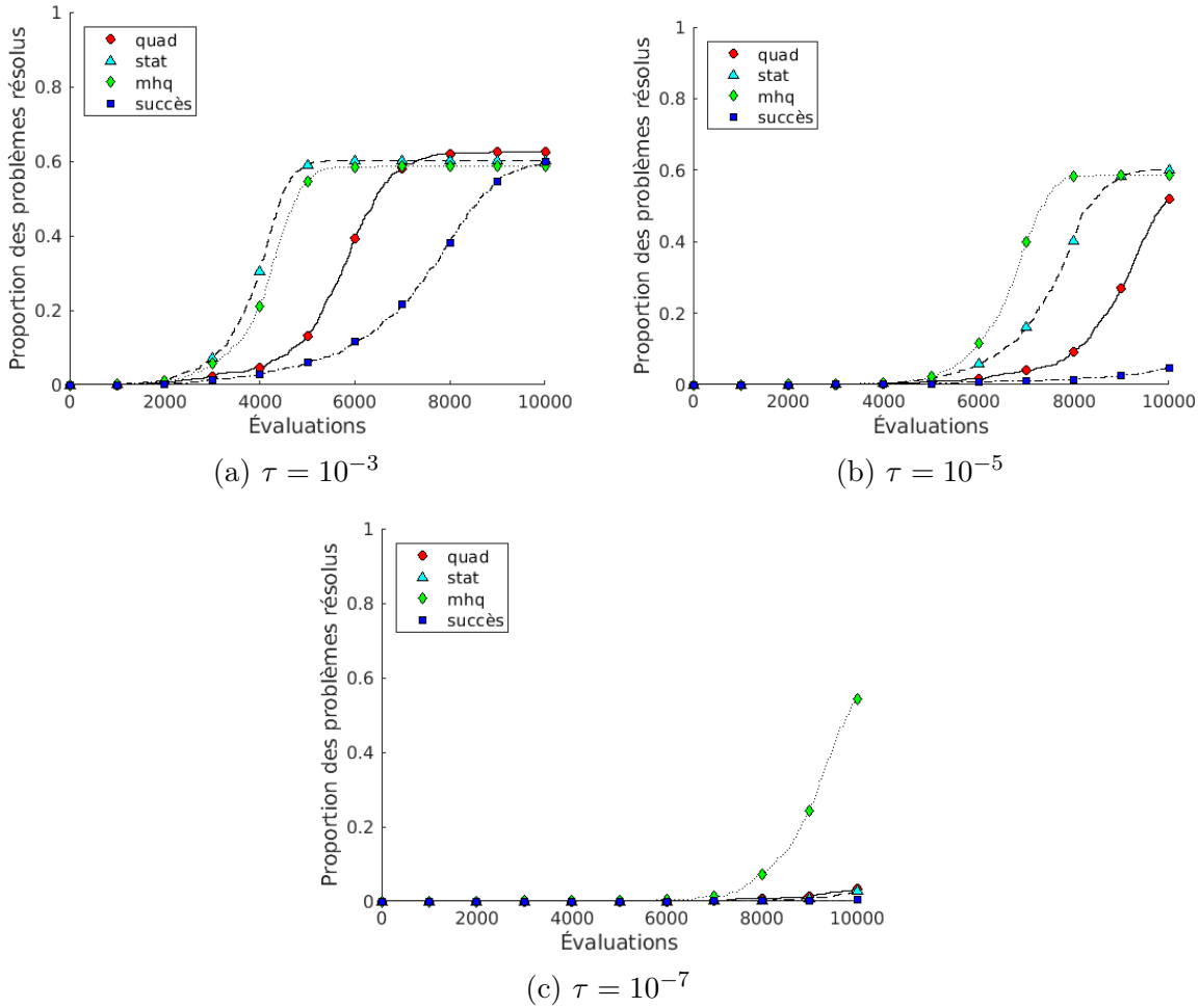
Figure 4.4 Profils de données obtenus avec une tolérance \tau sur 10 instances d'exécution de 100 problèmes numériques Simple_MDO_16_Variables.
