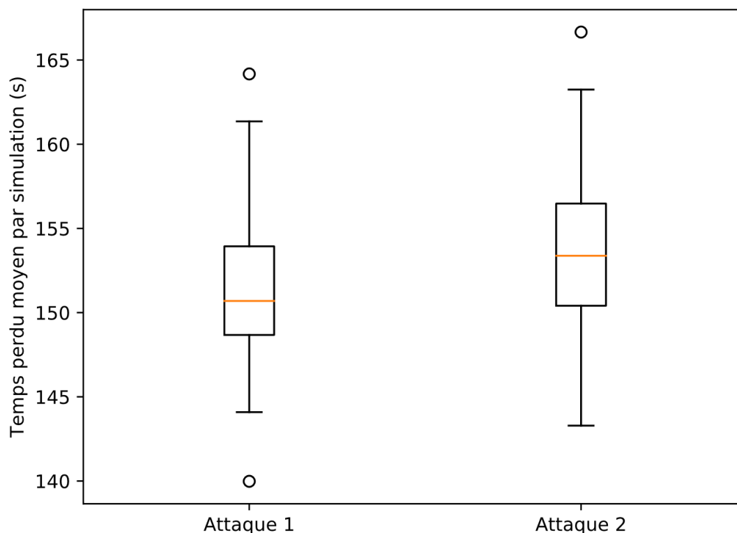
Figure 6.8 : Temps perdu moyen des attaques individuelles contre les feux de circulation
