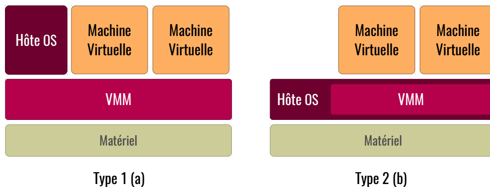
Figure 2.6 Types d'hyperviseurs
