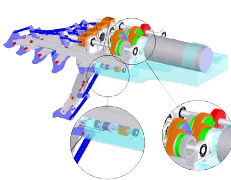
Figure 7-2 : Main anthropomorphe sous-actionnée par engrenage planétaire (Nasser, Rincon, & Rodriguez, 2006)
