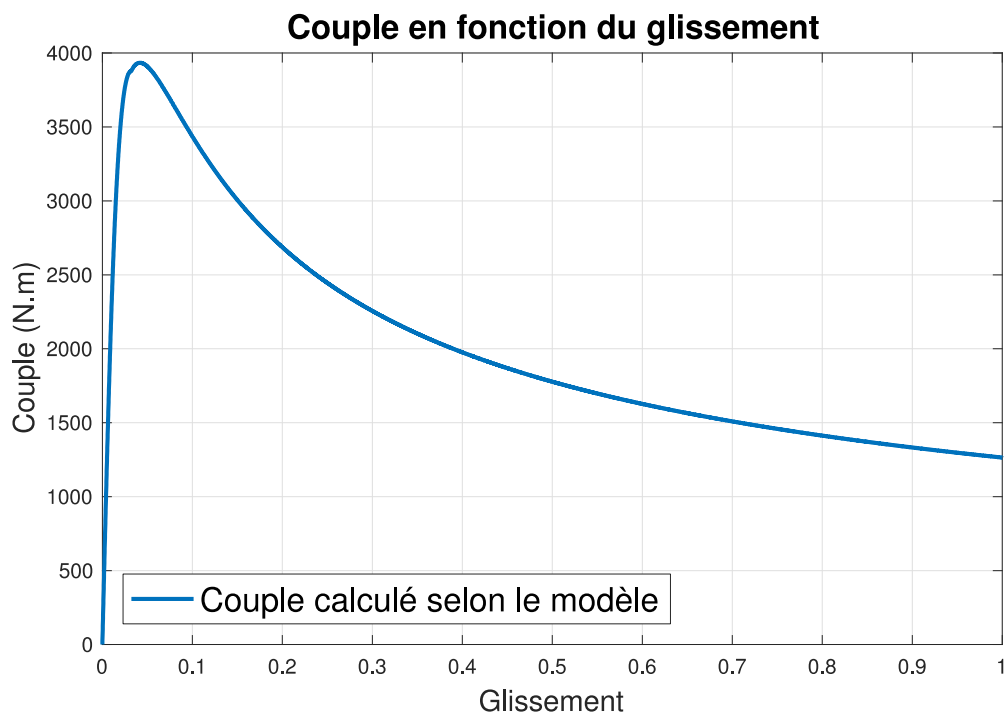
Figure 1.1 : Couple en fonction du glissement.
