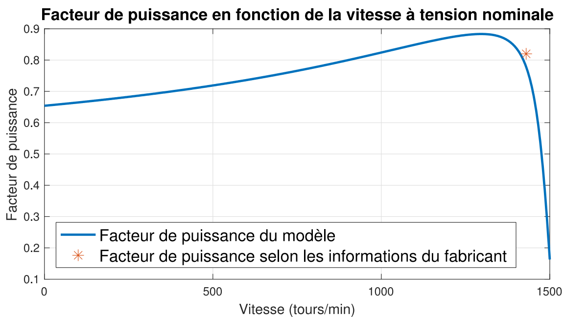
Figure 4.6 : Facteur de puissance en fonction de la vitesse.
