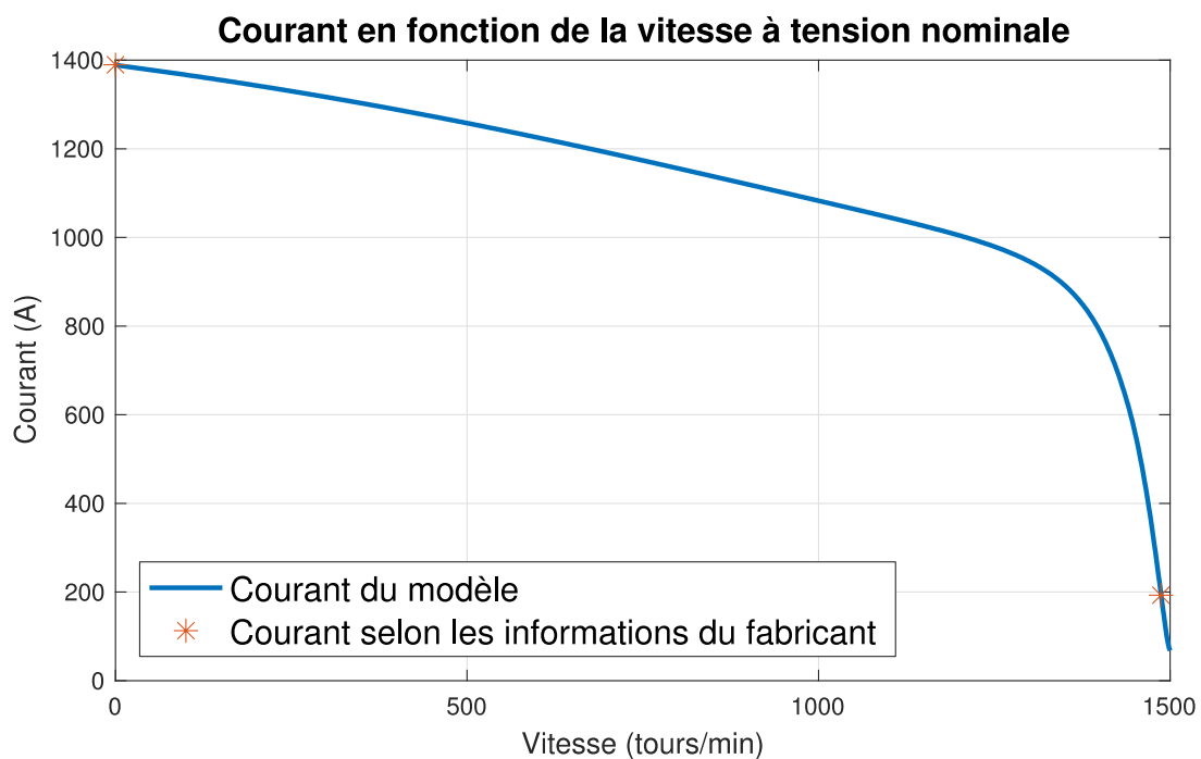
Figure 4.2 : Courant en fonction de la vitesse
