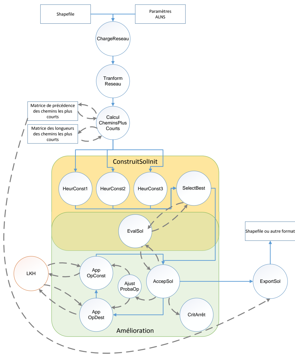
Figure 6.2 Représentation schématique du code de l'ALNS.
