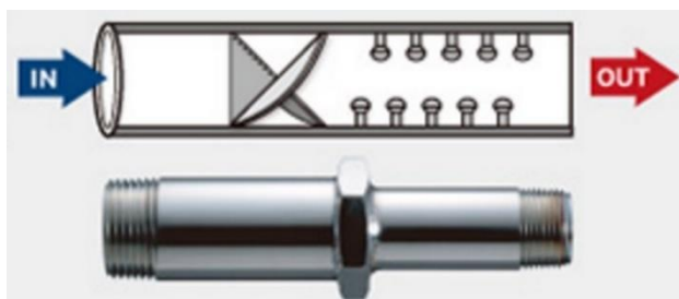
Figure 6.2 : Mélangeur statique OHR (tirée de http://www.ohr-labo.com/en/mixer1.html )
