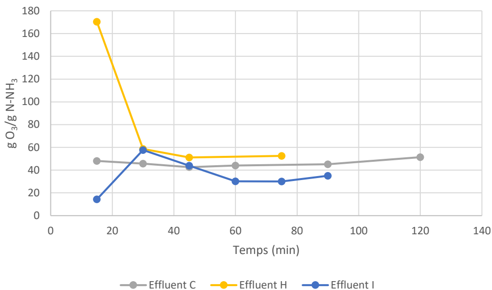
Figure 4.24 : Consommation d'O 3 en fonction du temps pour les essais réalisés avec les effluents C, H et I
