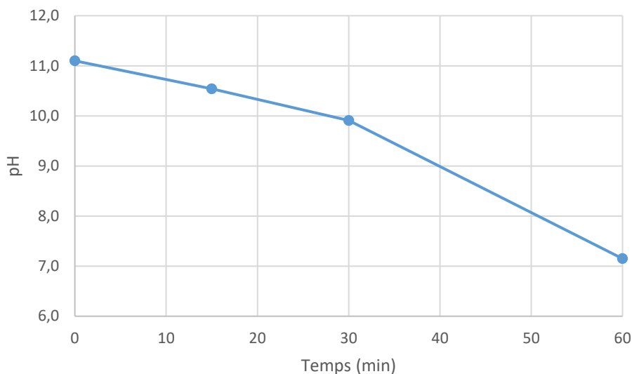
Figure 4.10 : pH en fonction du temps pour l'essai réalisé à pH 11 non maintenu
