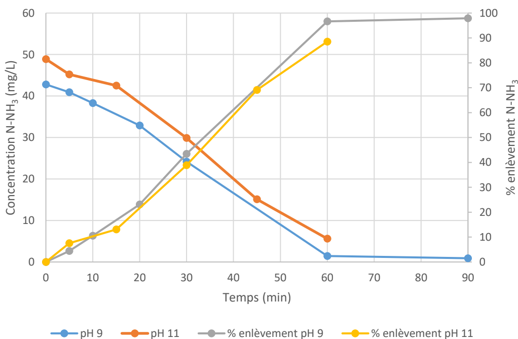
Figure 4.13 : Concentration et taux d'enlèvement de N-NH 3 en fonction du temps pour les essais réalisés avec le bromure à différents pH
