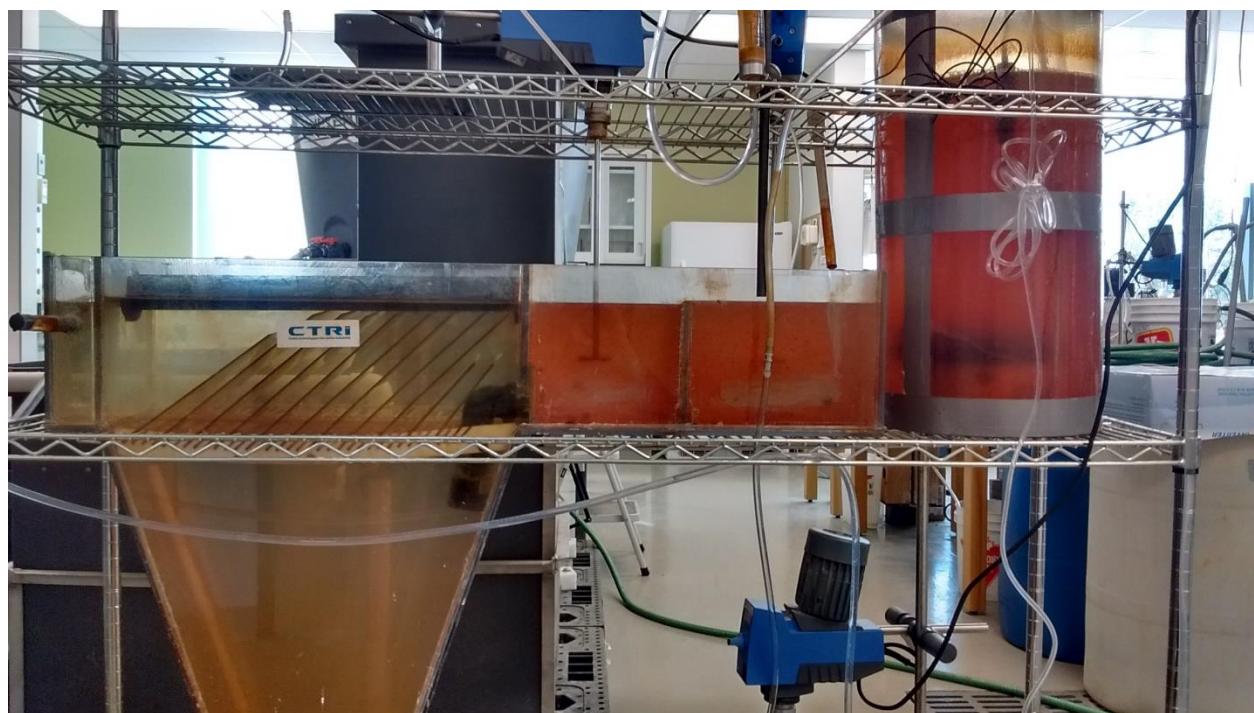
Figure 6.29 : Décanteur, réservoir de coagulation-floculation et colonne d'aération
