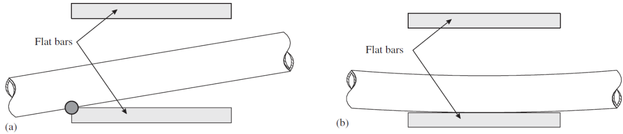
Figure 2-3 : Type de contact tube/support : (a) contact ponctuel; (b) contact segmentaire (M. Hassan & Rogers, 2005)
