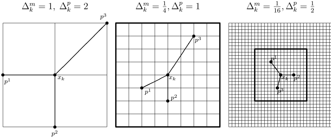
Figure 2.9 Exemples de cadres de MADS P_k = \{x_k + \Delta_k^m d : d \in D_k\} = \{p^1, p^2, p^3\} pour différentes valeurs de \Delta_k^m and \Delta_k^p . Dans les trois figures, le treillis M_k est l'intersection des lignes horizontales et verticales. On remarque que le nombre de points de sonde possibles augmente de façon exponentielle quand \Delta_k^m décroît.
