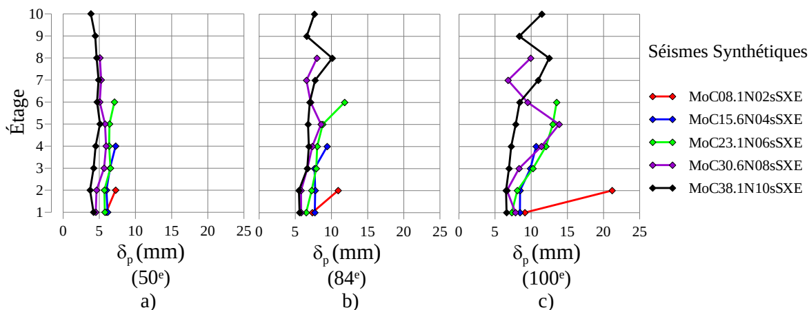
Figure 5.20 - Bâtiments standards à Montréal: Demande de déformation ( \delta_p (mm)) : a) Médiane (50°); b) 84 e fractile; c) Maximum (100°)
