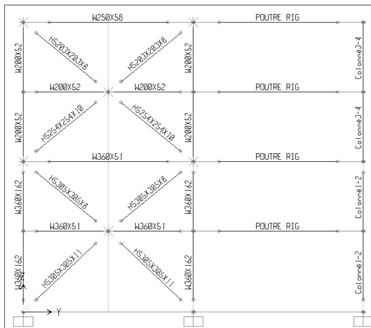
Figure 3.18 - Modèle 2D du cadre étudié dans SAP2000
