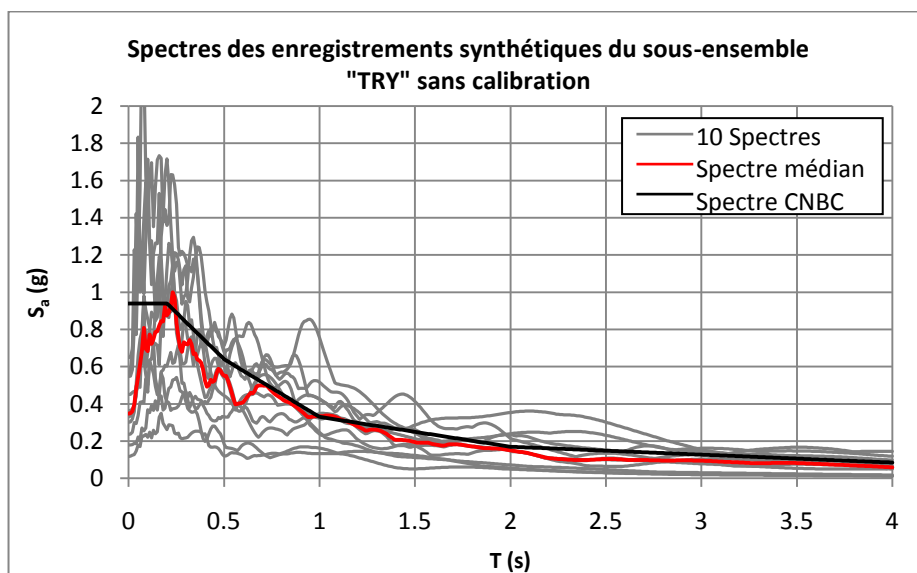
Figure 3.7 - Spectres des accélérographes sélectionnés du sous-ensemble TRY
