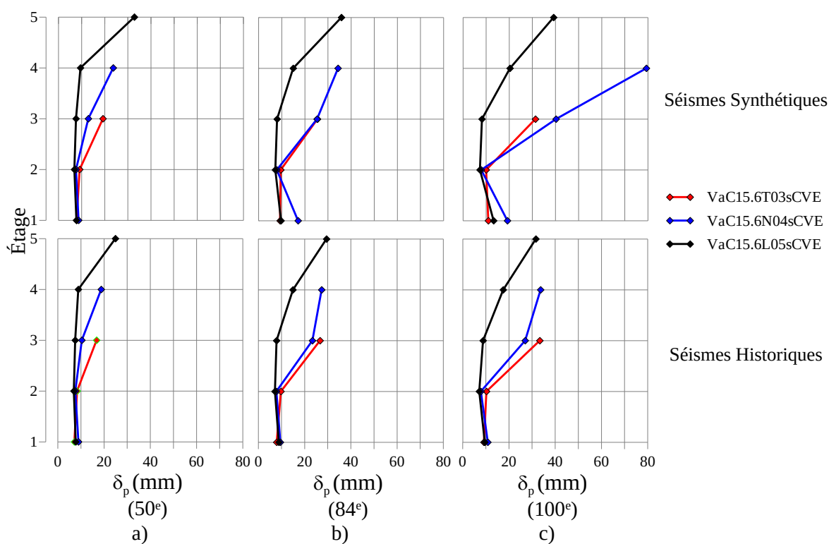
Figure 5.27 - Vancouver hauteur d'étages: Demande de déformation ( \delta_p (mm)): a) Médiane (50 e ); b) 84 e fractile; c) Maximum (100 e )
