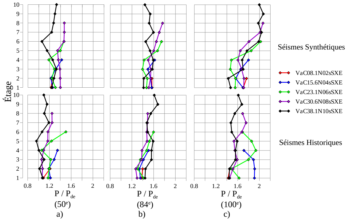
Figure 5.11 - Bâtiments standards à Vancouver: Ratio P/P_{de} : a) Médiane (50 e ); b) 84 e fractile; c) Maximum (100 e )
