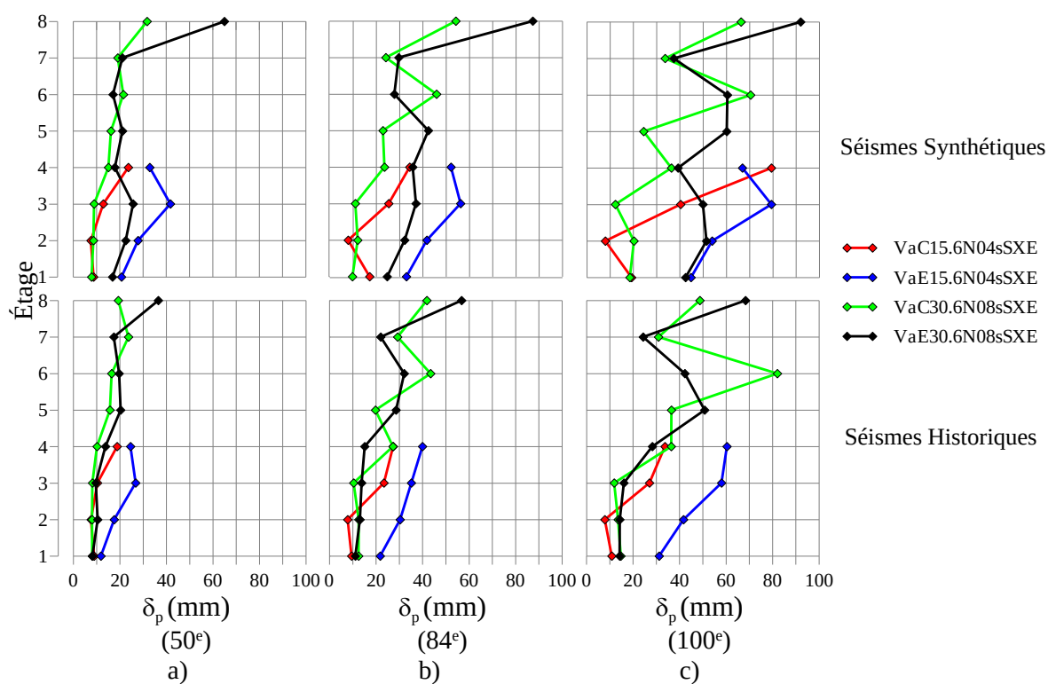
Figure 5.23 - Vancouver sites de catégorie C et E: Demande de déformation ( \delta_p (mm)): a) Médiane (50 e ); b) 84 e fractile; c) Maximum (100 e )
