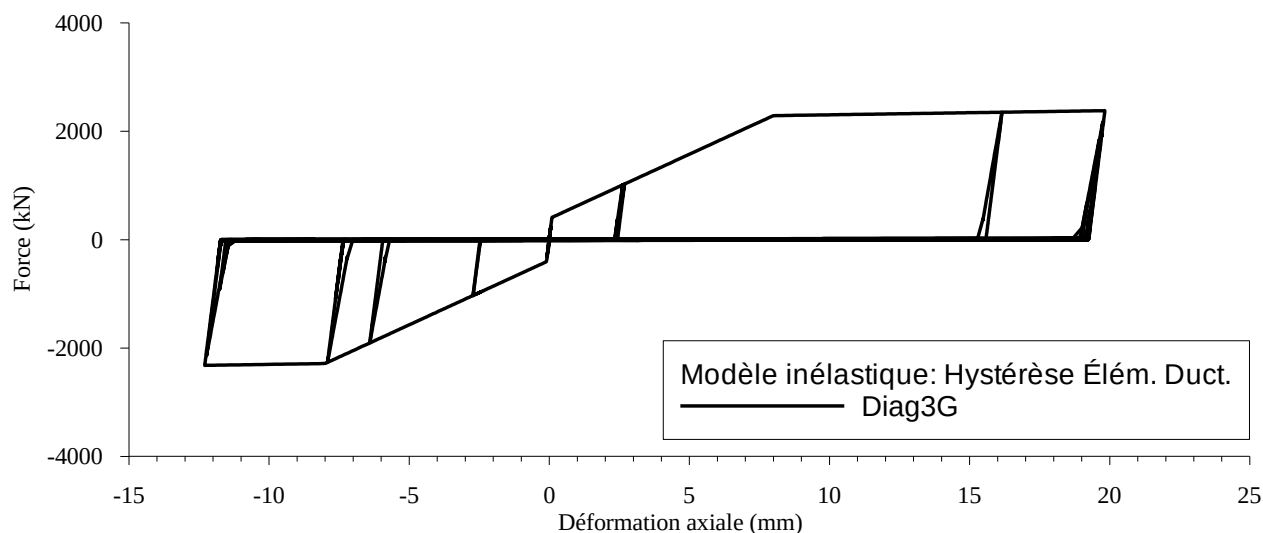
Figure 4.17 - Comportement axiale de la connexion : Analyses inélastiques
