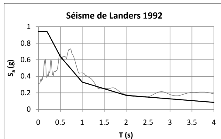
Figure 5.30 - Spectre du séisme de Landers 1992
