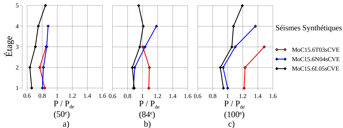
Figure 5.17 - Montréal hauteur d'étages: Ratio V_d/V_{de} : a) Médiane (50 e ); b) 84 e fractile; c) Maximum (100 e )
