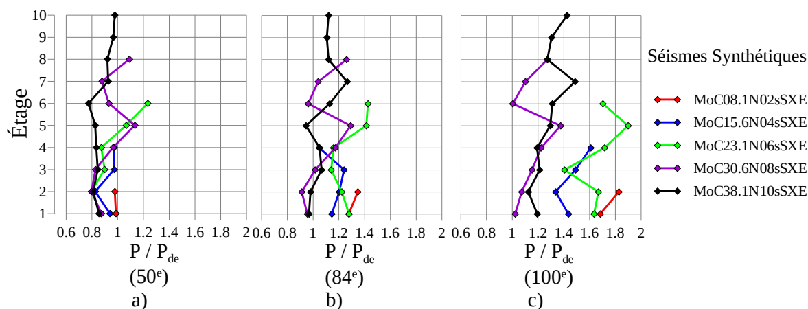
Figure 5.10 - Bâtiments standards à Montréal: Ratio P/P_{de} : a) Médiane (50 e ); b) 84 e fractile; c) Maximum (100 e )
