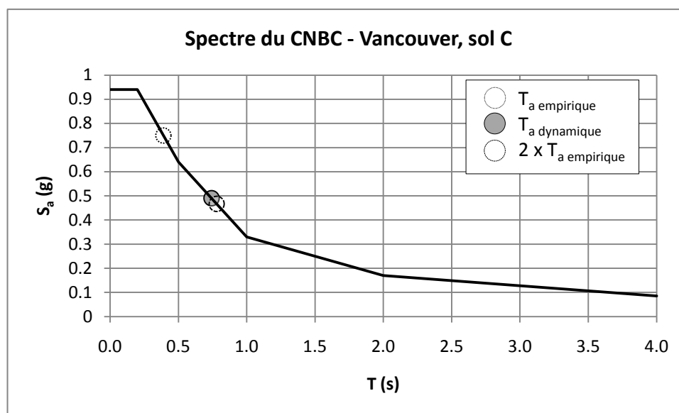
Figure 3.17 - Spectre de dimensionnement
