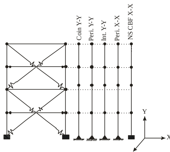
Figure 4.8 - Modèle OpenSees
