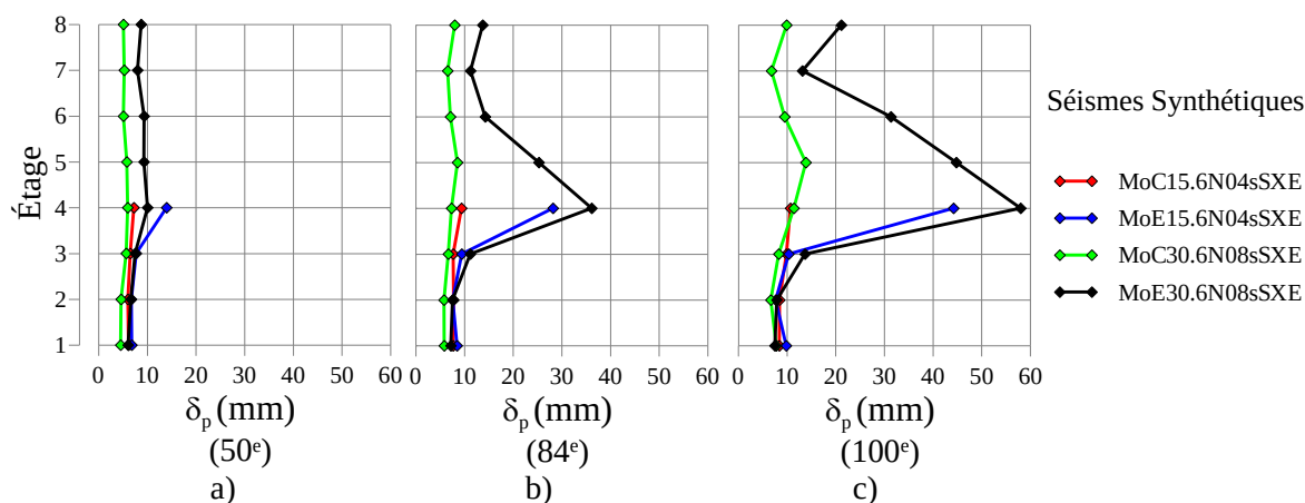
Figure 5.22 - Montréal sites de catégorie C et E: Demande de déformation ( \delta_p (mm)): a) Médiane (50 e ); b) 84 e fractile; c) Maximum (100 e )
