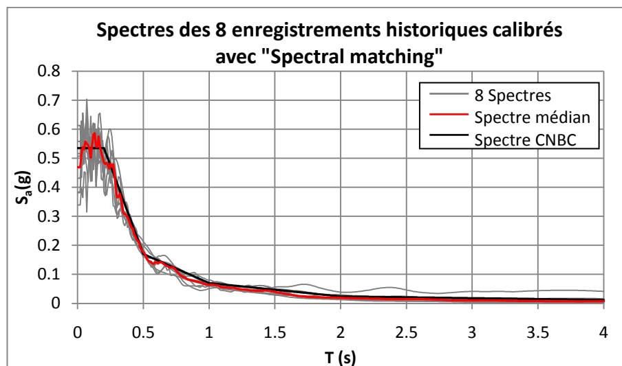
Figure 2.3 - Spectres des 8 enregistrements historiques calibrés avec "spectral matching"
