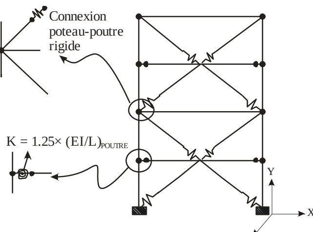
Figure 4.21 - Connexion des poutres
