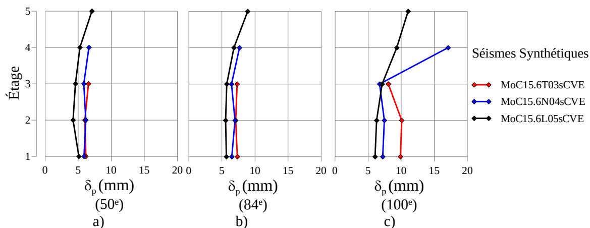
Figure 5.26 - Montréal hauteur d'étages: Demande de déformation ( \delta_p (mm)) : a) Médiane (50 e ); b) 84 e fractile; c) Maximum (100 e )
