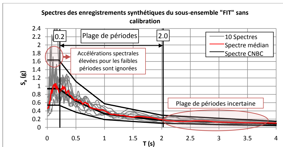
Figure 3.5 - Spectres des accélérogrammes sélectionnés du sous-ensemble FIT
