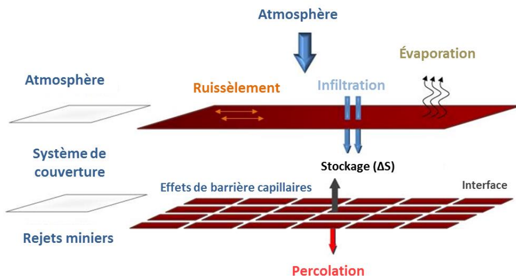
Figure 2.6 : Représentation schématique des composantes du bilan hydrique d'une couverture Store-and-release (1D) avec effet de barrière capillaire
