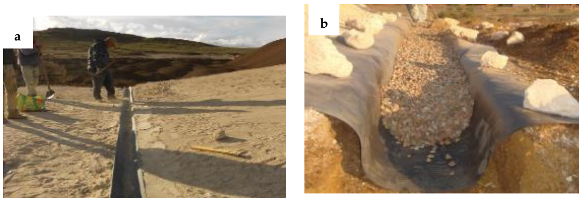
Figure 3.17 : Installation d'un drain de surface (a) et de la géomembrane pour récupérer les eaux s'écoulant à l'interface entre la couche de bris capillaire et la couche de rétention d'eau (b)
