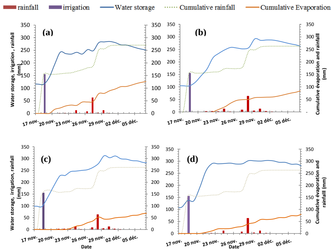
Figure G.1 : Bilan hydrique pour les 4 stations : 1 (a), 2 (b), 3 (c), and 4 (d).
