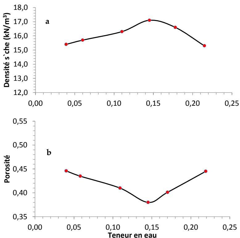
Figure 3.8 : Courbes densité sèche-teneur en eau (a) et porosité –teneur en eau (b) (Bossé, 2014)
