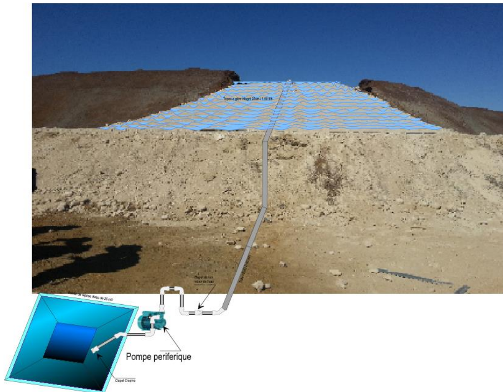
Figure A.12 : Schéma de la cellule inclinée avec système d'irrigation
