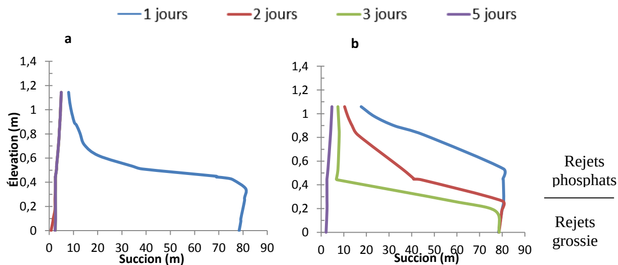
Figure 5.14 : Profils de suction matricielle avec (a) la courbe en drainage (MDC) et (b) la courbe en mouillage (MWC)
