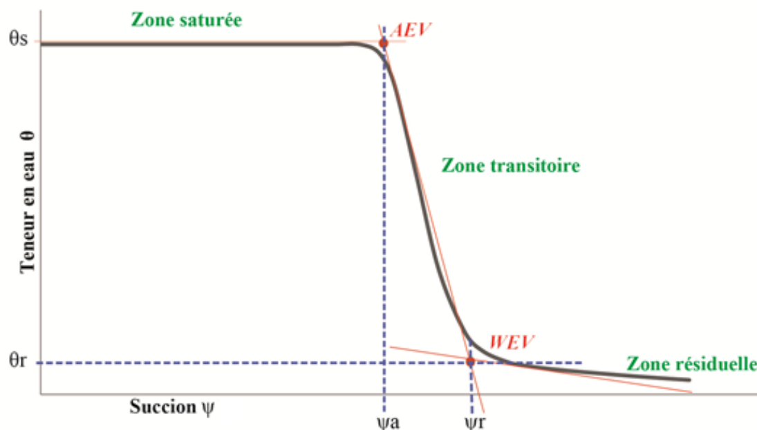
Figure 2.3 : Courbe de rétention d'eau (adapté de Fredlund et al. 2012)
