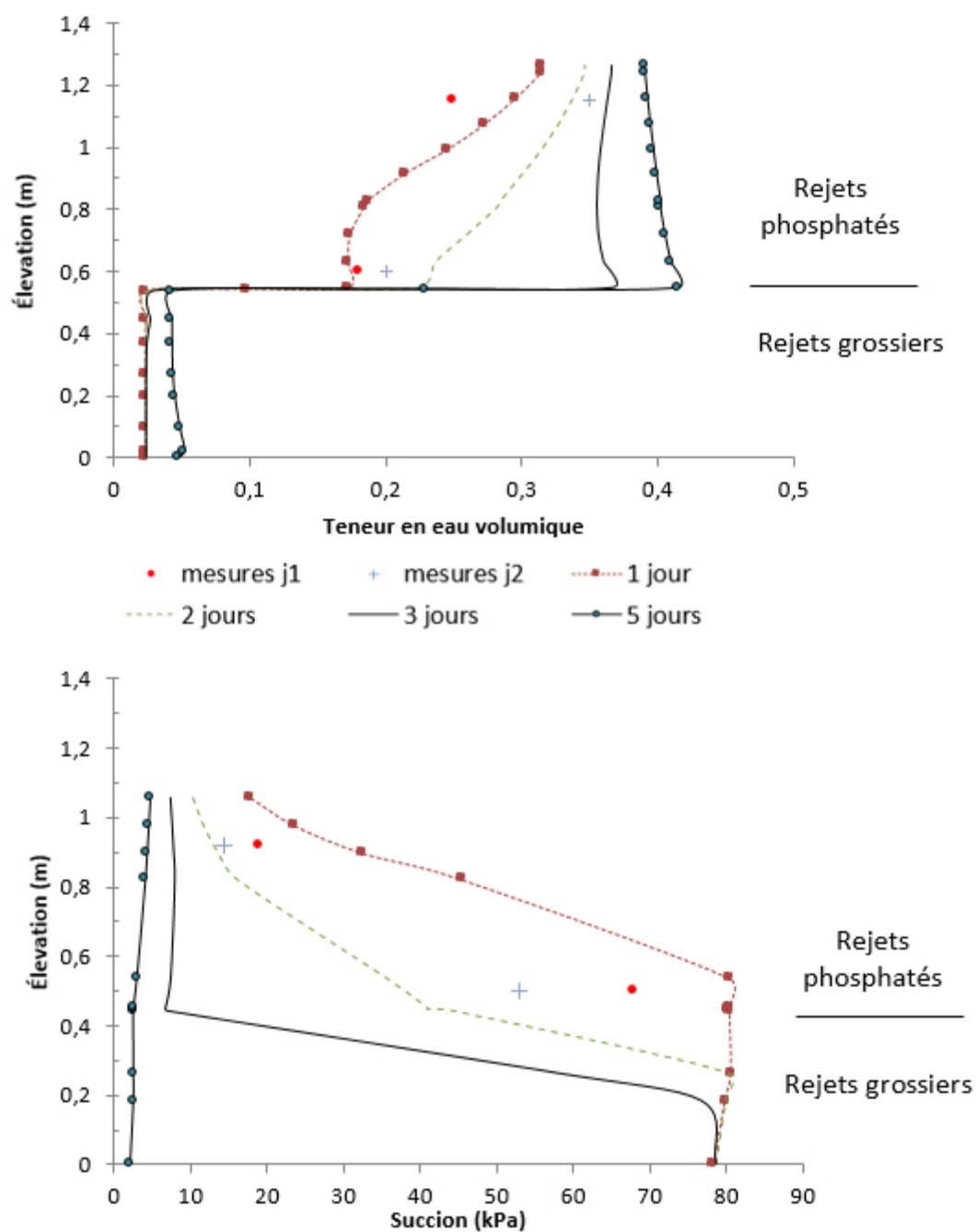
Figure 5.5 : Profils de teneur en eau et de suction prédits (symboles reliés) et mesurés (symboles non reliés) pour la station 3
