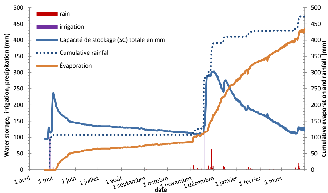
Figure G.3 : Bilan hydrique des 4 stations de mesures (station 1, 2, 3 et 4) d'avril 2014 à avril 2015.
