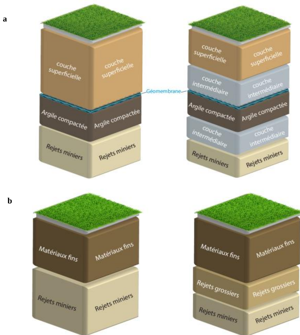
Figure J.1 : Systèmes de recouvrement conventionnel (a) et les recouvrements alternatifs type store-and-release (b) pour le contrôle du DMA
