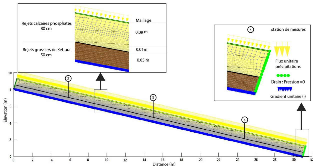
Figure 5.3 : Maillages et conditions frontières utilisés pour la modélisation numérique et emplacements des stations de mesures
