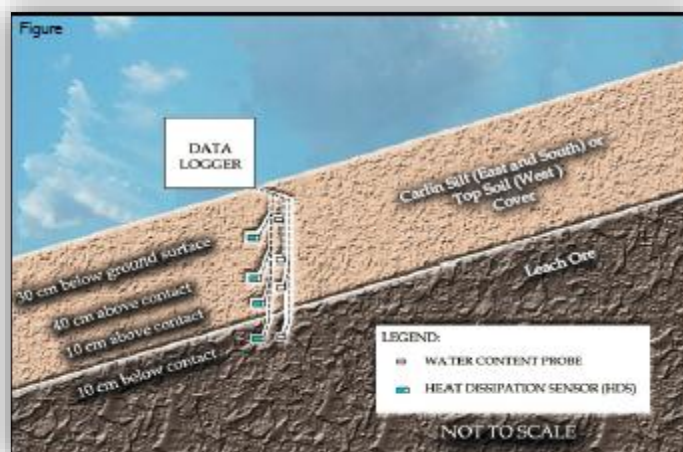
Figure 2.11: Représentation schématique du système de monitoring (Zhan et al. 2014)
