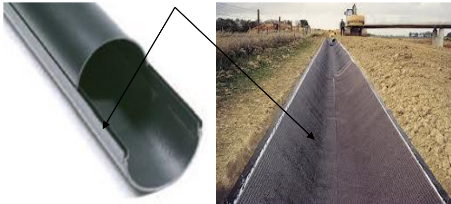
Figure A.8 : Exemples de drain
