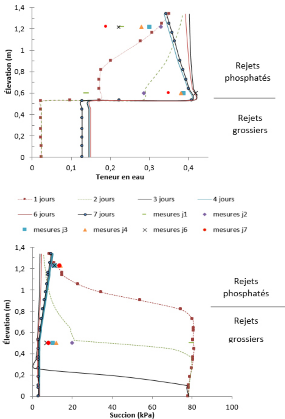
Figure 5.9 : Profils de teneur en eau et de suction prédits (symboles reliés) et mesurés (symboles non reliés) pour la station 2
