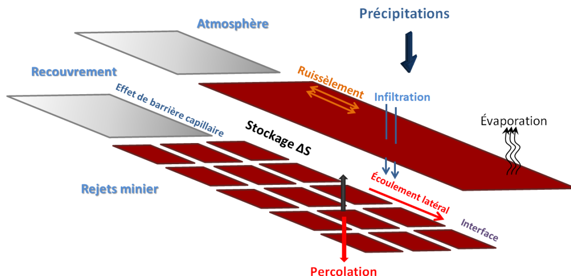
Figure 2.8 : Recouvrement SR inclinée avec les différentes composantes du bilan hydrique
