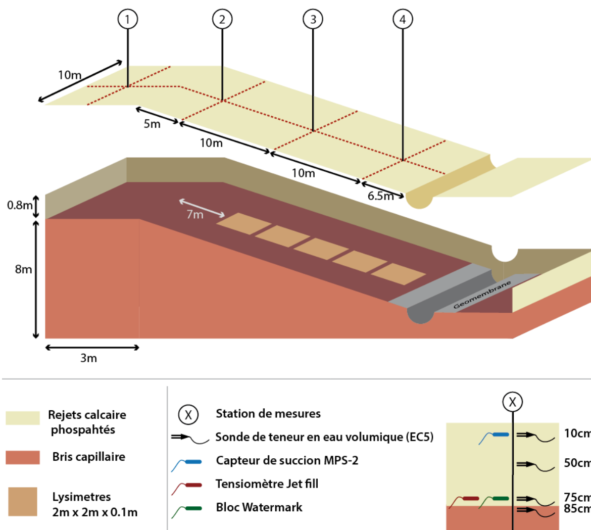
Figure 3.12 : Configuration schématique 3D de la cellule inclinée
