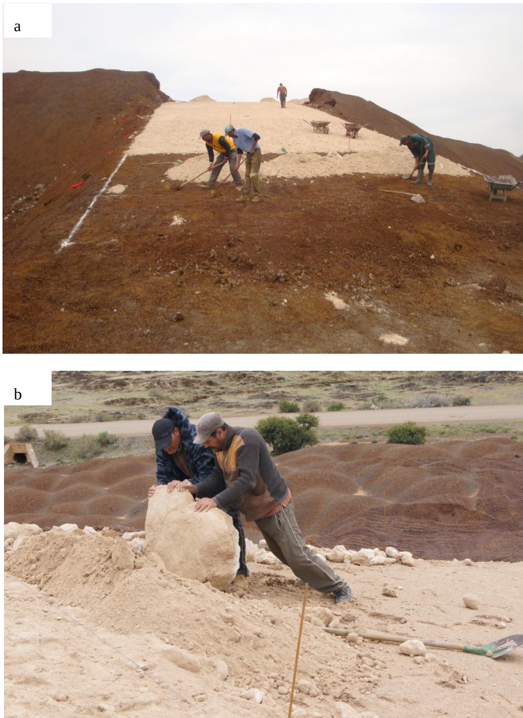
Figure C.4 : Mise en place de la couche calcaire
