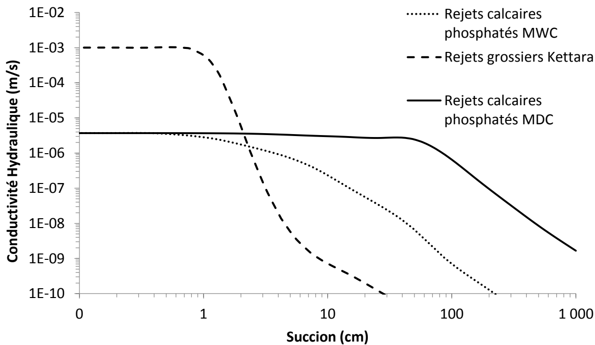
Figure 5.2 : Fonctions de perméabilité des matériaux utilisés dans les modélisations numériques
