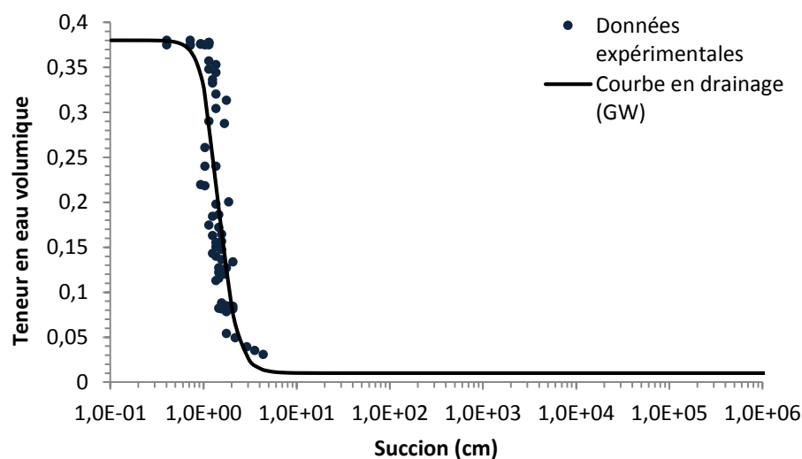
Figure 3.10 : Courbe de rétention d'eau (Bossé, 2014)
