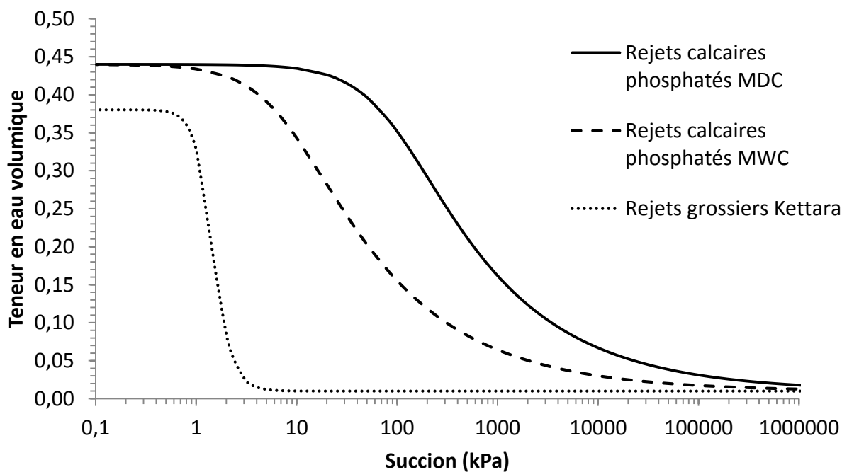
Figure 5.1 : Courbes de rétention d'eau des matériaux utilisés dans les modélisations numériques
