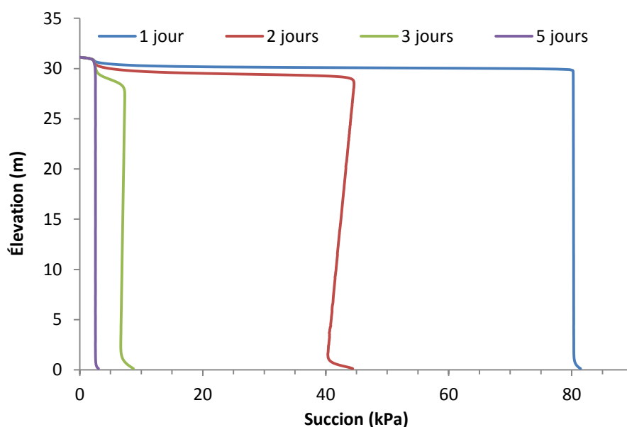
Figure 5.7 : Pressions à l'interface durant l'évènement de mouillage de 100 mm
