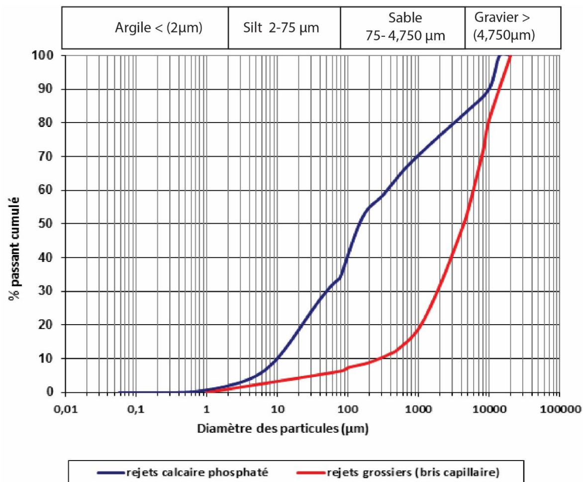
Figure 3.7 : Courbe granulométrique des deux composantes du recouvrement SR (rejets calcaires phosphatés et le bris capillaire)
