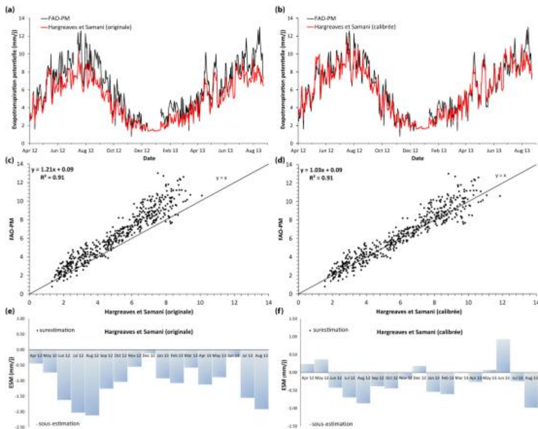
Figure I.2 : Comparaison des estimations de l'ETP, des droites de corrélations et des erreurs systématiques moyennes entre les formules de Hargreaves-Samani (originale ou calibrée) et le standard de Penman-Monteith.
