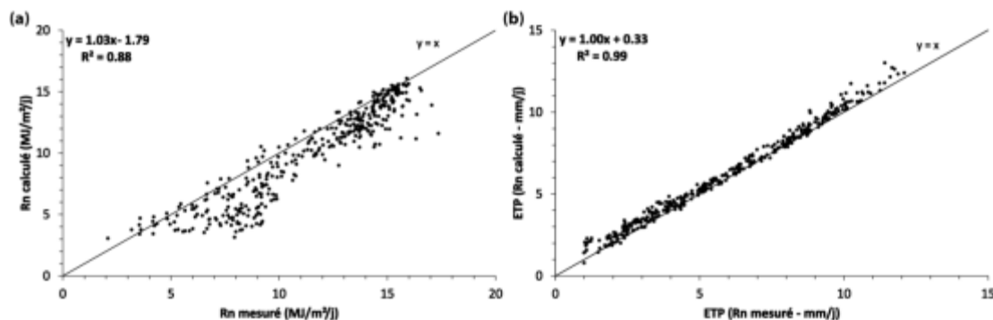
Figure I.1 : Droites de corrélation entre les estimations du rayonnement net (méthode direct/indirecte) (a) et des ETP résultantes (b).
