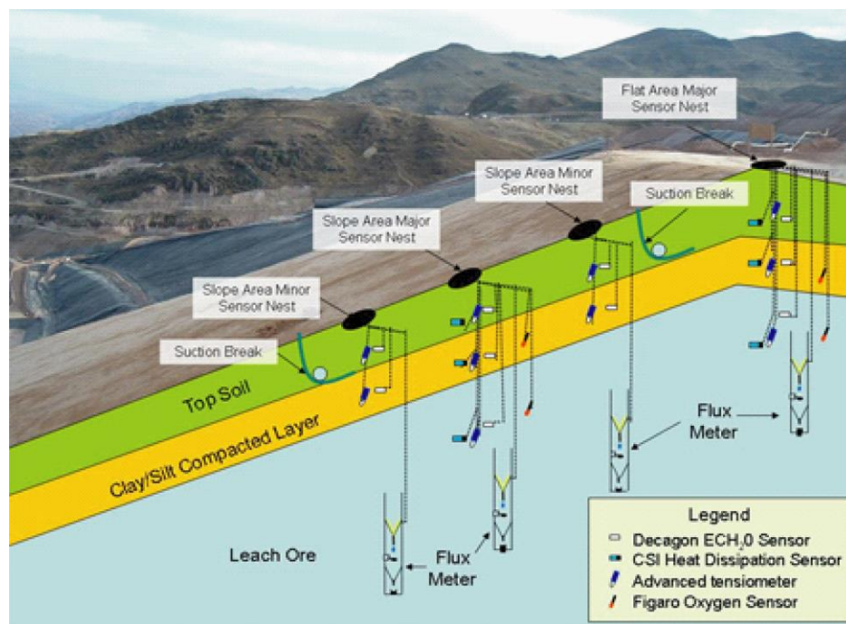
Figure A.3 : Exemple d'installation du matériel de mesure dans un système incliné (Zhan et al.2007)
