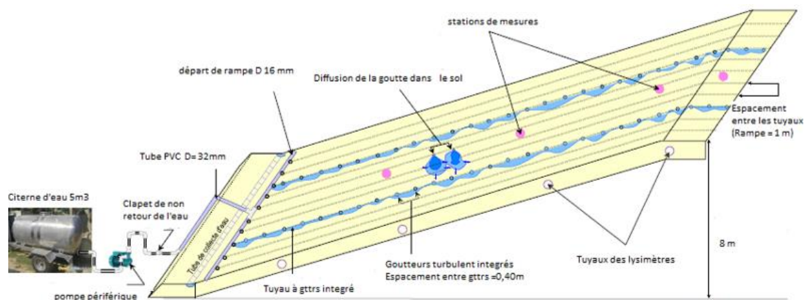
Figure A.10 : Simulation d'événements extrêmes pour le système incliné
