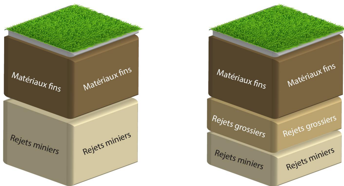
Figure 2.5 : Systèmes de recouvrement pour le contrôle du DMA par réduction des infiltrations d'eau (Adapté de Bossé, 2014)
