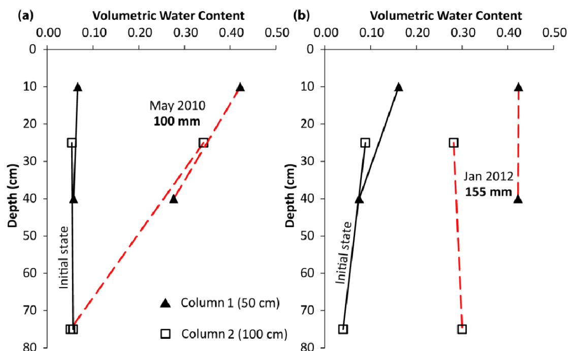
Figure 3.4 : Profil de teneur en eau volumique : (a) simulation d'un événement extrême de 100 mm; (b) simulation d'un événement extrême de 155 mm (Bossé et al. 2013)
