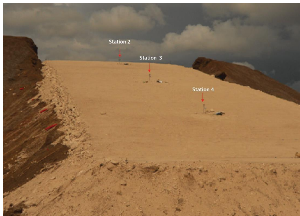
Figure 3.18 : Stations de mesures 2, 3 et 4 de la cellule inclinée (la station 1 est sur la partie plane en haut de la pente)
