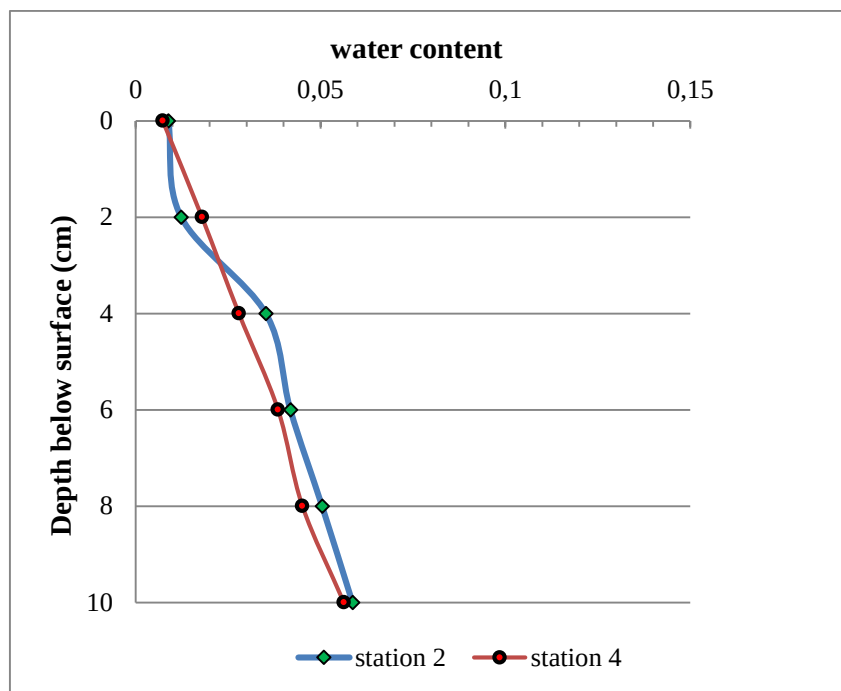
Figure E.2 : Résultats de teneur en eau de 0 à 10 cm de profondeur pour la station 2 et 4
