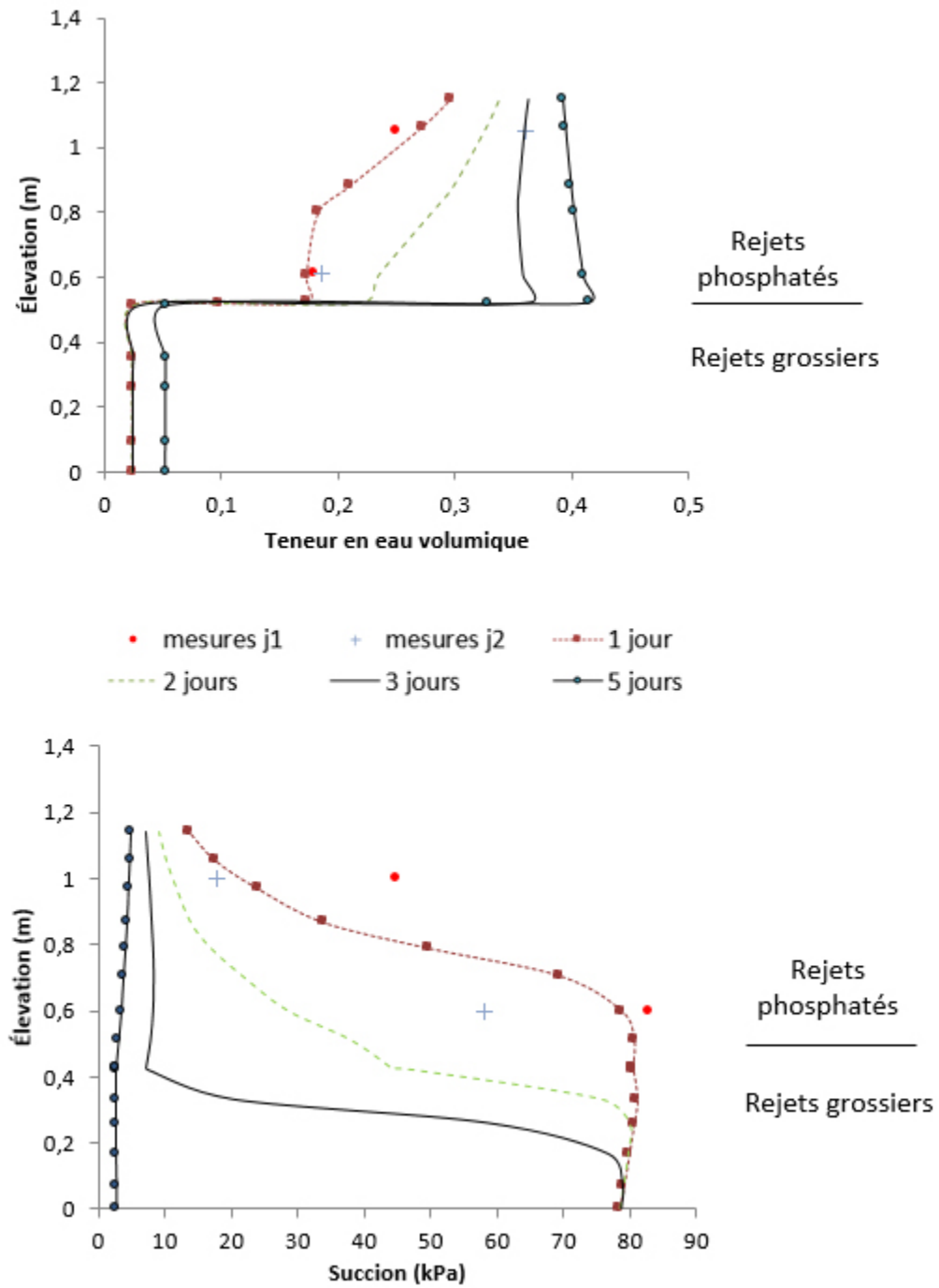
Figure 5.6 : Profils de teneur en eau et de suction prédits (symboles reliés) et mesurés (symboles non reliés) pour la station 4
