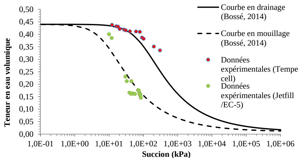
Figure 3.9 : CRE obtenues par mesures expérimentales en cellule de Tempe, par mesures directes de terrain et CRE obtenues par Bossé (2014)
