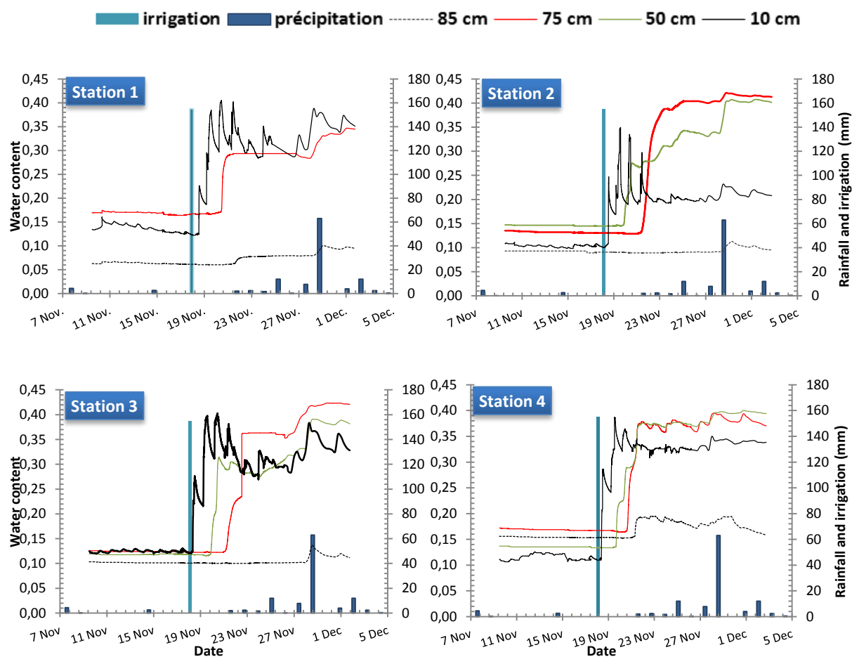
Figure G.2 : Évolution de la teneur en eau volumétrique à 10, 50, 75 et 85 cm de profondeur pour les 4 stations de la couverture SR expérimentale inclinée durant l'évènement de mouillage de 155mm
