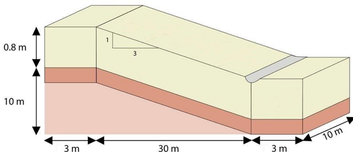
Figure A.2 : Représentation schématique 3D d'une cellule expérimentale
