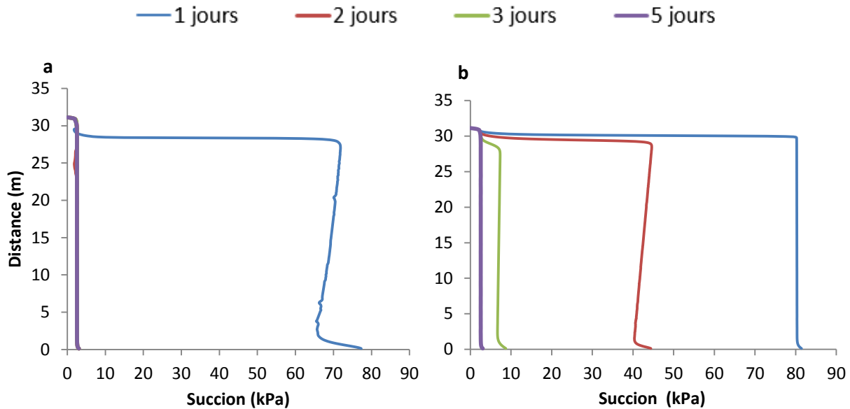
Figure 5.15 : Pressions à l'interface obtenue avec (a) la courbe en drainage (MDC) et (b) la courbe en mouillage (MWC)
