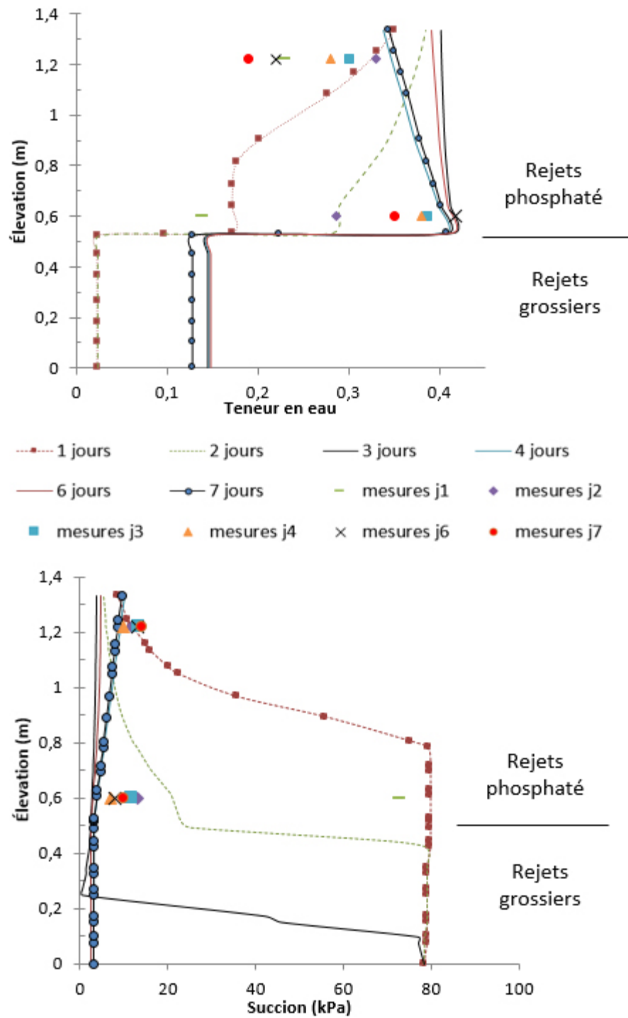
Figure 5.10 : Profils de teneur en eau et de suction prédits (symboles reliés) et mesurés (symboles non reliés) pour la station 3
