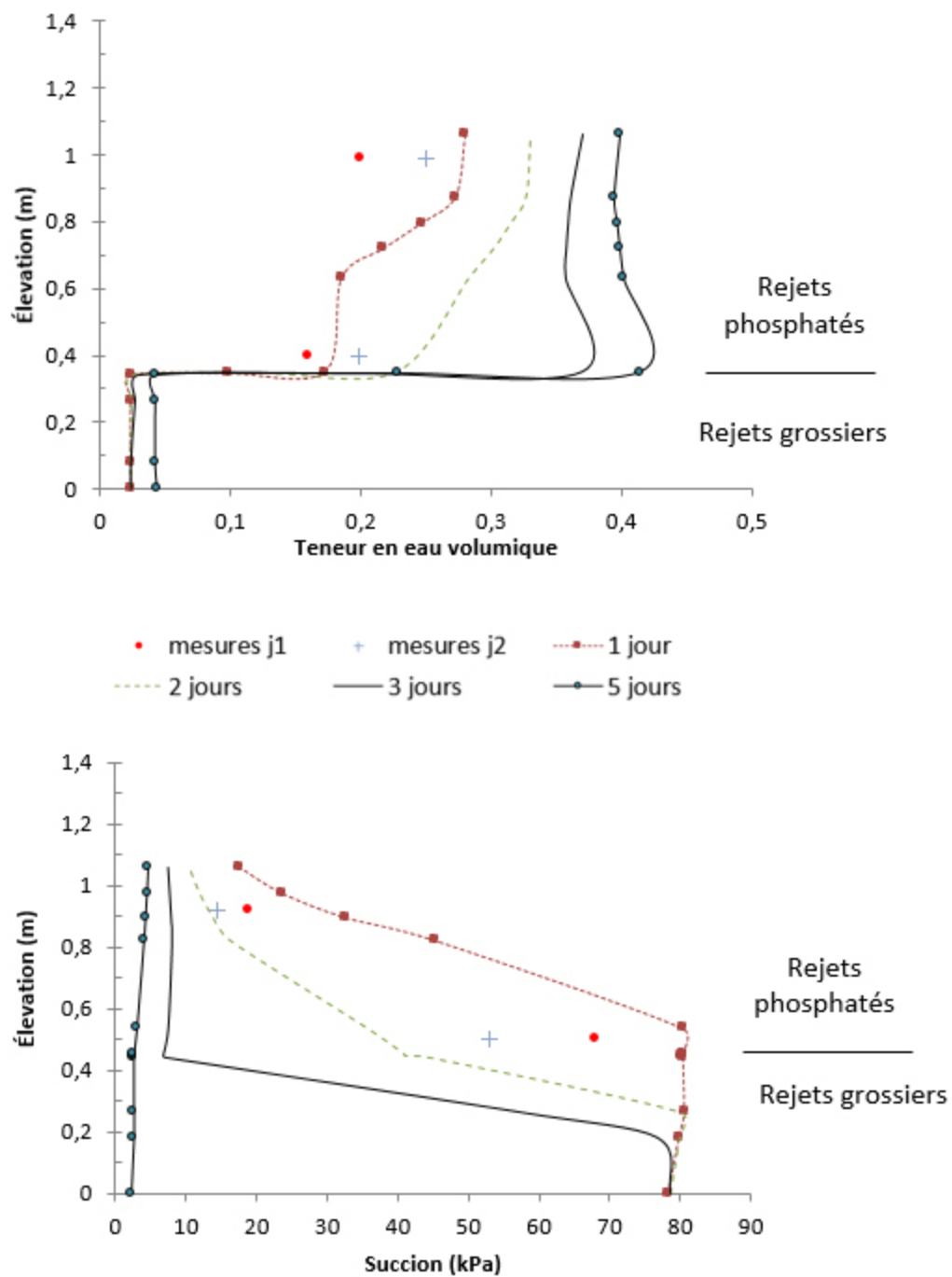
Figure 5.4 : Profils de teneur en eau et de suction prédits (symboles reliés) et mesurés (symboles non reliés) pour la station 2
