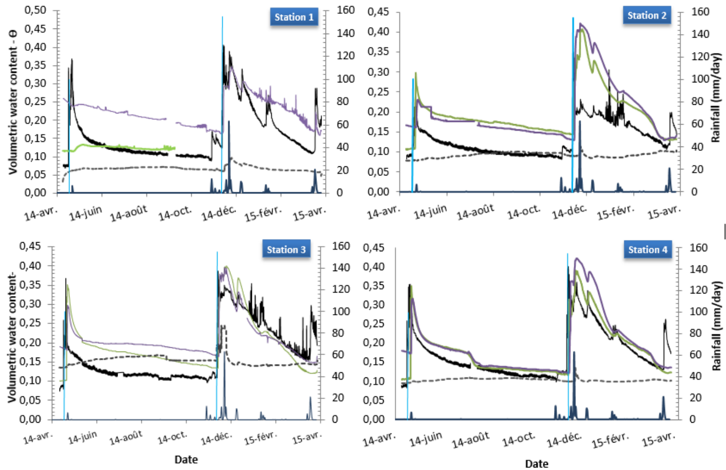
Figure G.4: Évolution de la teneur en eau volumétrique à 10, 50, 75 et 85 cm de profondeur pour les 4 stations de la couverture SR expérimentale inclinée d'Avril 2014 à Avril 2015
