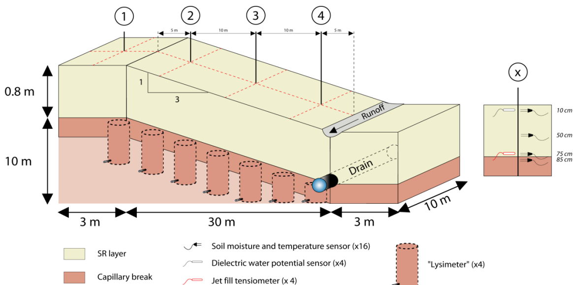
Figure A.5 : Représentation schématique 3D d'une cellule expérimentale inclinée avec 4 stations de mesure
