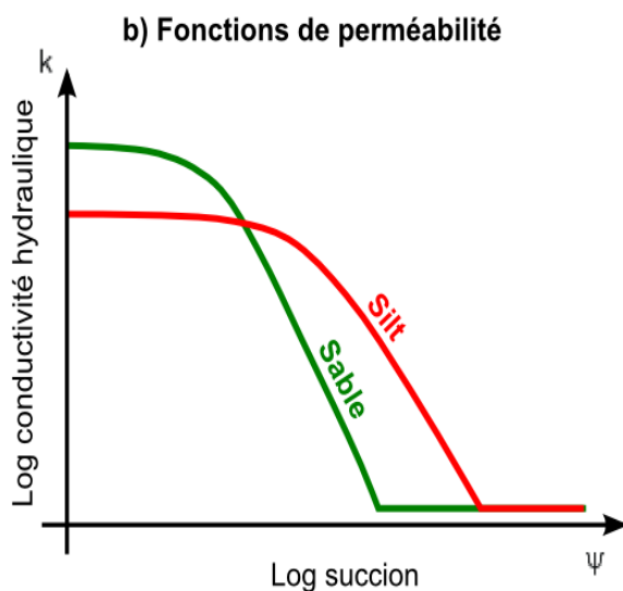
Figure 2.4 : Fonctions de perméabilité d'un sable et d'un silt (Aubertin et al. 2015)
