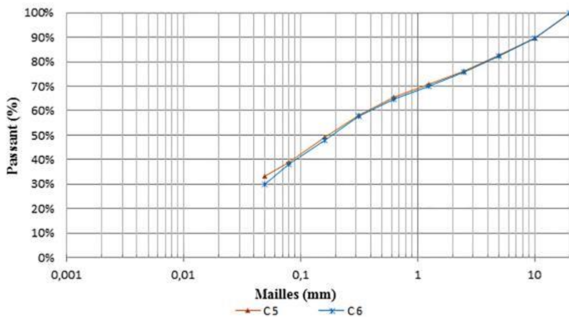
Figure E.1 : Essais de granulométrie
