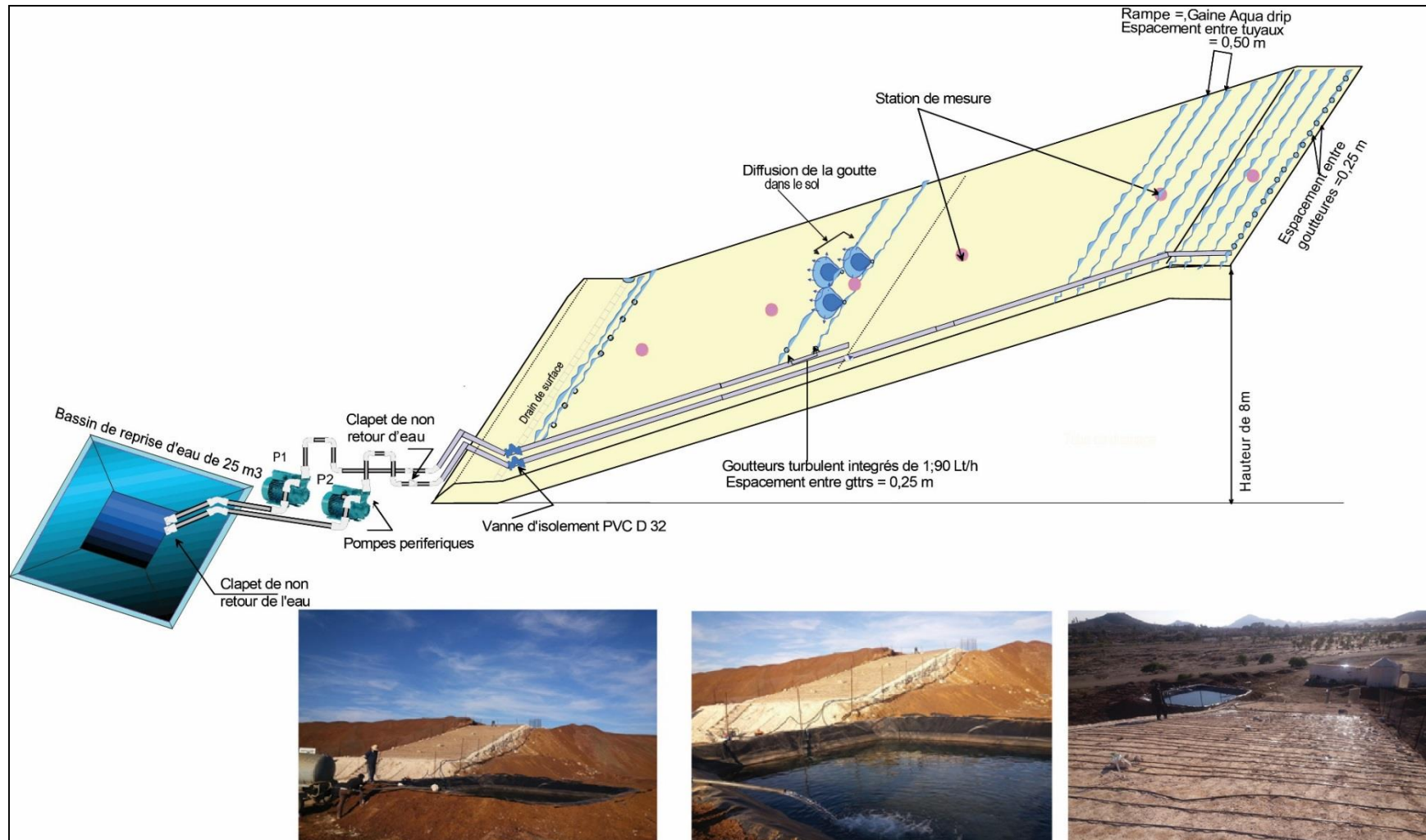
Figure 3.26 : Mise en place du système d'irrigation pour simuler 155 mm
