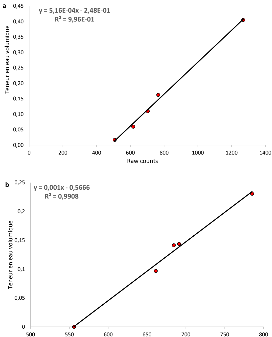
Figure D.1 : Courbes de calibration des sondes EC-5 pour les rejets grossiers et les rejets calcaires phosphatés de Kettara
