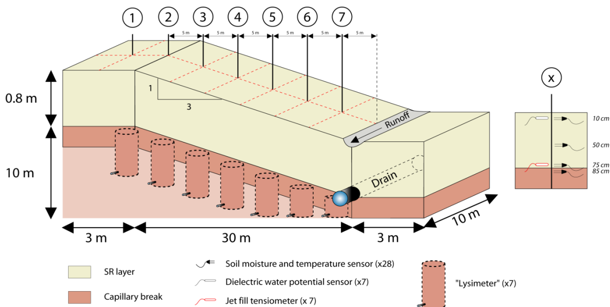
Figure A.4 : Représentation schématique 3D d'une cellule expérimentale inclinée avec 7 stations de mesures
