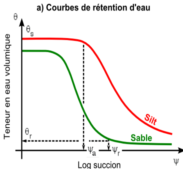
Figure 2.2 : Courbe de rétention d'eau d'un sable et d'un silt (Aubertin et al. 2015)
