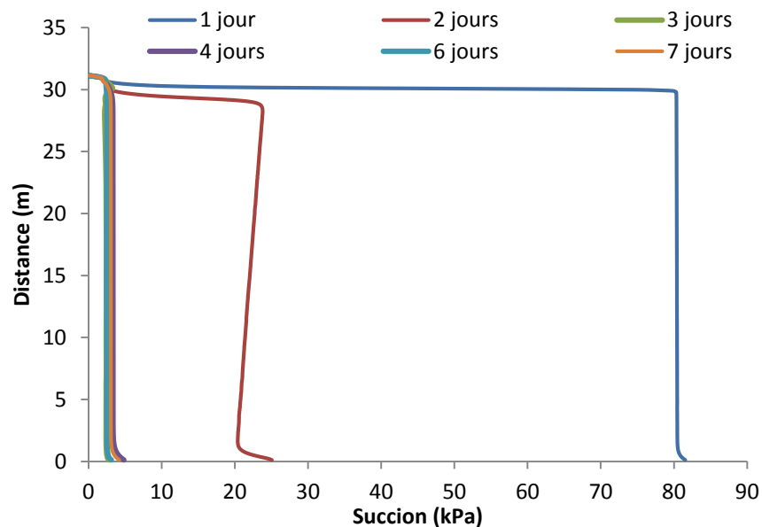
Figure 5.12 : Pressions à l'interface durant l'évènement de mouillage de 155 mm
