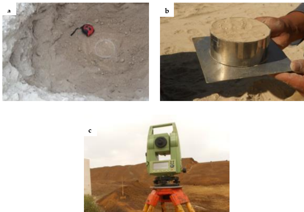
Figure 3.23 : Essais de contrôle qualité : a) et b) mesure de la porosité in situ; c) mesure de l'angle de la pente à l'aide d'une station totale
