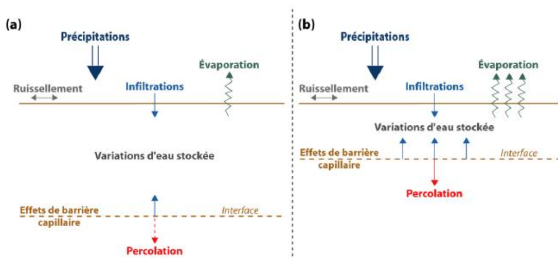
Figure 2.7 : Comportement hydrogéologique de deux recouvrements SR d'épaisseur de 100 (a) et 50 (b) cm (Bossé, 2014).
