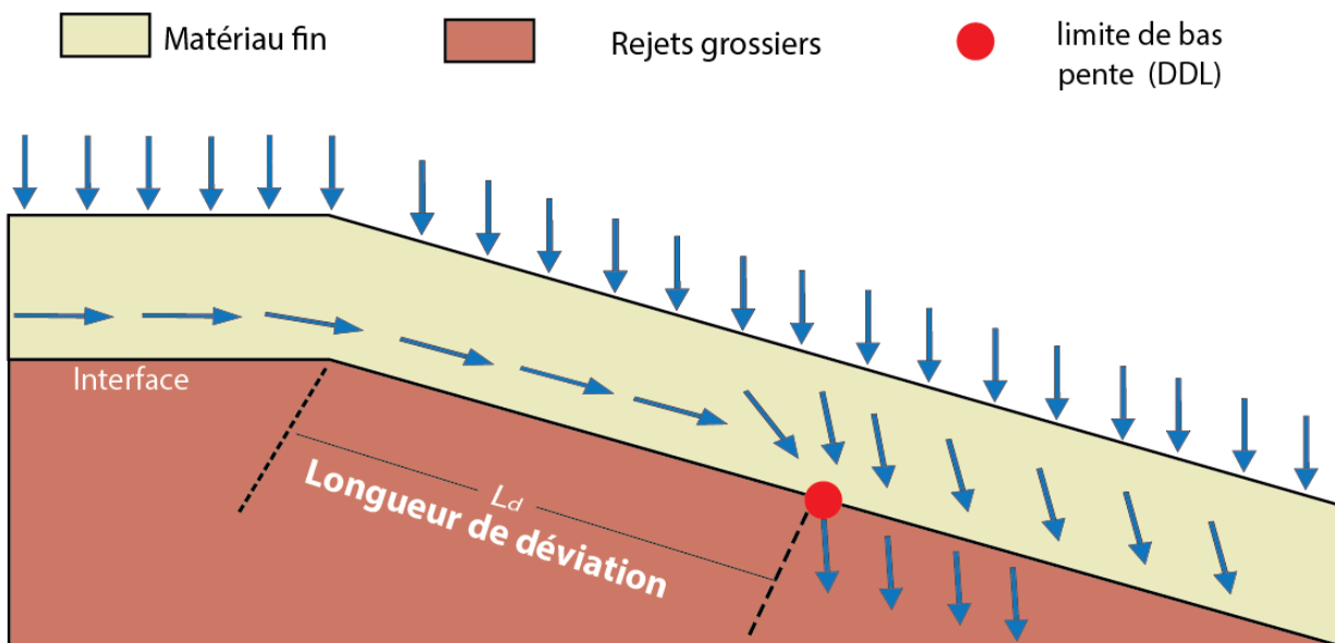
Figure 2.9 : Représentation schématique de l'écoulement d'eau à travers une couverture inclinée et rupture du bris capillaire au point DDL représenté par le point rouge (adapté de Bussière, 1999)
