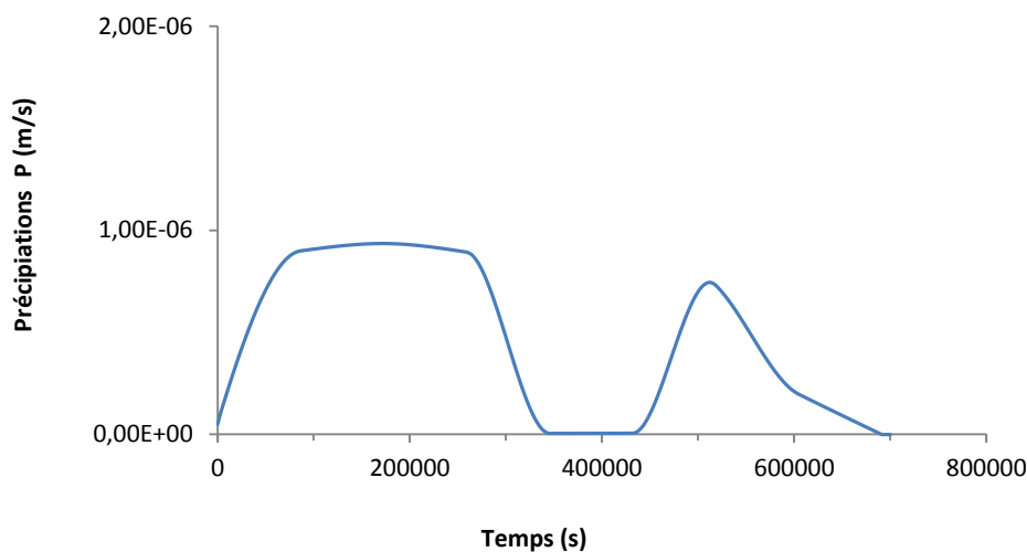
Figure 5.8 : Fonction de précipitations appliquée comme condition frontière durant le régime transitoire
