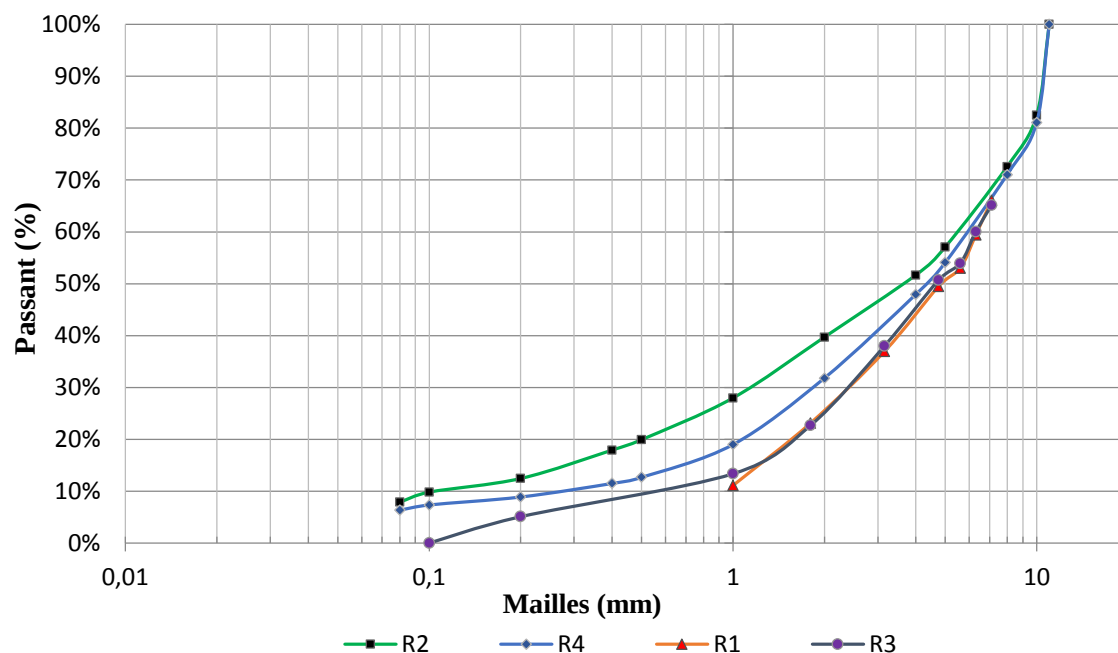
Figure 3.21 : Courbes granulométriques typiques des rejets grossiers de Kettara (bris capillaire)
