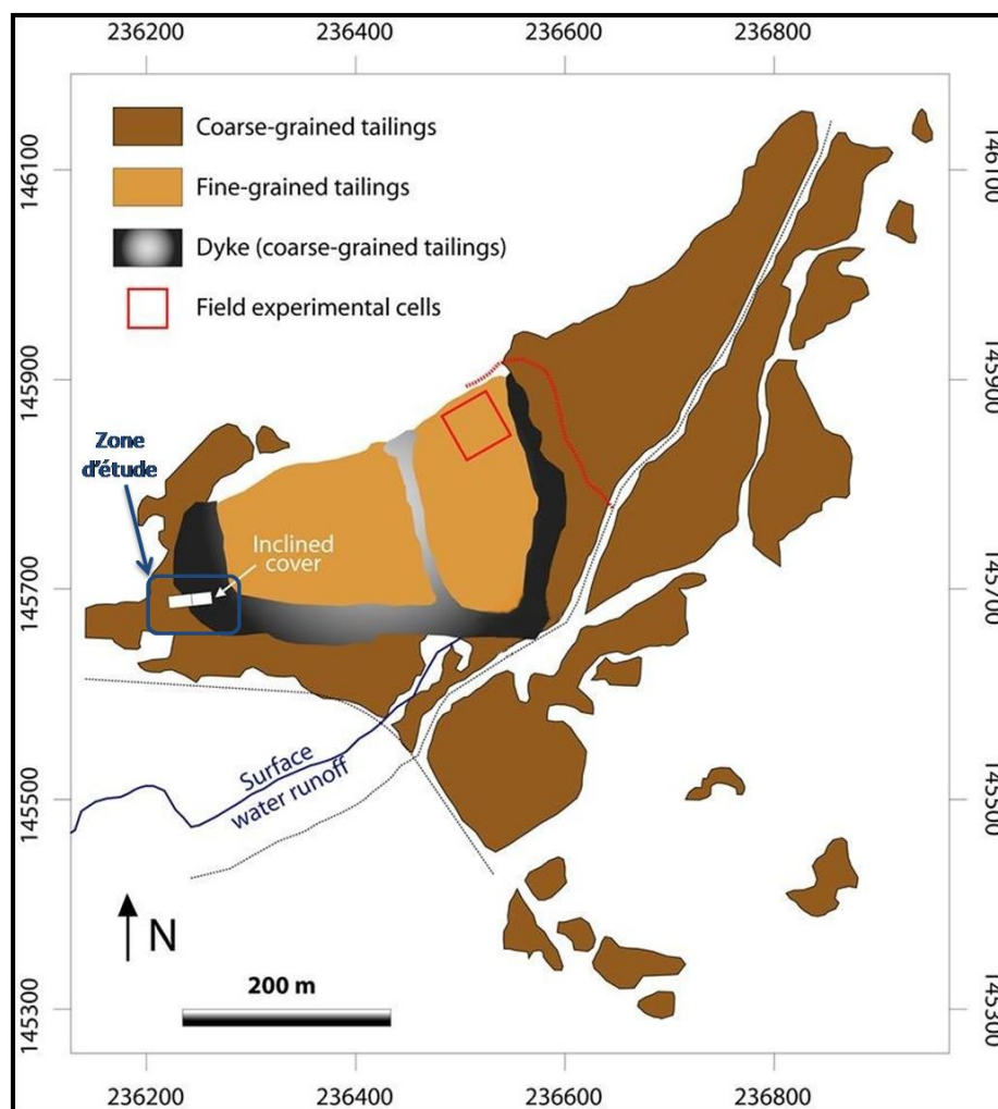
Figure A.1 : Zone d'étude expérimentale avec une largeur de 10m et une hauteur de 11m (Bossé et al. 2014).
