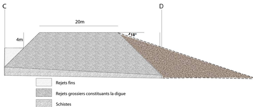
Figure A.6 : Aplanissement de la pente de 45^\circ à 14^\circ .
