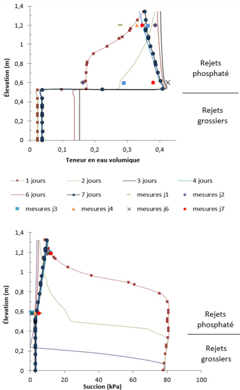
Figure 5.11 : Profils de teneur en eau et de succion prédits (symboles reliés) et mesurés (symboles non reliés) pour la station 4
