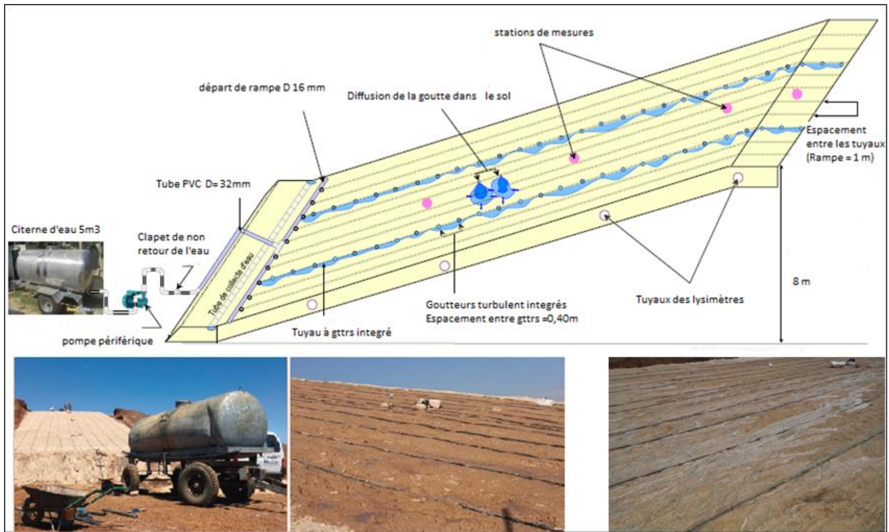
Figure 3.25 : Mise en place du système d'irrigation pour simuler 100 mm
