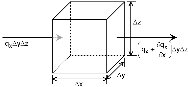
Figure 2.1: Écoulement d'eau à travers un élément de sol (d'après Hillel, 1988)
