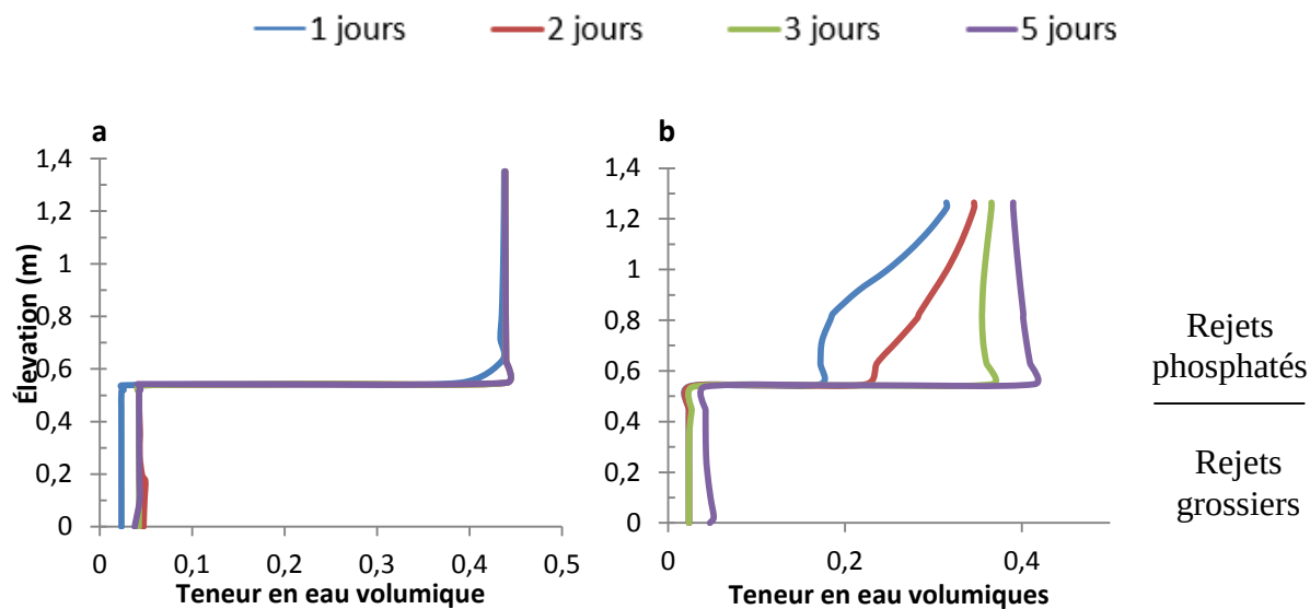
Figure 5.13 : Profils de teneur en eau en utilisant (a) la courbe en drainage (MDC) et (b) la courbe en mouillage (MWC)
