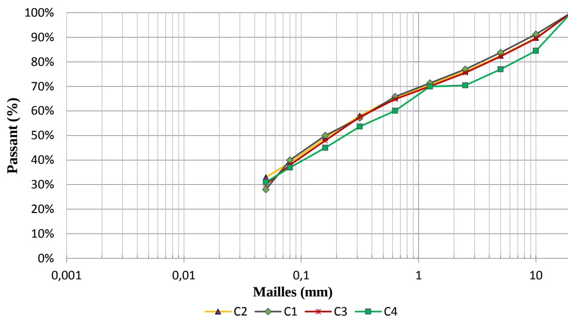
Figure 3.22 : Courbes granulométriques des rejets calcaires phosphatés
