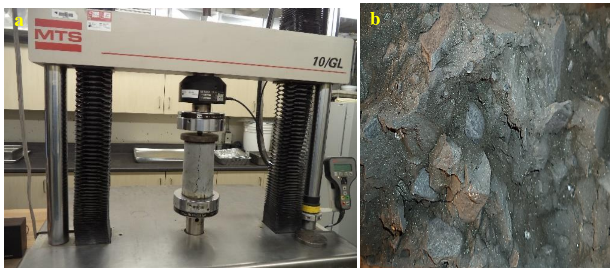
Figure 3.12 : Éssai de compression uniaxiale sur un échantillon de remblai mixte (a) et vue intérieure du remblai après cassage (b)
