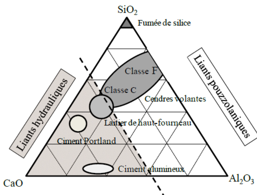
Figure 2.2 : Diagramme ternaire \text{CaO}-\text{Al}_2\text{O}_3-\text{SiO}_2 montrant la composition chimique de quelques liants hydrauliques et pouzzolaniques (Coussy, 2011)
