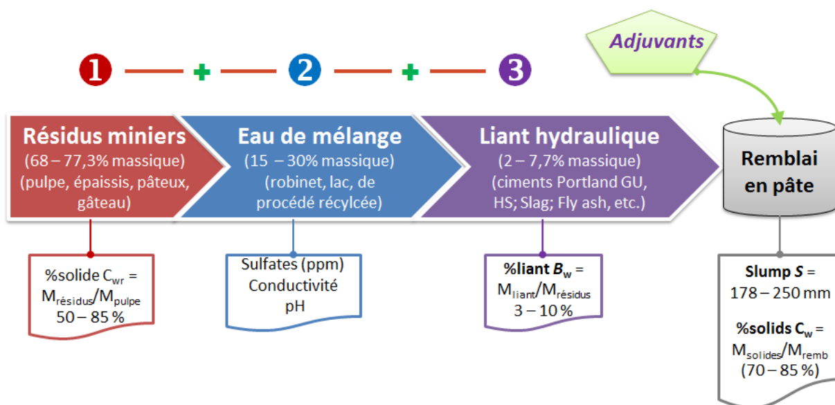
Figure 1.2 : Les différentes composantes du remblai en pâte cimentés (Belem, 2013)
