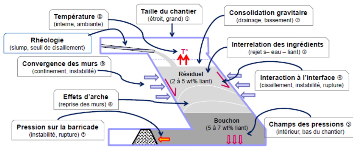
Figure 2.5 : Principaux facteurs influençant la résistance mécanique du RPC (Belem, 2009)
