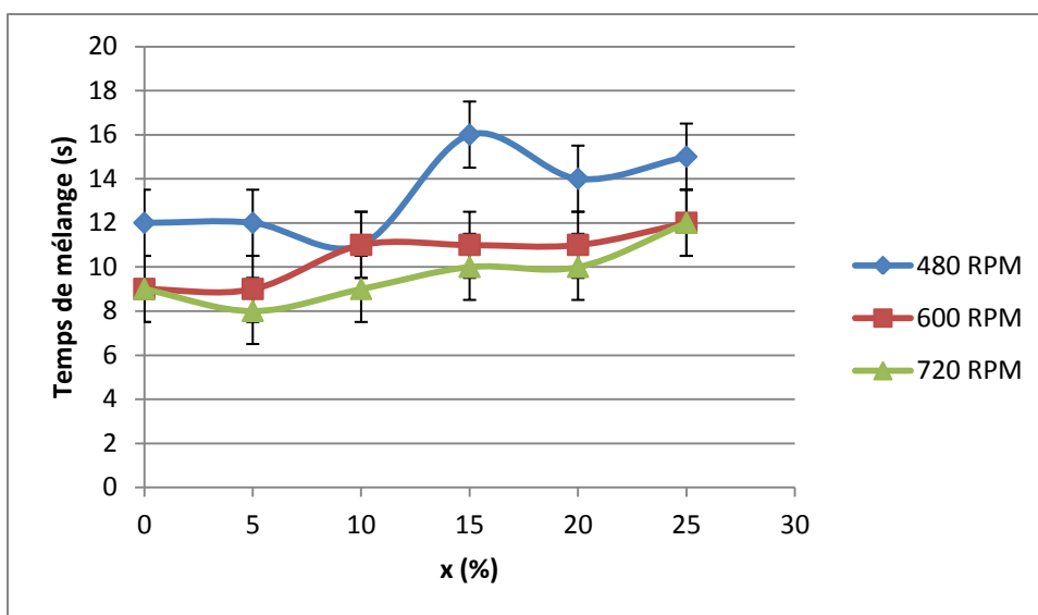
Figure 4. 15 : Temps de mélange en fonction de la fraction massique de solides pour chaque vitesse de rotation (Maxblend c=1'' )
