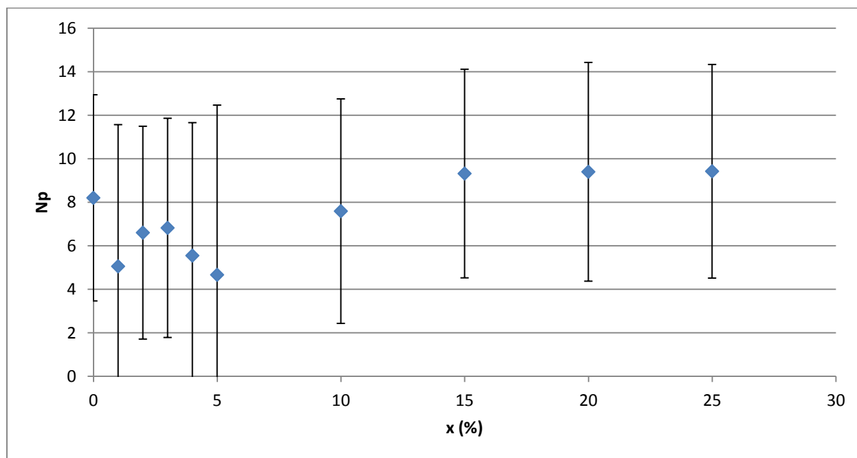
Figure B. 10 : Nombre de puissance moyen en fonction de la fraction massique pour Re > 20000 (Maxblend 1'')
