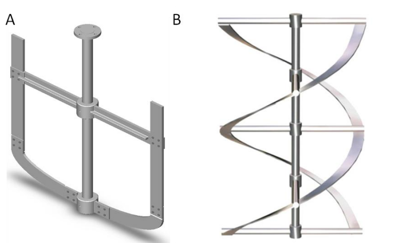
Figure 2. 1 : Exemples de mobiles d'agitation utilisés en régime laminaire. A : Ancre (Post Mixing Optimization and Solutions, LLC, 2013). B : Ruban hélicoïdal (Shandong OUMI Machinery Manufacturing Co.,Ltd, 2015).
