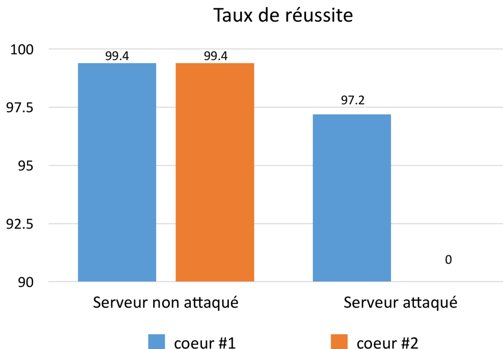
Figure 5.9 Taux de réussite : rapport entre nombre de tâches traitées et nombre de tâches reçues dans le modèle "IaaS". Chaque cœur représente une machine virtuelle du serveur
