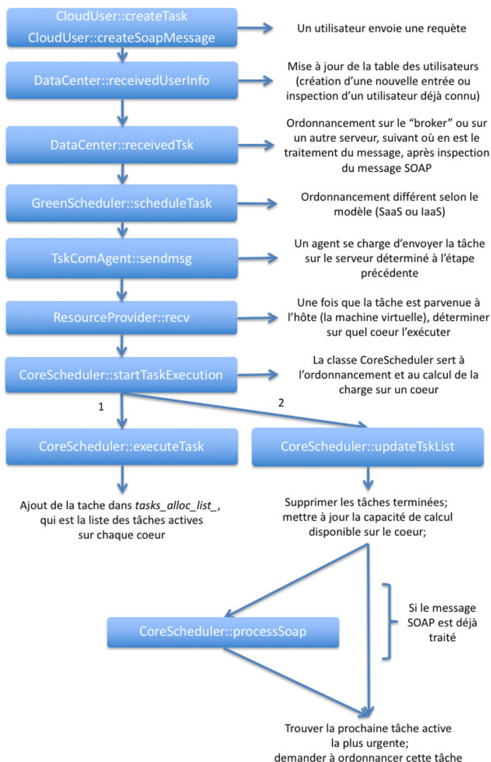
Figure 3.2 Nouveau schéma de fonctionnement après modifications du simulateur GreenCloud
