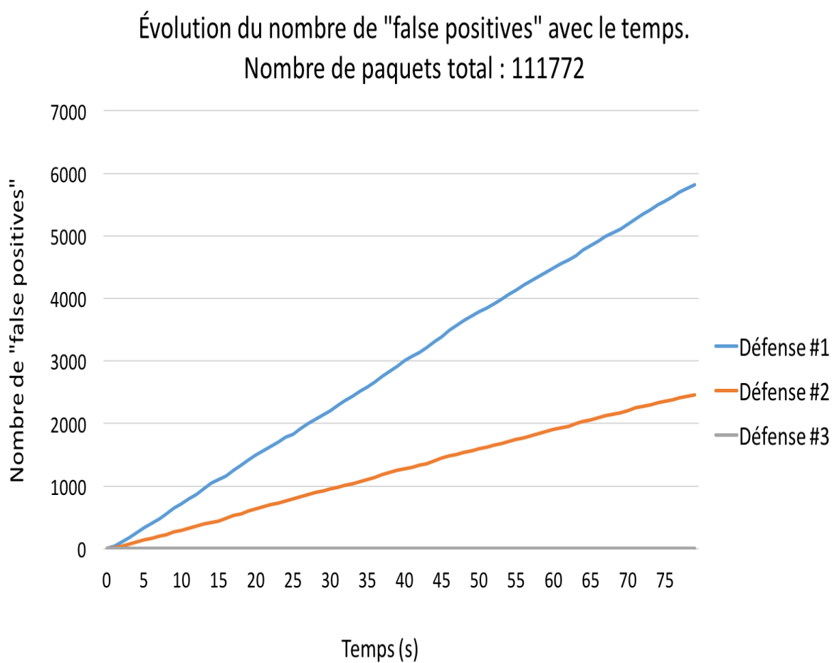
Figure 5.10 Évolution du nombre de "false positives" avec le temps, en fonction des différents degrés de défense
