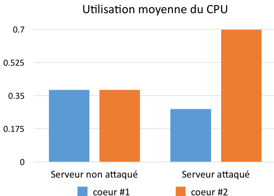
Figure 5.7 Utilisation moyenne du CPU dans le modèle "IaaS", chaque coeur du serveur est attribué à une des machines virtuelles (2 machines virtuelles par serveur).
