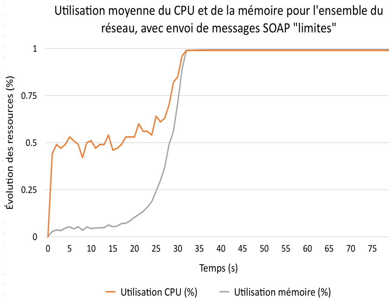
Figure 5.13 Évolution des ressources du réseau avec envoi de paquets à la limite de ce qu'autorise la défense
