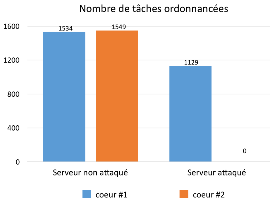
Figure 5.8 Nombre moyen de tâches ordonnancées dans le modèle "IaaS", chaque coeur du serveur est attribué à une des machines virtuelles (2 machines virtuelles par serveur)
