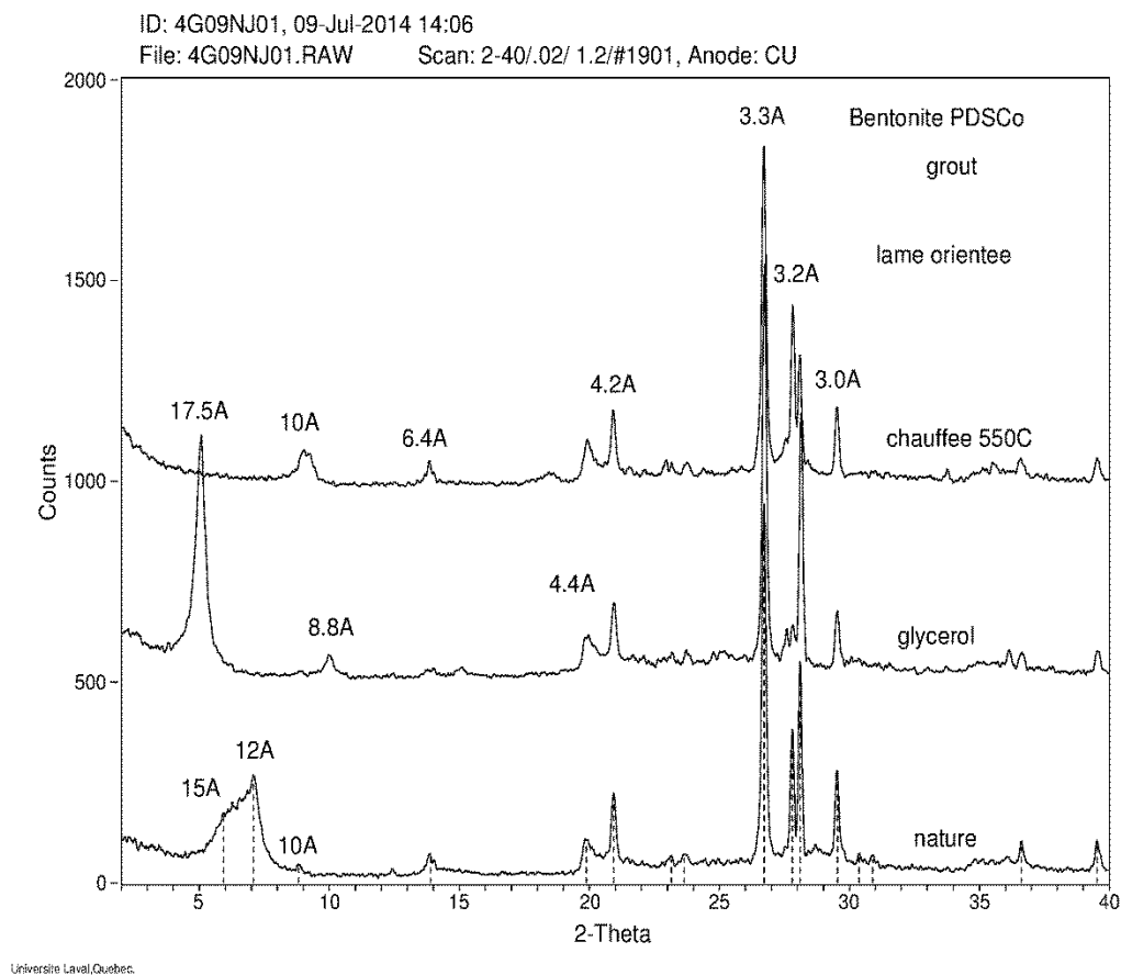
Diffractogramme de la bentonite.
