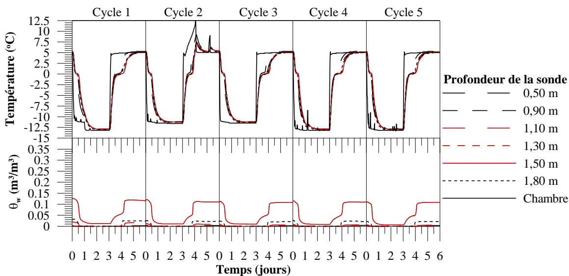
Figure 5.4: Évolution des températures et des teneurs en eau volumiques mesurées lors des phases de gel-dégel pour les différentes sondes de la colonne 2.
