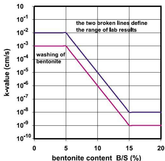
Figure 2.7: Plage de variation type de la conductivité hydraulique saturée pour plusieurs sables propres en fonction de la teneur en bentonite (Chapuis, 2002b).
