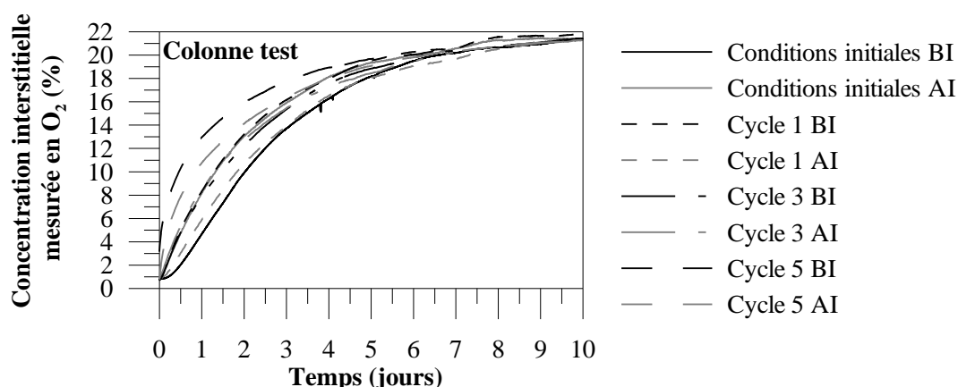
Figure 5.2: Valeurs de la concentration interstitielle mesurée en \text{O}_2 en fonction du temps lors des essais de diffusion d'oxygène obtenus pour la colonne test après drainage et aux conditions expérimentales des colonnes 1, 2 et 3 avant (BI) et après (AI) infiltration.
