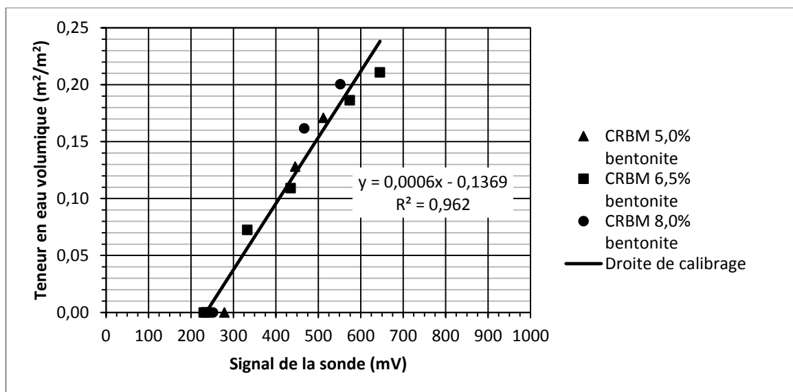
Droite de calibrage des sondes 5TM à 5°C.
