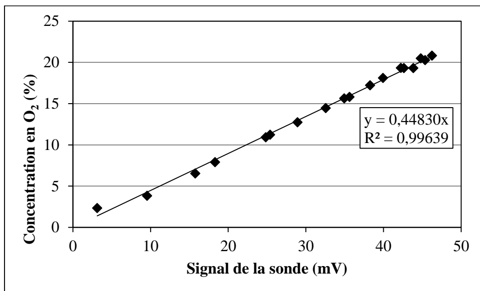
Concentration d'oxygène interprétée en fonction du signal de la sonde pour la colonne 2.
