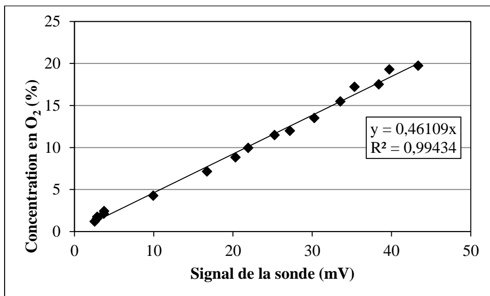
Concentration d'oxygène interprétée en fonction du signal de la sonde pour la colonne 3.
