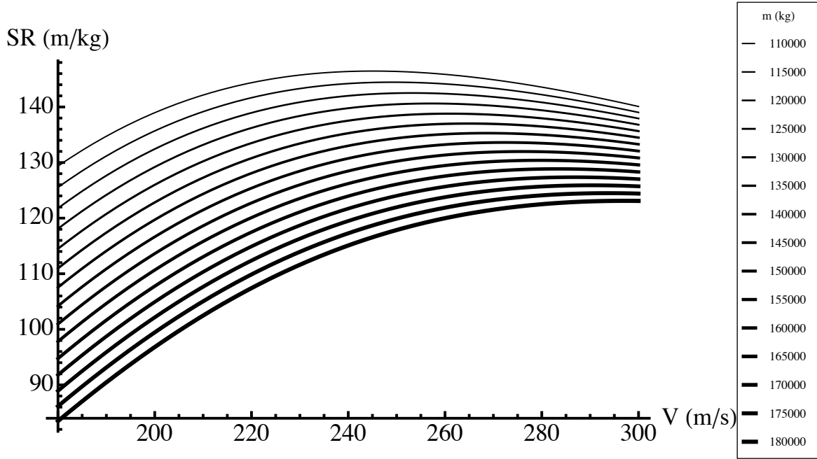
Figure 4.9 Graphes de la distance spécifique SR en fonction de la vitesse V pour différentes valeurs de la masse m .
