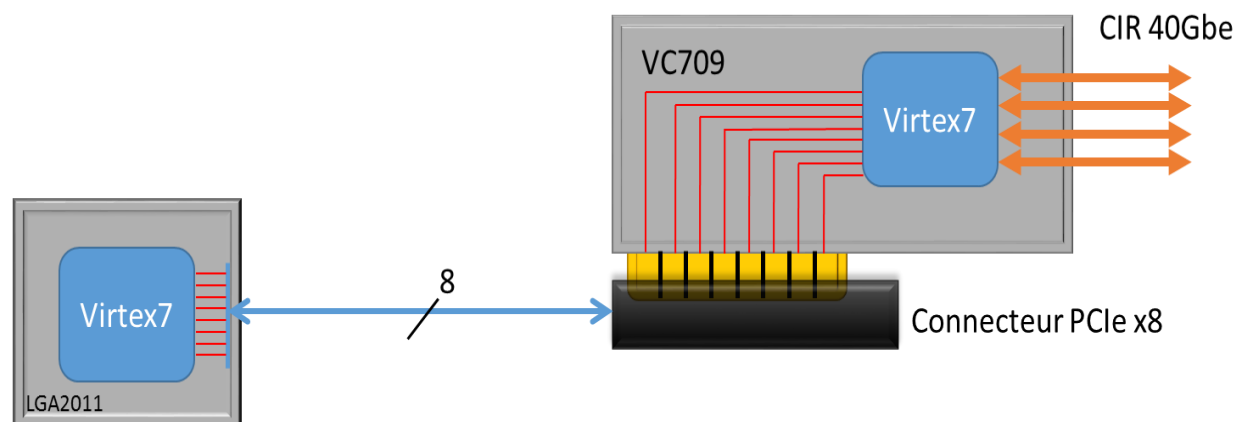
Figure 3-13 Connexion filaire entre le VC709 et le Virtex 7 « in-socket »
