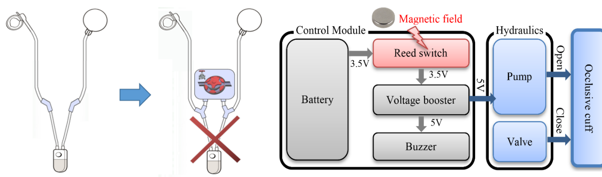
Figure 4-3: Illustration du concept proposé pour notre troisième génération de SUA
