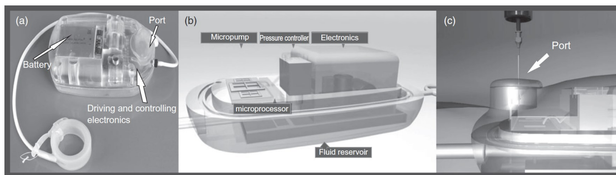
Figure 3-9: GAAS II et ses différents composants [68]
