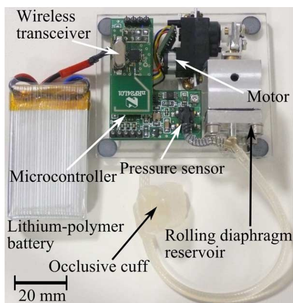
Figure 3-7: Illustration de AAUS et de ses composants internes. (© 2012 IEEE, [63])
