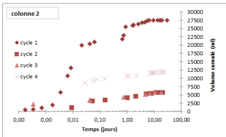
Évolution des volumes d'eau récupérés à la base des colonnes 1 et 2
