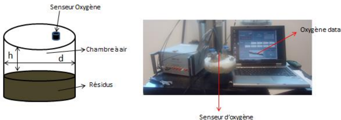
Figure 3-1 : Dispositif expérimental mis en œuvre pour les essais de consommation d'oxygène
