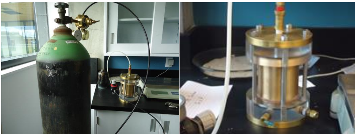
Figure 3-5 : Essais de rétention d'eau en cellule Tempe
