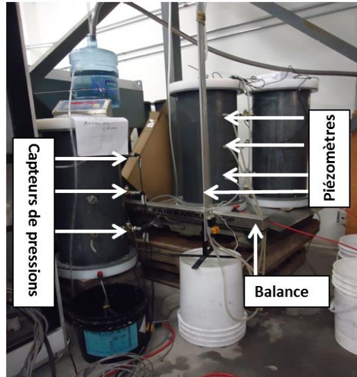
Figure 3-3: Déroulement des essais de perméabilité en colonne
