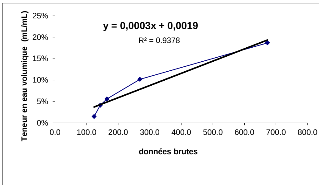
Droite de calibration de la sonde GS-3
