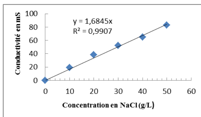
Figure 3-8 : Droite de calibration du conductimètre
