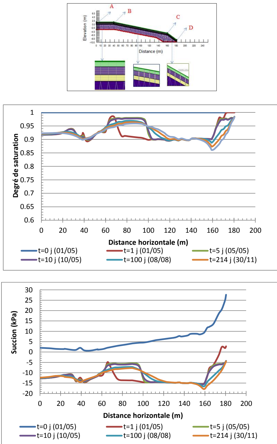
Figure 5-14 : Degré de saturation et profil de suction au milieu de la couche de rétention d'eau en fonction de la distance horizontale
