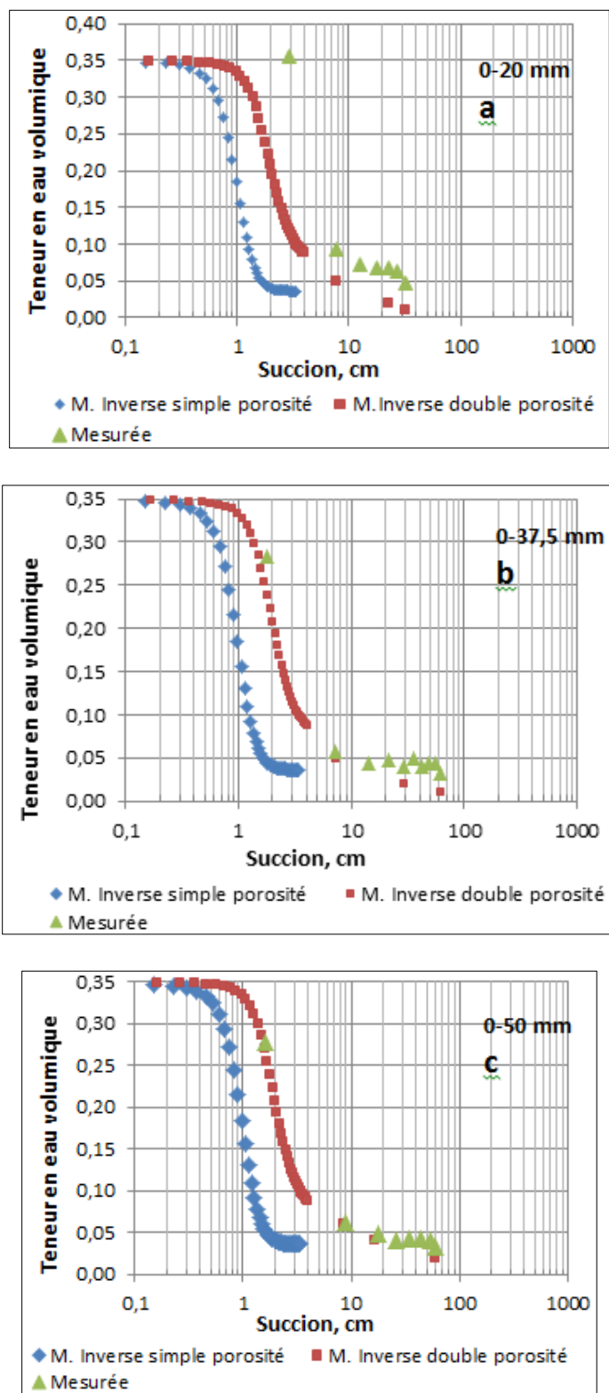
Figures 3-26 : CRE mesurées et obtenues par modélisations inverses; a) stériles 0-20 mm, b) stériles 0-37,5 mm et c) stériles 0-50 mm
