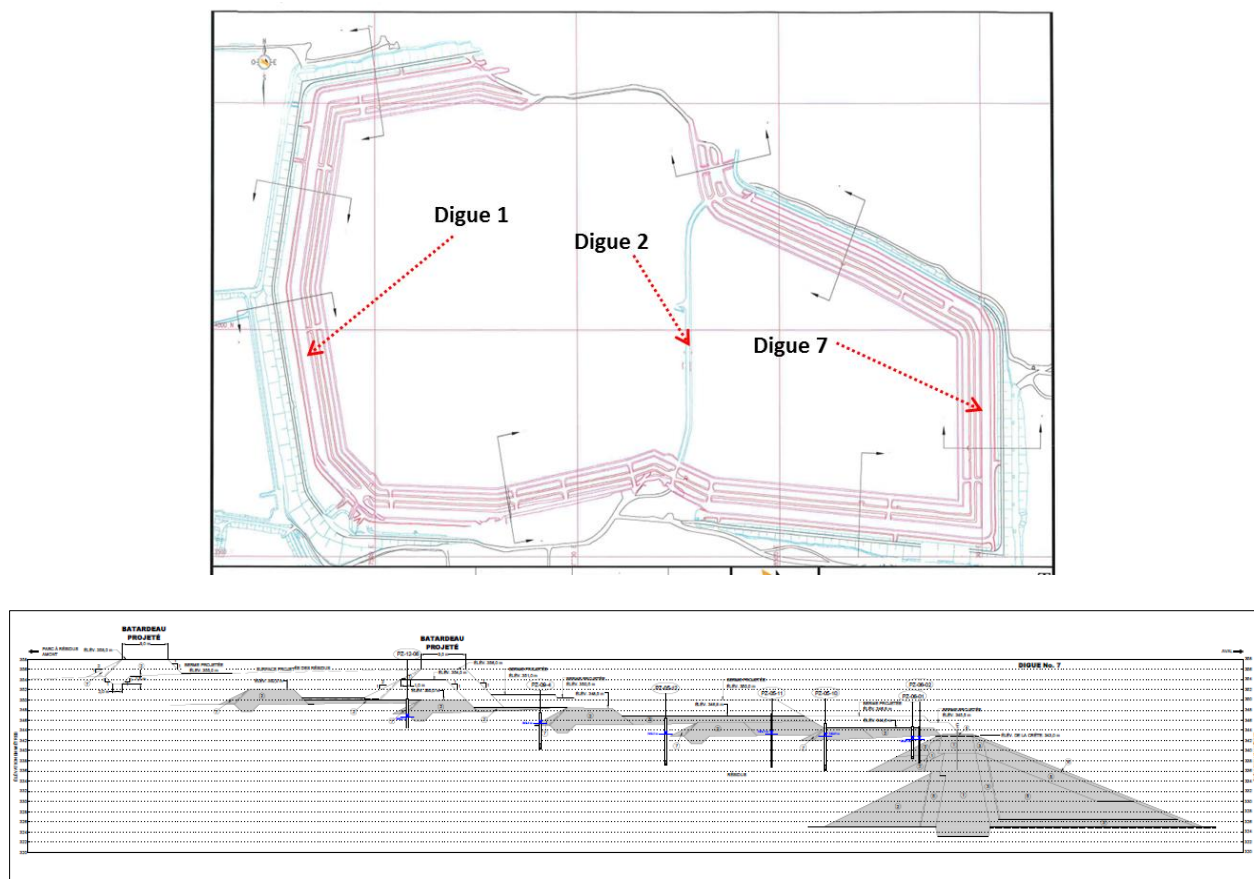
Figure 5-6 : Localisation des différentes digues du parc à résidus LaRonde avec les différents rehaussements amont et vue de la coupe sur la digue 7 (Golder, 2013)
