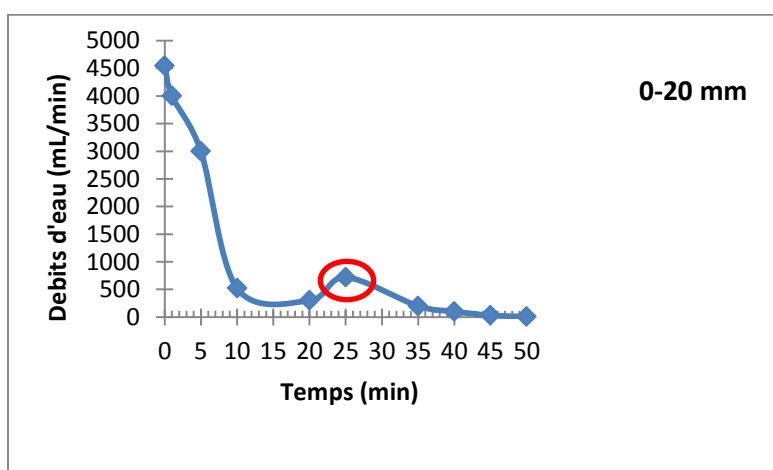
Figures 3-16 : Débits d'eau lors des essais d'infiltration avec identification des phases d'arrivée d'eau (encerclées en rouge)
