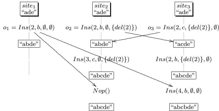
Figure 2.1 Violation de la propriété TP2 par l'algorithme de Suleiman.
