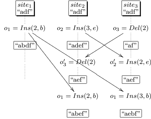
Figure 2.2 Violation de la propriété TP2 par SDT.
