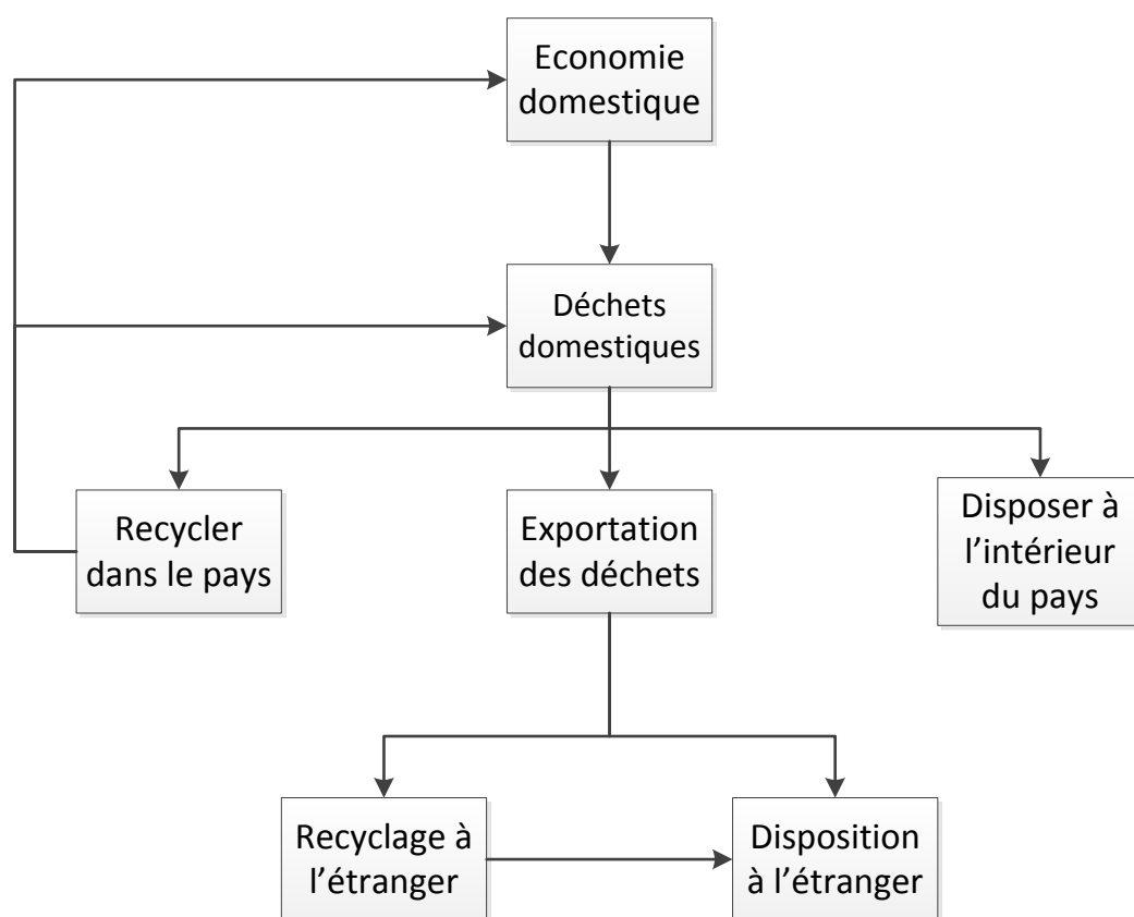
Figure 1-7: Diagramme du commerce des déchets (Kellenberg, 2012)
