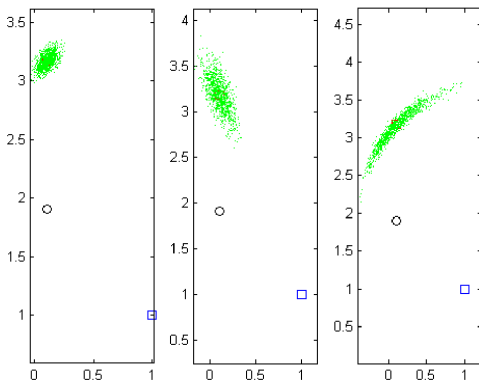
Figure 2.5 Nuage de point de la simulation du mouvement élémentaire d'un robot pour 1000 échantillons avec différents paramètres de bruit (rectangle bleu : pose de départ, rectangle rouge : pose d'arrivée, cercle noir : centre de l'arc du mouvement élémentaire)
