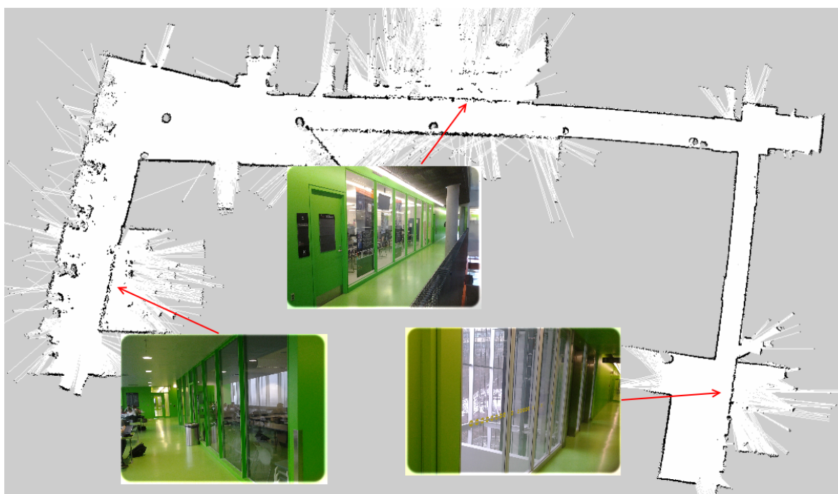
Figure 3.17 Résultat de test à l'étage 5 du pavillon Lassonde : carte-sonar
