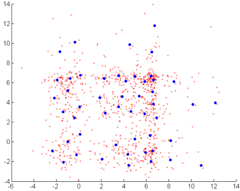
Figure 5.15 Représentation de 50 scénarios (points bleus) obtenus par l'algorithme d'échange des centres représentant 1000 données (croix rouges).
