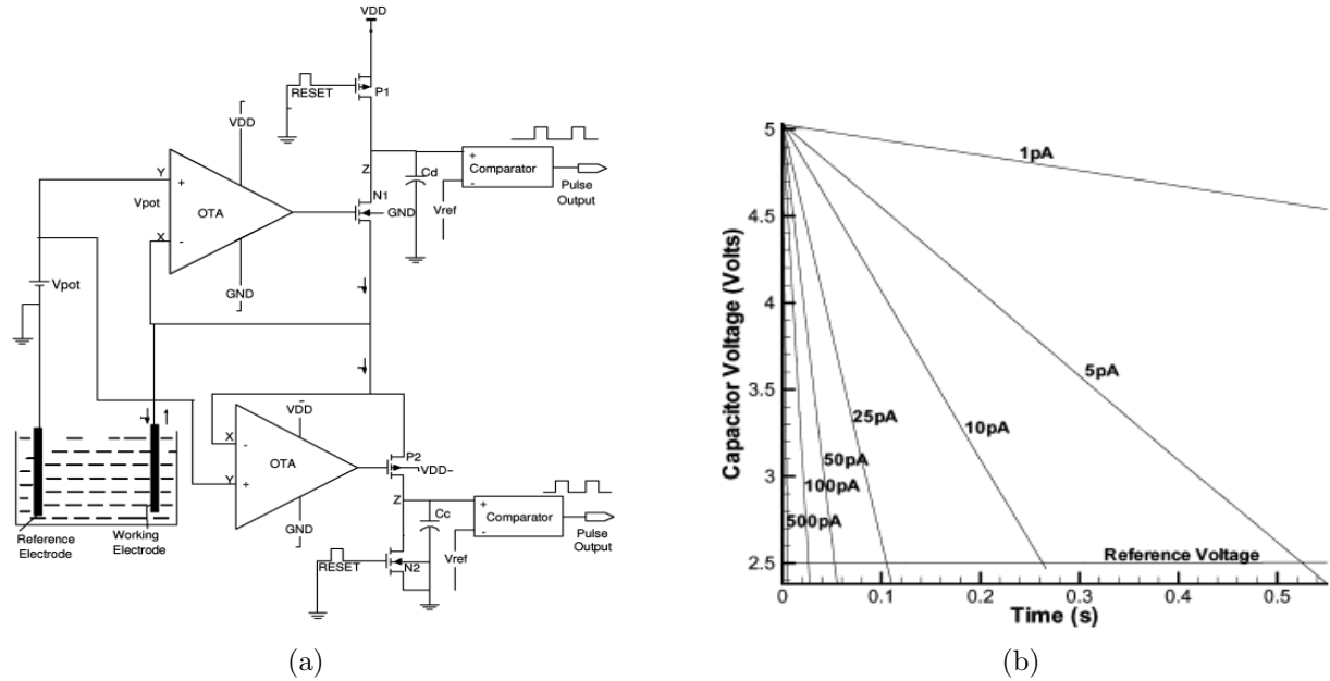
Figure 2.14 Potentiostat proposé par Narula et Harris (2006). (a) Schéma-bloc du circuit. (b) Tension aux bornes de la capacité de mesure versus le temps de décharge qui dépend de l'amplitude du courant d'entrée.
