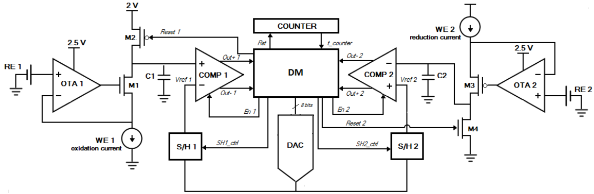
Figure 3.5 Architecture du potentiostat proposé (Massicotte et Sawan (2013)).
