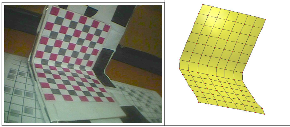
Figure 2.29 à gauche : Objet de calibrage où les points \mathbf{p}_i sont identifiés ; à droite : Modèle 3D de l'objet de calibrage obtenu avec le MicroScribe (numériseur 3D) (voir figure 2.27).
