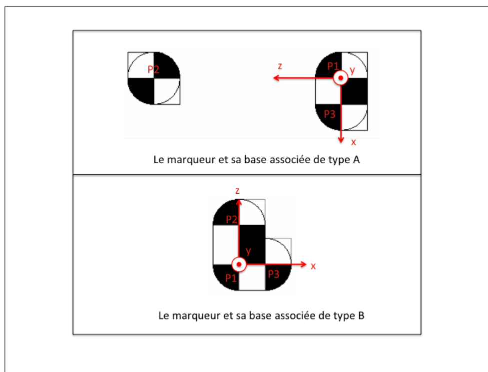
Figure 2.14 Les marqueurs utilisés et leurs bases associées
