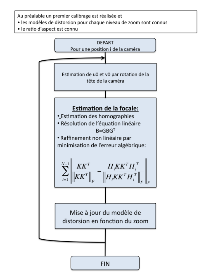
Figure 2.22 Résumé de l'algorithme d'autocalibrage par rotation pure
