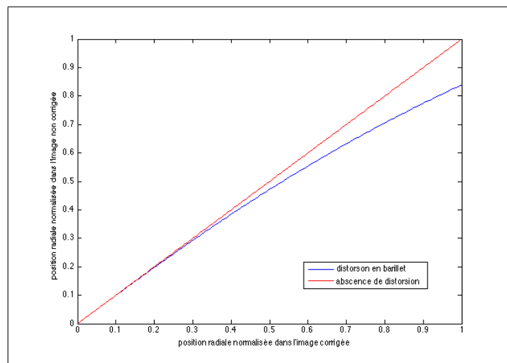
Figure 2.24 Position radiale dans l'image distordue en fonction de la position radiale dans l'image non distordu
