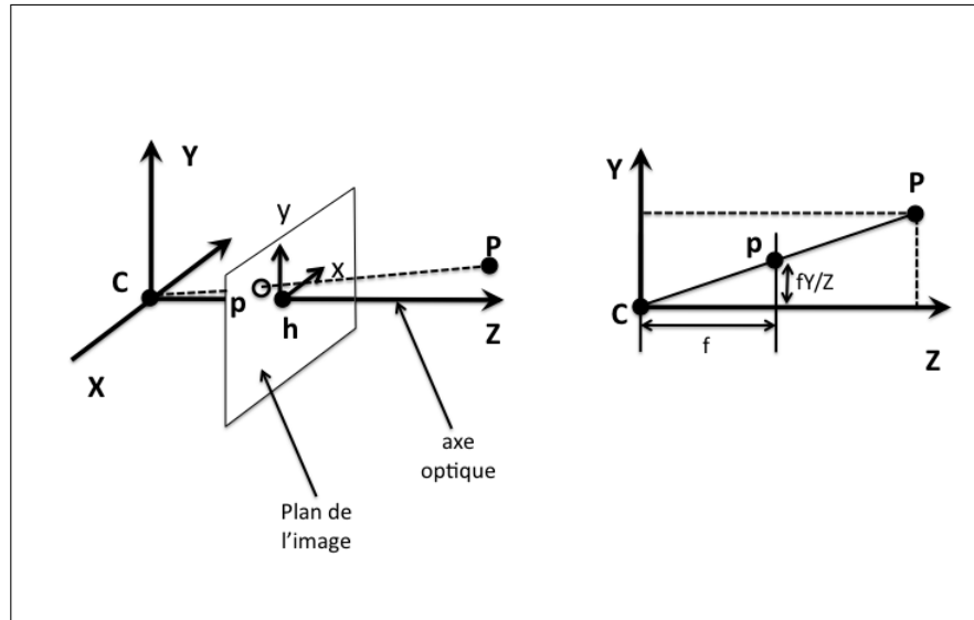
Figure 1.2 Géométrie de la caméra CCD ; h est le point principal
