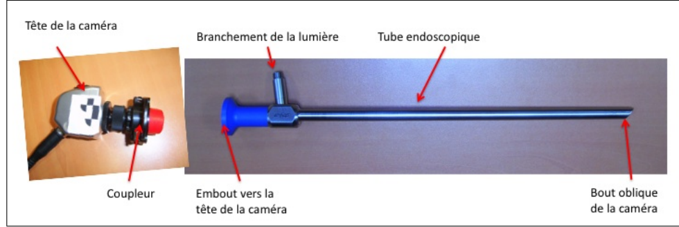
Figure 2.9 La tête de la caméra est reliée à l'endoscope par un coupleur
