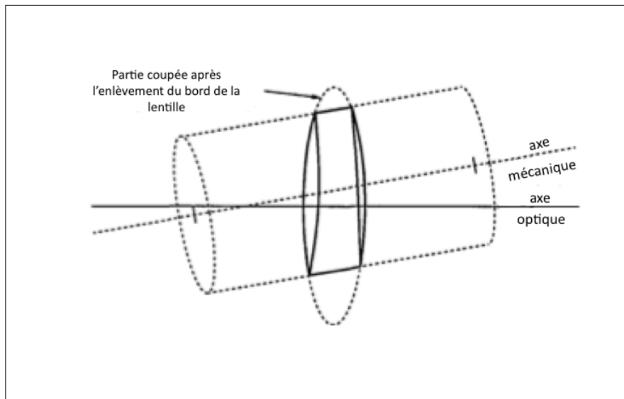
Figure 1.8 L'axe mécanique est différent de l'axe optique (Willson and Shafer, 1994)
