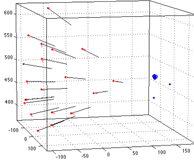
Figure 3.13 Erreur sur l'estimation du bout de l'instrument
