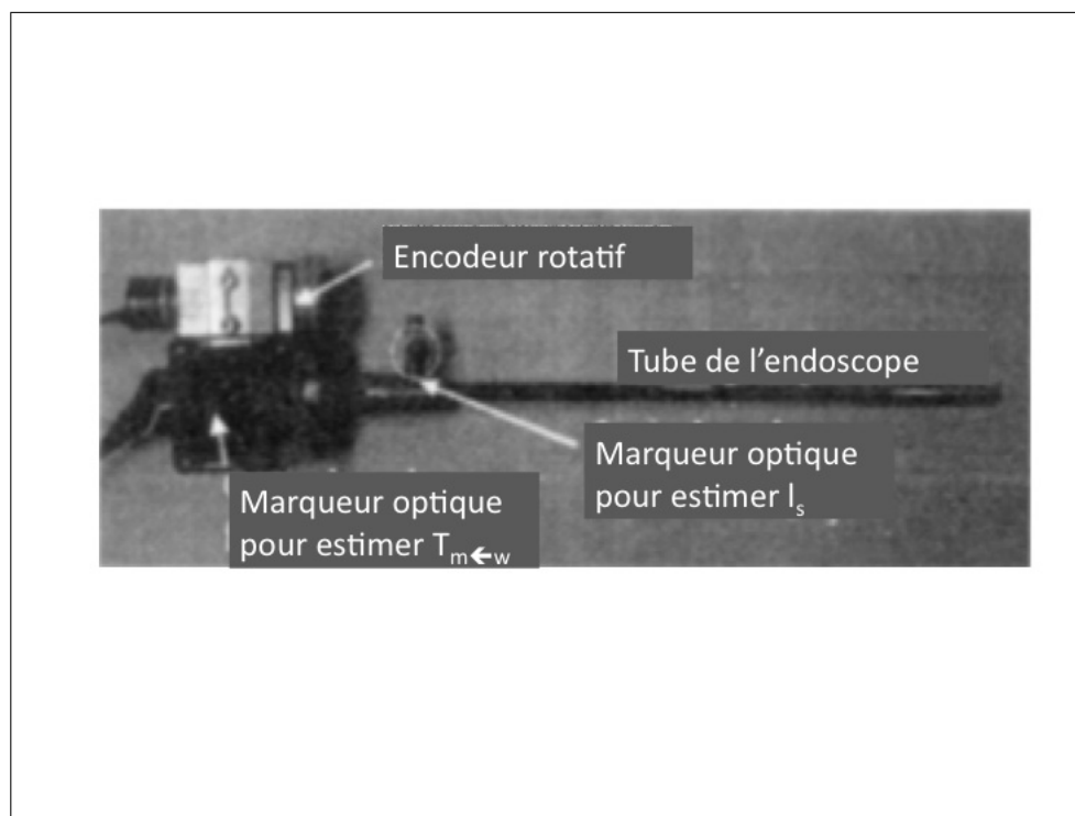
Figure 1.27 Caméra et tube endoscopique et placement du marqueur et de l'encodeur rotatif (Yamaguchi et al., 2005)
