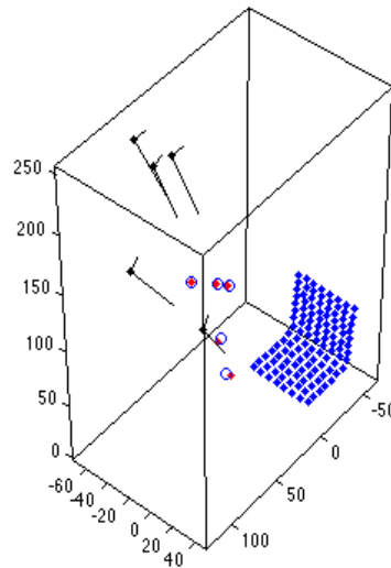
Figure 3.11 Configuration d'un calibrage manuel (en noir les marqueurs du MicronTracker, en point rouge les positions de caméra du calibrage manuel et en rond bleu les positions de caméra du suivi de mouvement)
