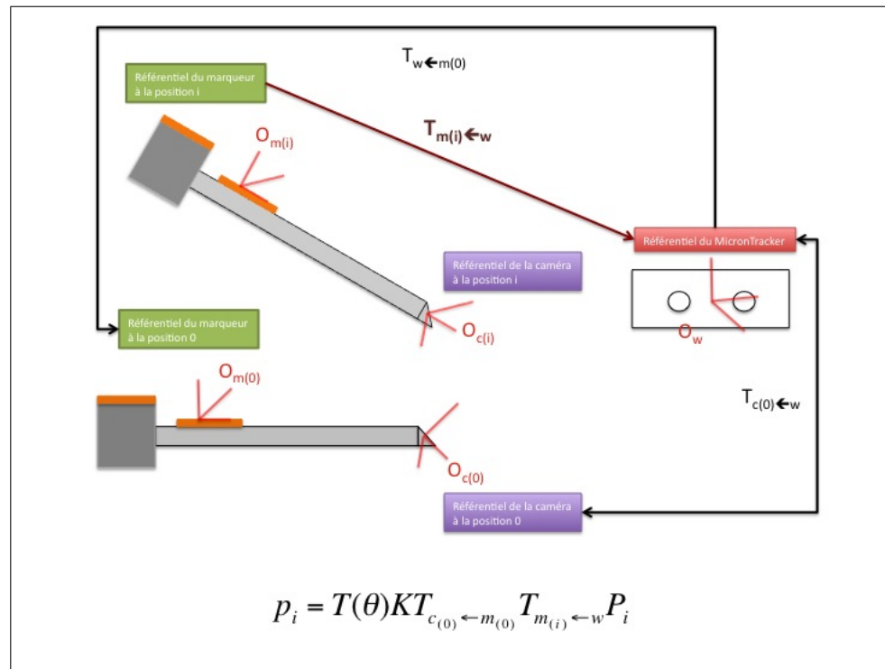
Figure 2.16 Modèle du suivi de mouvement
