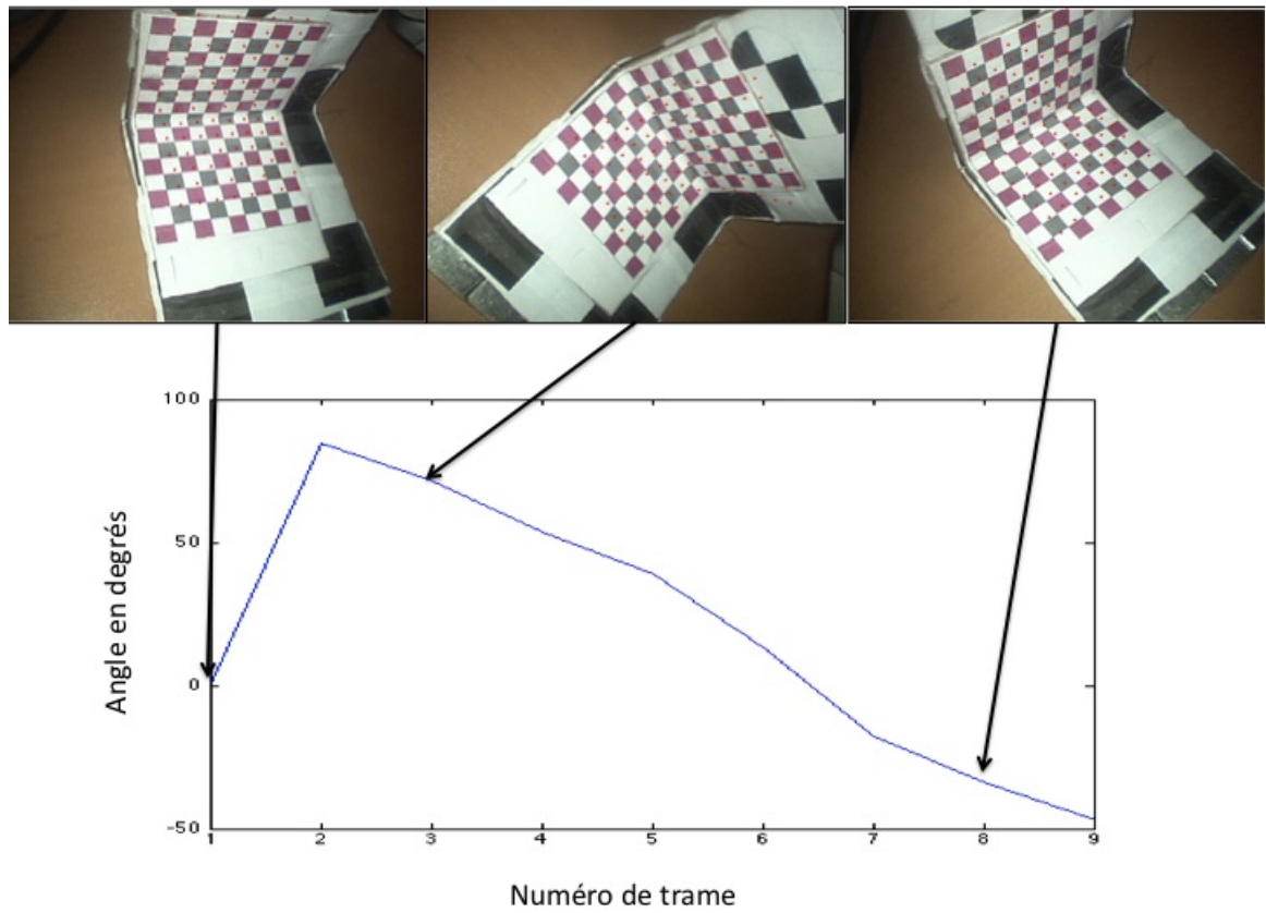
Figure 3.15 Estimation de la rotation entre la caméra et l'endoscope
