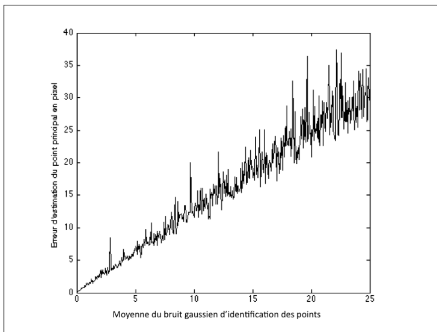
Figure 3.4 Erreur d'identification du point principal en fonction du bruit d'identification des points
