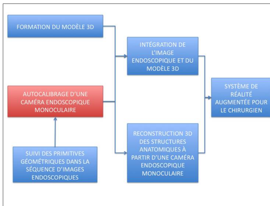
Figure 3 L'autocalibrage dans le projet
