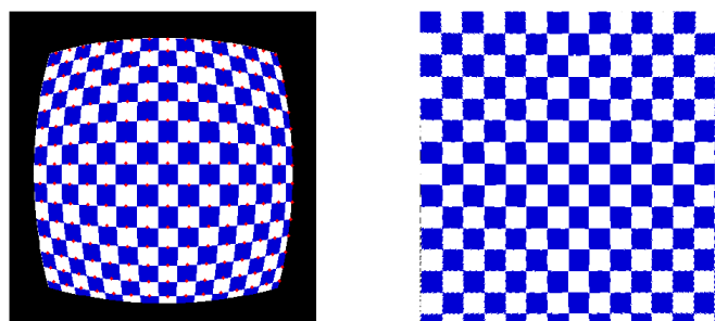
Figure 3.1 à gauche : image simulée ; à droite : image corrigée
