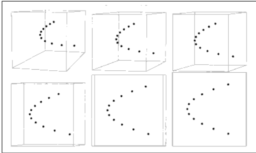
Figure 1.10 Représentation d'une cubique twistée pour plusieurs vues (Hartley and Zisserman, 2002)
