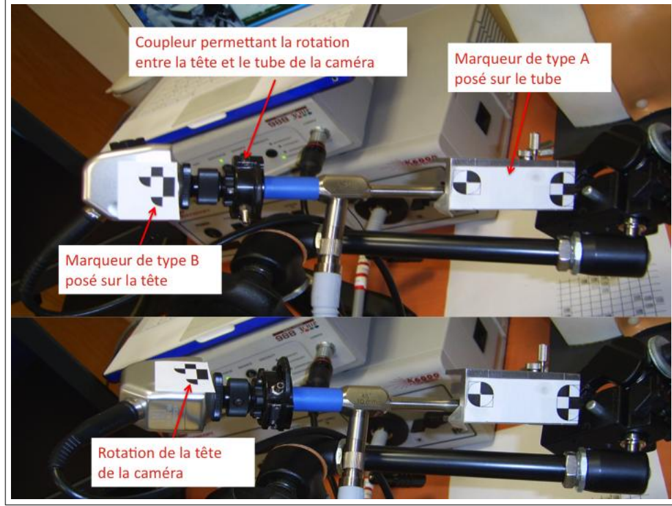
Figure 2.15 Placement des marqueurs sur la caméra endoscopique
