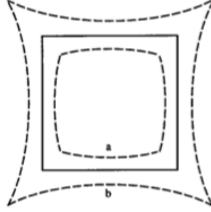
Figure 1.6 Effet de la distorsion radiale : a) distorsion avec k_1 négatif dit en barillet b) distorsion avec k_1 positif dit en croissant
