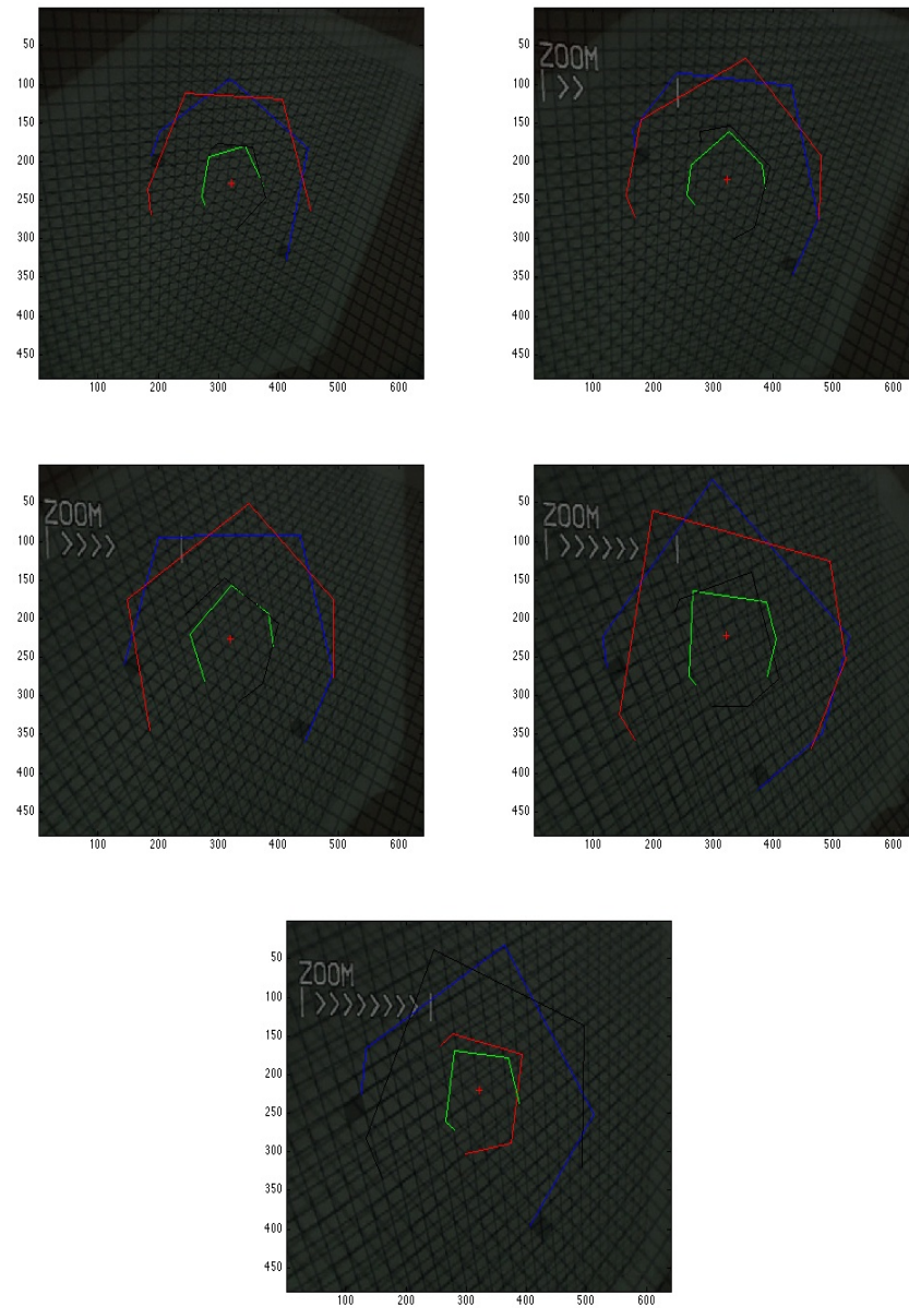
Figure 3.6 Estimation du point principal pour différents zooms
