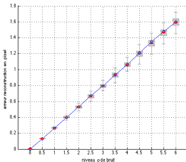
Figure 3.10 Erreur sur l'estimation de l'erreur de reprojection en fonction du bruit
