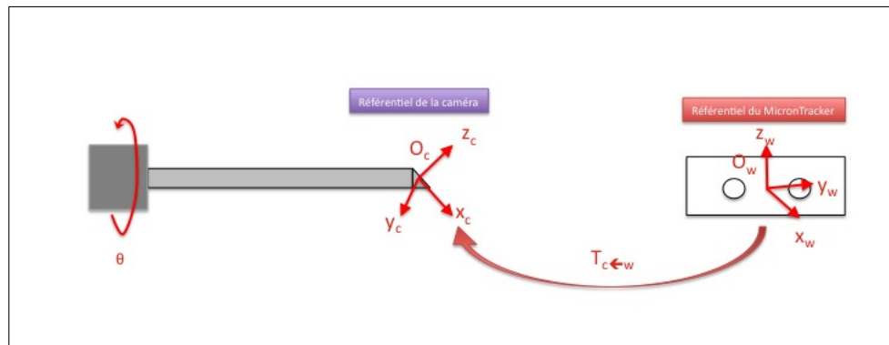
Figure 2.11 Les deux bases des référentiels du monde w et de la caméra c
