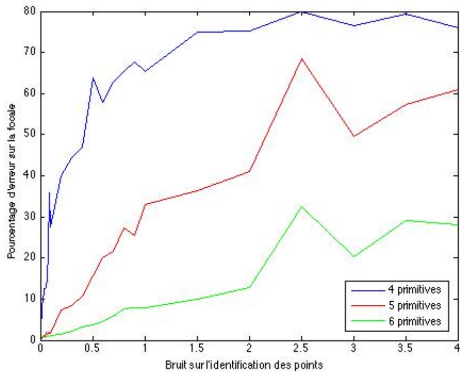
Figure 3.19 Erreur d'estimation de la focale en fonction du bruit sur l'identification des primitives
