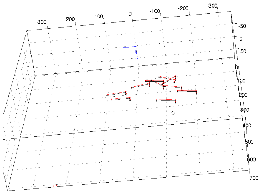
Figure 3.12 Comparaison entre la numérisation 3D du Microntracker et du Microscribe ; le rond est le centre de la caméra stéréoscopique du Microntracker
