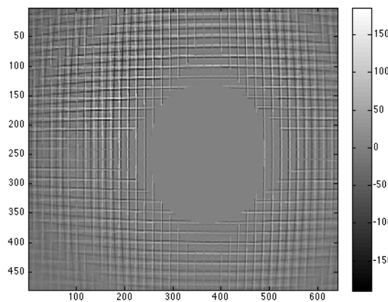
Figure 2.2 Différence entre l'image distordue et l'image non distordue ; l'erreur est de 0 au centre de distorsion
