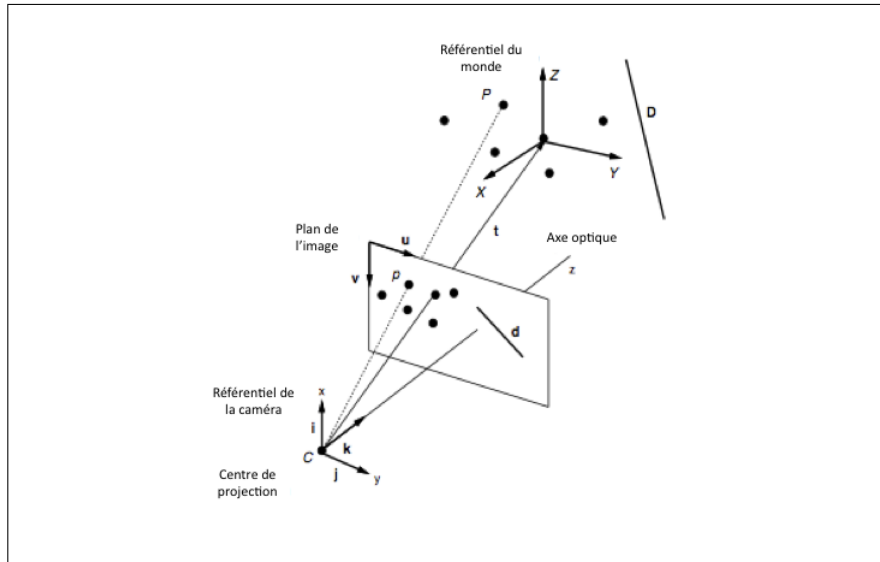
Figure 1.1 Modèle linéaire de la caméra
