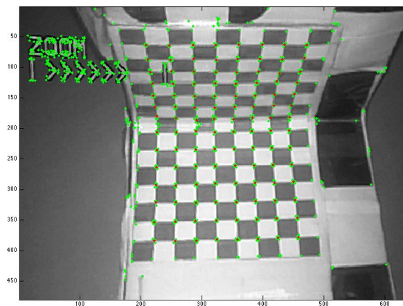
Figure D.2 Détection des points de la grille après identification des coins dans l'image
