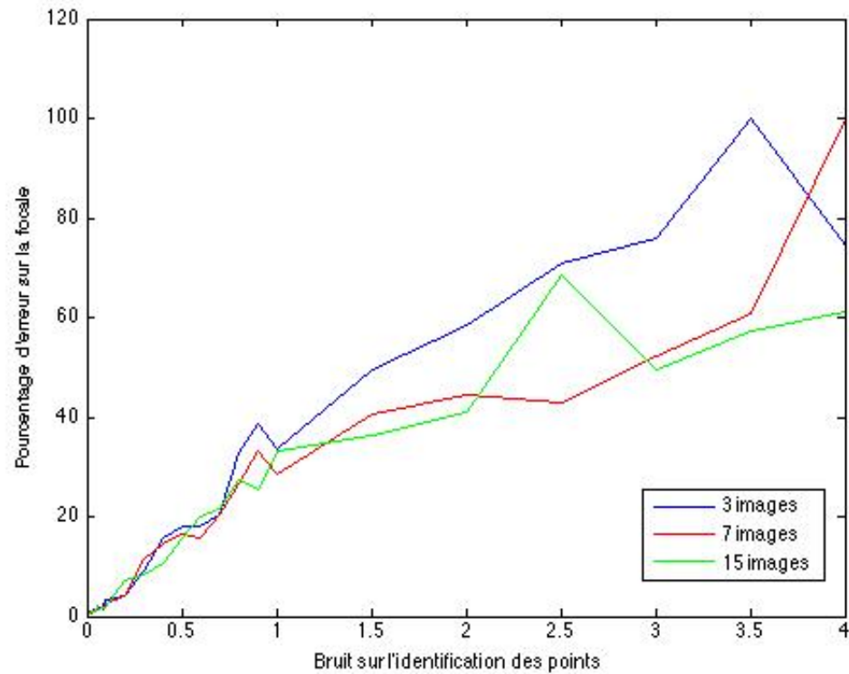
Figure 3.20 Erreur d'estimation de la focale en fonction du bruit sur l'identification des primitives
