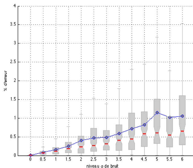
Figure 3.7 Erreur sur l'estimation de la focale en fonction du bruit
