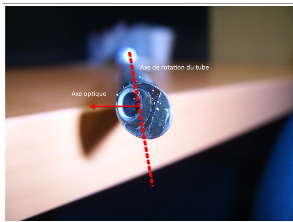
Figure 2.10 les deux axes de rotation lors de la rotation du tube alors que la tête de la caméra est fixe
