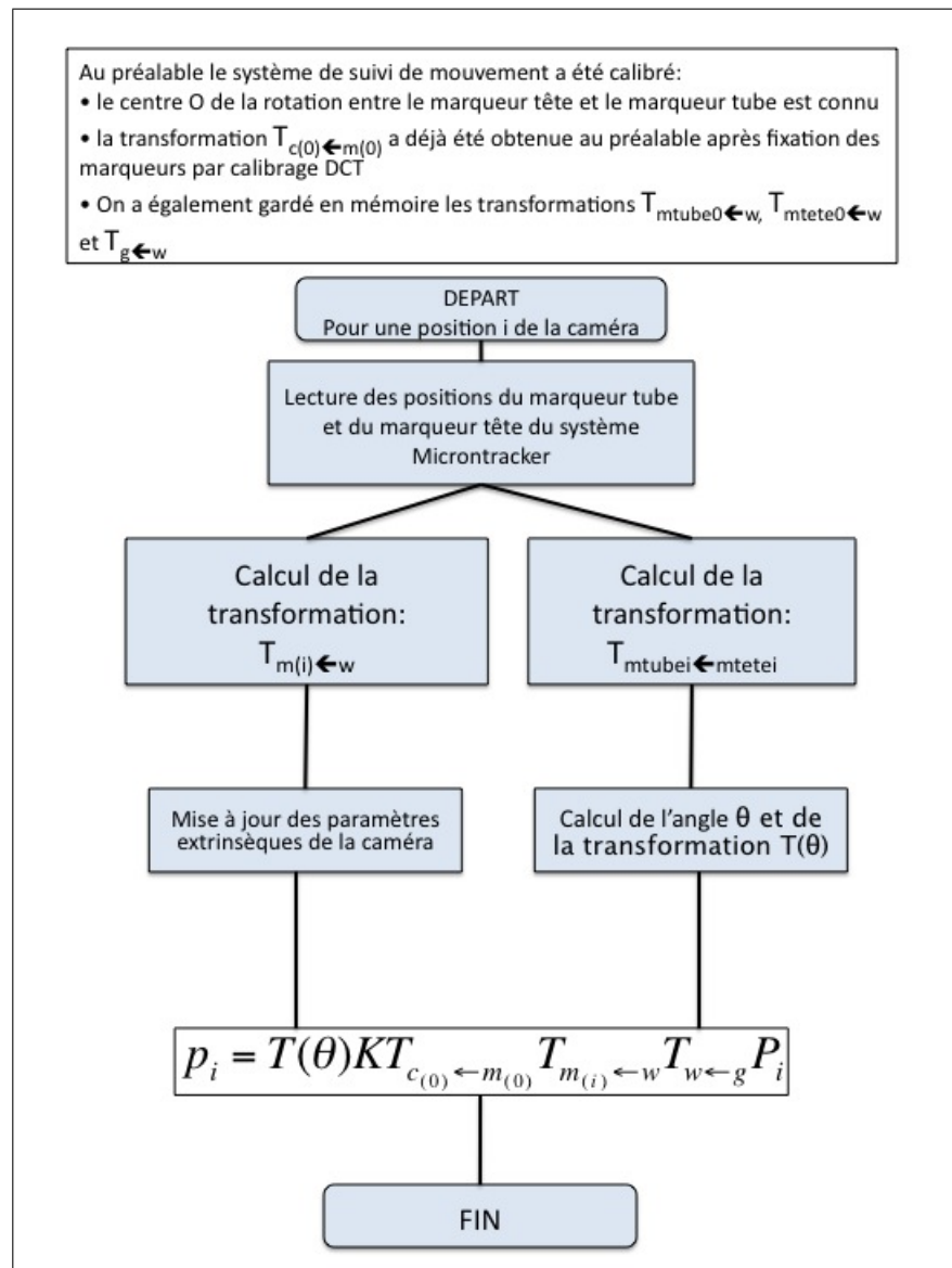
Figure 2.18 Étapes de l'algorithme de suivi de mouvement
