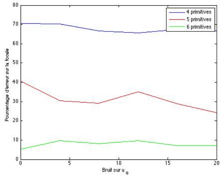
Figure 3.21 Erreur d'estimation de la focale en fonction du bruit sur l'identification des primitives
