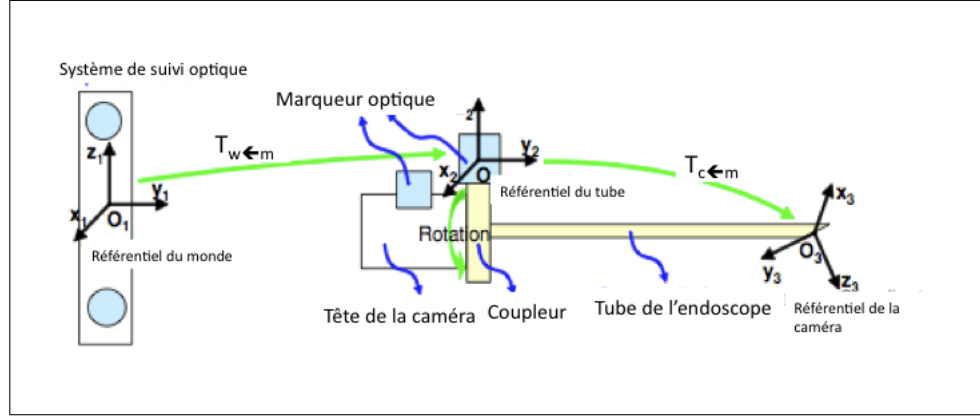
Figure 1.28 Caméra et tube endoscopique et placement des marqueurs selon Wu (Wu and Jaramaz, 2008)
