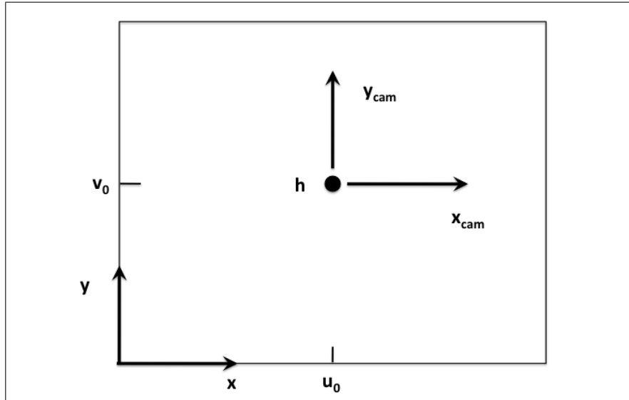
Figure 1.3 Référentiel de l'image et de la caméra ; \mathbf{h}(u_0, v_0) est le point principal
