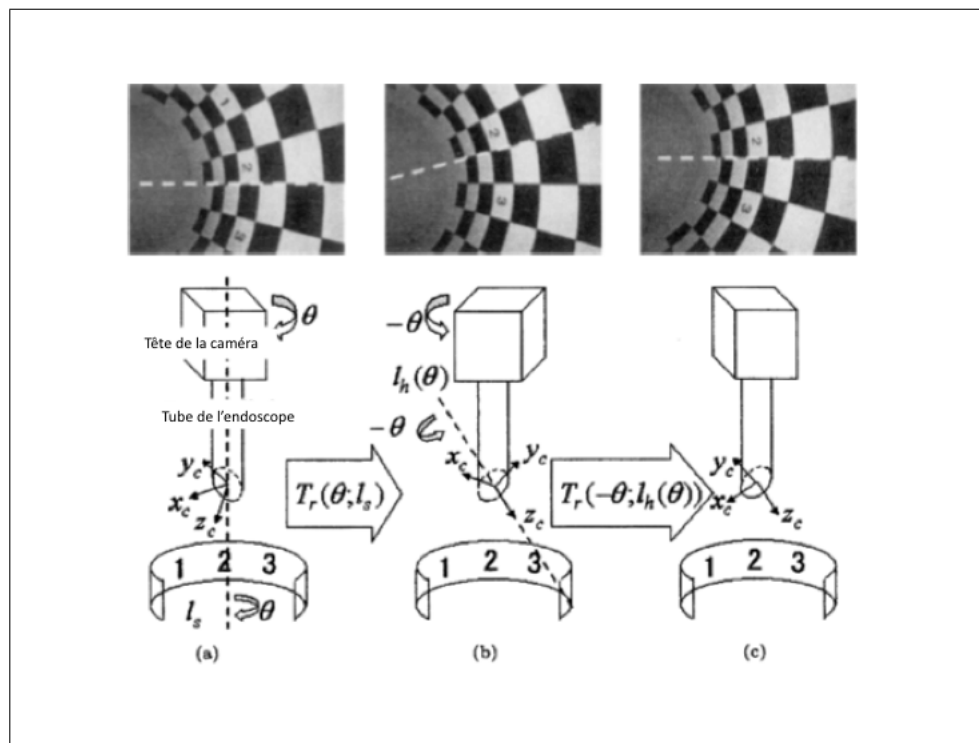
Figure 1.26 Schéma du modèle de projection pour les endoscopes à vision oblique
