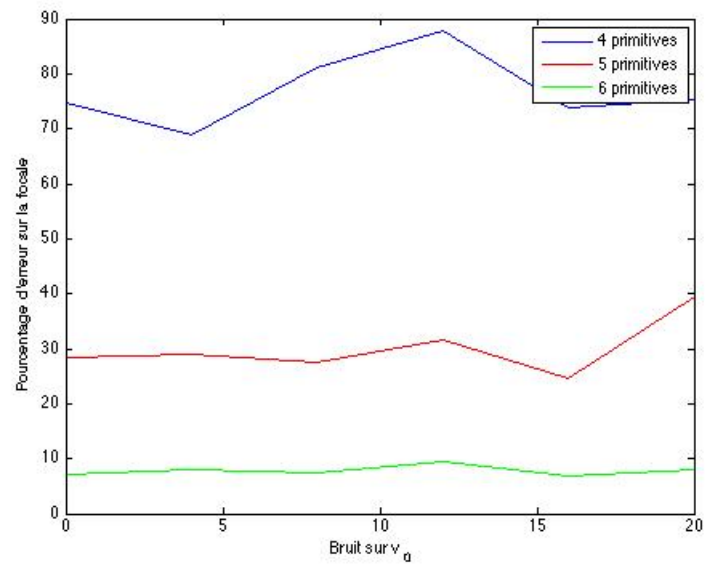
Figure 3.22 Erreur d'estimation de la focale en fonction du bruit sur l'identification des primitives
