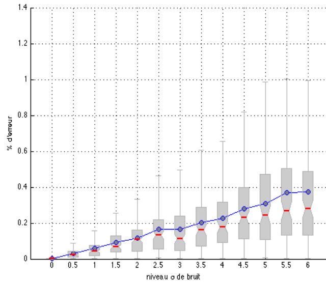
Figure 3.8 Erreur sur l'estimation de \alpha en fonction du bruit
