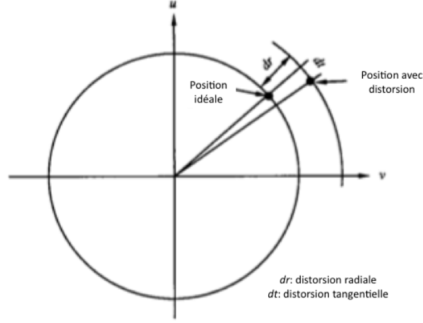
Figure 1.5 Distorsion radiale et tangentielle
