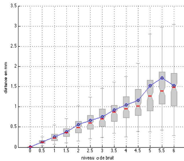
Figure 3.9 Erreur sur l'estimation de la position en fonction du bruit
