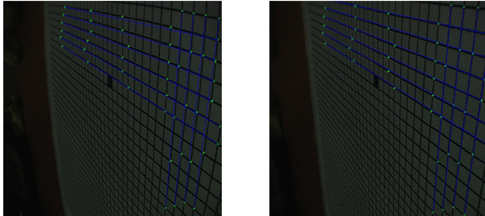
Figure 3.3 à gauche : image et lignes avec distorsion ; à droite : image et lignes sans distorsion
