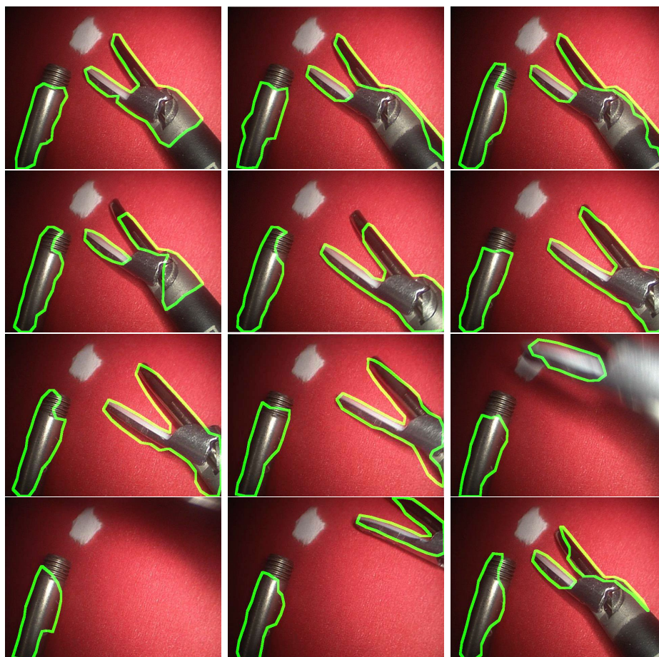
Figure A.21 Résultat sur la séquence en environnement contrôlé
