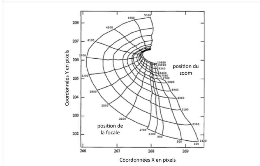
Figure 1.7 Variation du point principal en fonction de la focale et du zoom (Willson and Shafer, 1994)
