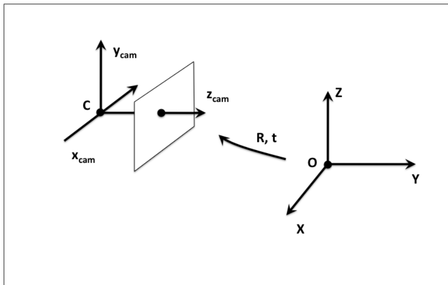
Figure 1.4 La transformation rigide entre le référentiel monde et le référentiel de la caméra
