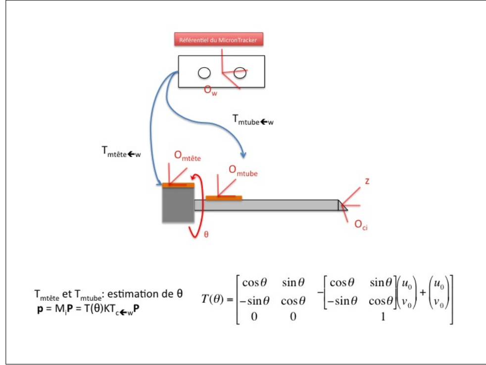
Figure 2.17 Modèle de rotation de la tête de la caméra
