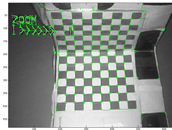
Figure D.1 Détection des coins après algorithme de Rosten (Rosten and Drummond, 2005)
