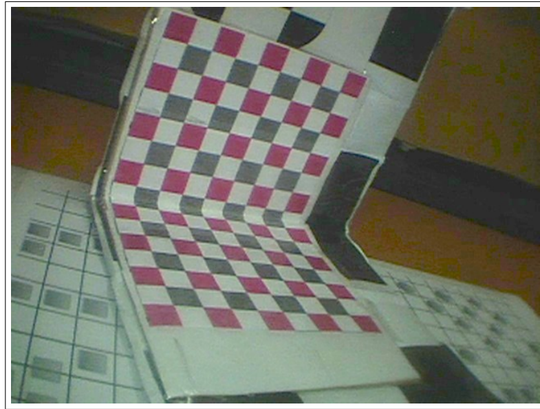
Figure 2.8 Objet de calibrage utilisé pour le calibrage DLT
