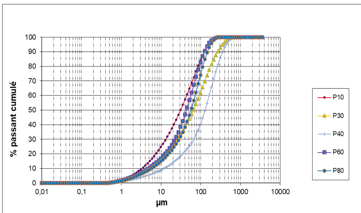
Figure D.6 Courbes granulométriques de profil : station H5
