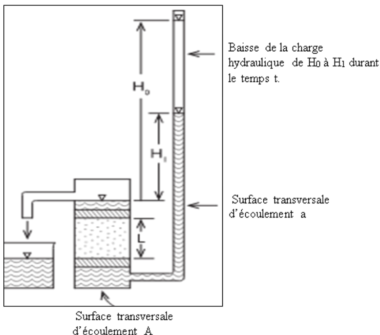
Figure 3.9 Mesure de la k_{sat} au perméamètre à charge variable descendante (Todd, 1959)
