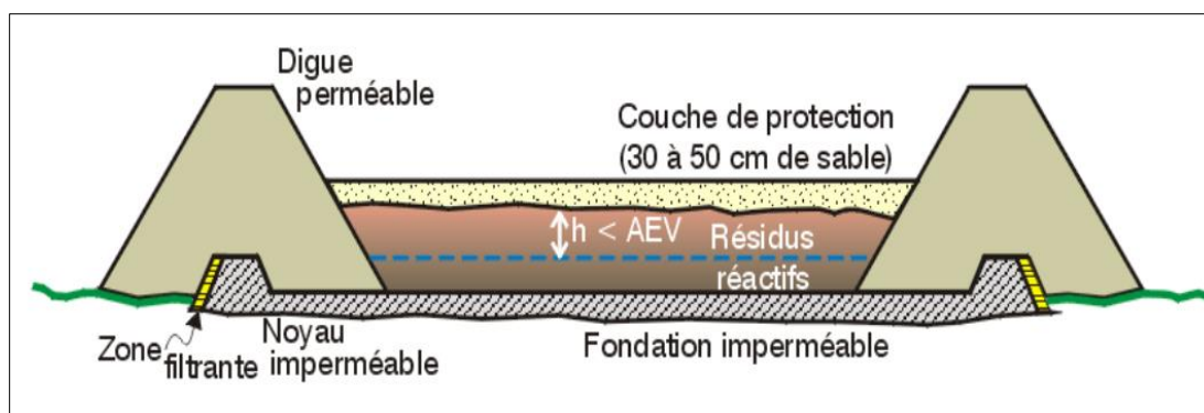
Figure 2.2: Modèle conceptuel d'une nappe phréatique surélevée dans les résidus réactifs pour réduire le drainage minier acide (adapté d'Aubertin et al., 1999).
