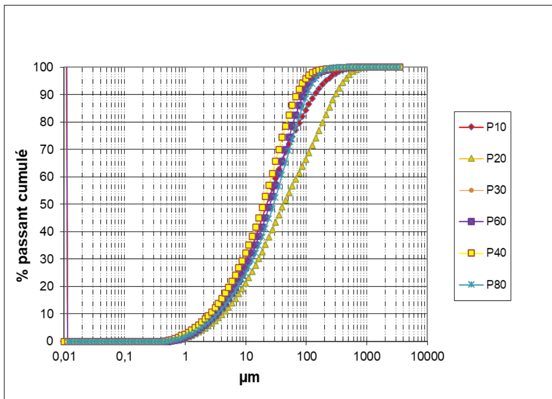
Figure D.14 Courbes granulométriques de profil : station SH17
