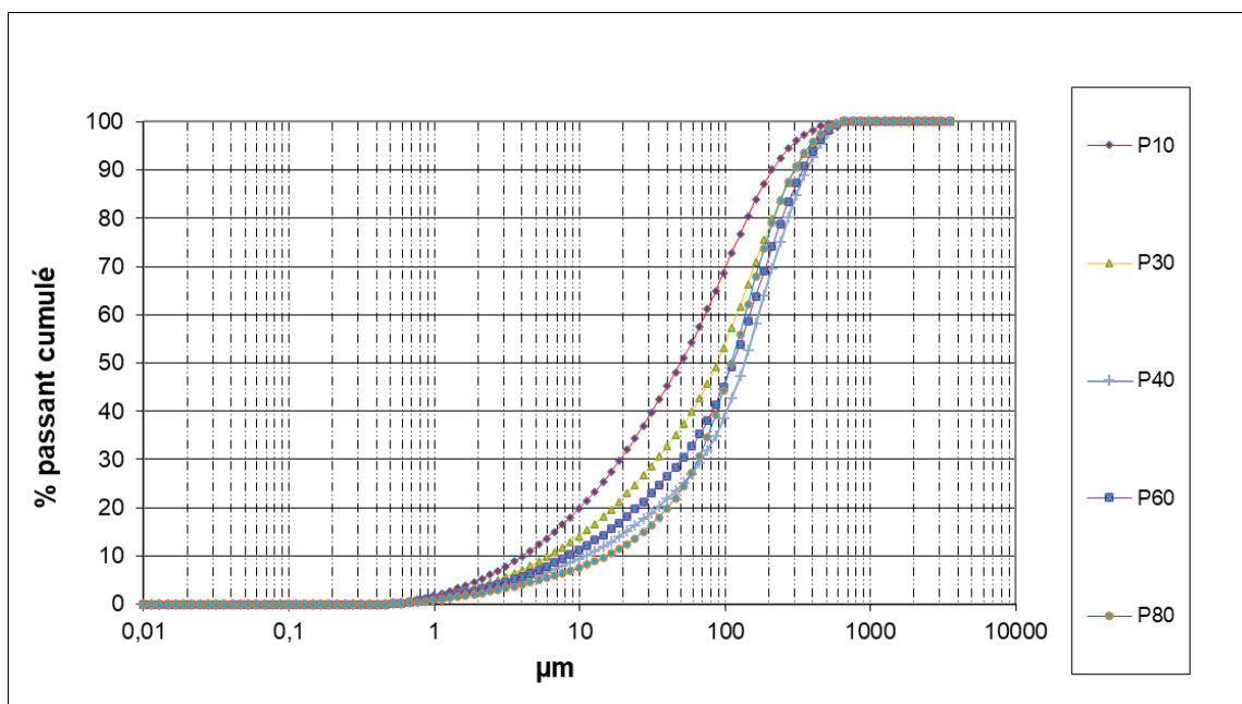
Figure D.3 Courbes granulométriques de profil : station H2
