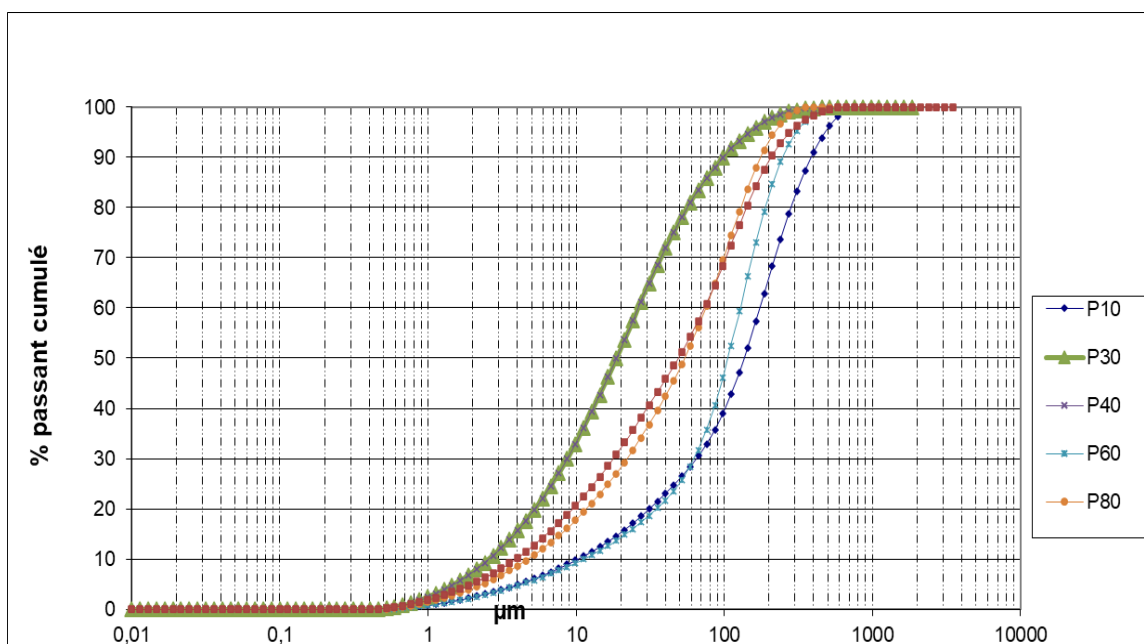
Figure D.16 Courbes granulométriques de profil : station TSV21
