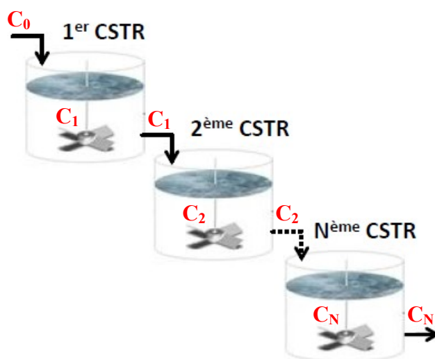
Figure 1-2: Fonctionnement du modèle N-CSTR
