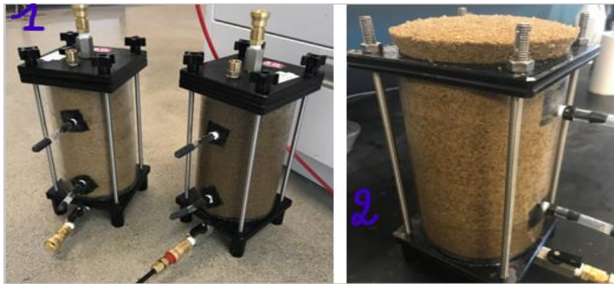
Figure 3.3-6 : Photos illustrant : (1) la phase de saturation du mélange sable et PSA dans le perméamètre à parois rigides; et (2) le gonflement du matériau après saturation complète.
