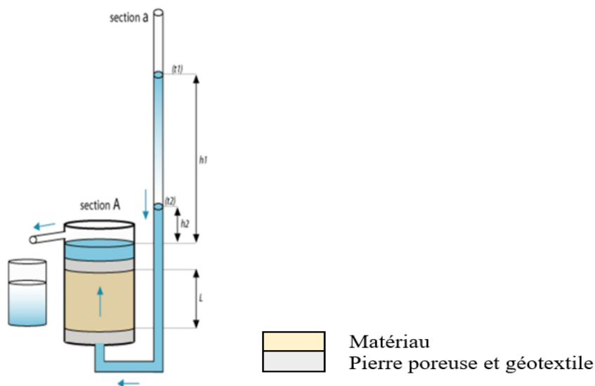
Figure 3.3-7: Schéma d'un perméamètre à parois rigide
