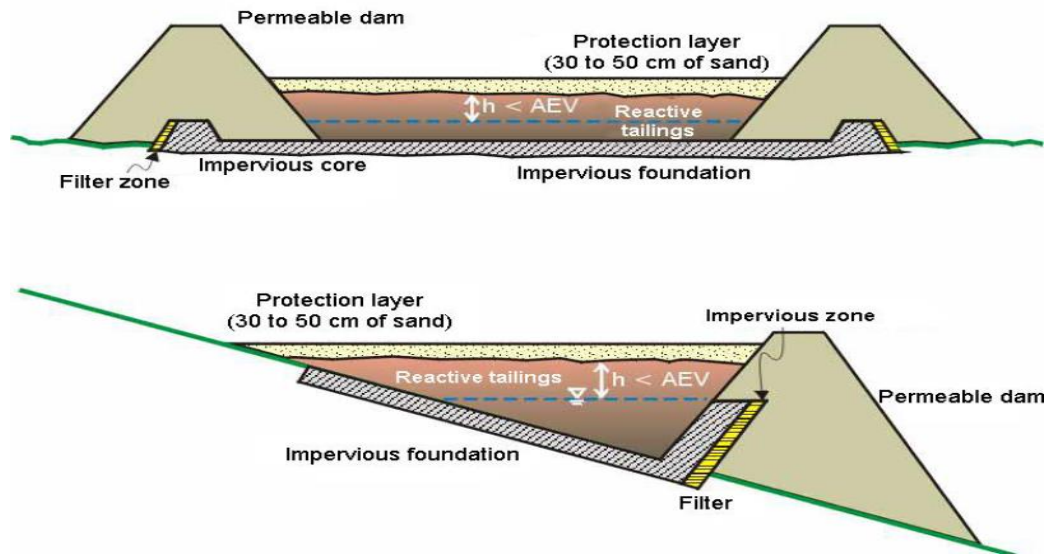
Figure 2.2-1: Modèles conceptuels de la nappe phréatique surélevée dans des résidus réactifs pour contrôler la génération du DMA (Aubertin et al. , 1999)
