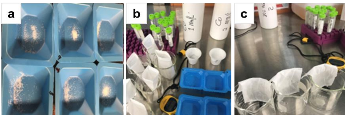
Figure 3.3-5: Étapes des essais d'adsorption de métaux par les PSA : a) PSA secs, b) processus d'adsorption après ajout de la solution métallique synthétique et c) séparation des PSA contenus dans un sachet de thé de la solution résiduelle sans y appliquer une pression.
