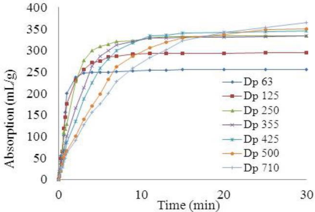
Figure 2.3-2 : Capacité d'absorption des grains de PSA de différents diamètres ( D_p ) (d'après Casquilho et al. , 2013)
