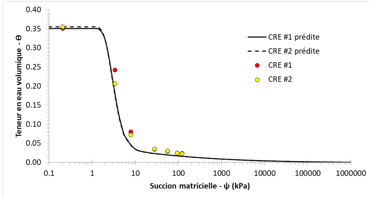
Figure 4.2-2 : Courbe de rétention d'eau du sable utilisé (matériau témoin)
