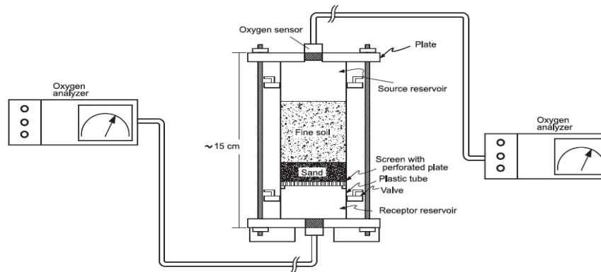
Figure 2.5-1 : Appareil à deux chambres pour la détermination expérimentale de D_e (tiré de Mbonimpa et al. , 2003).
