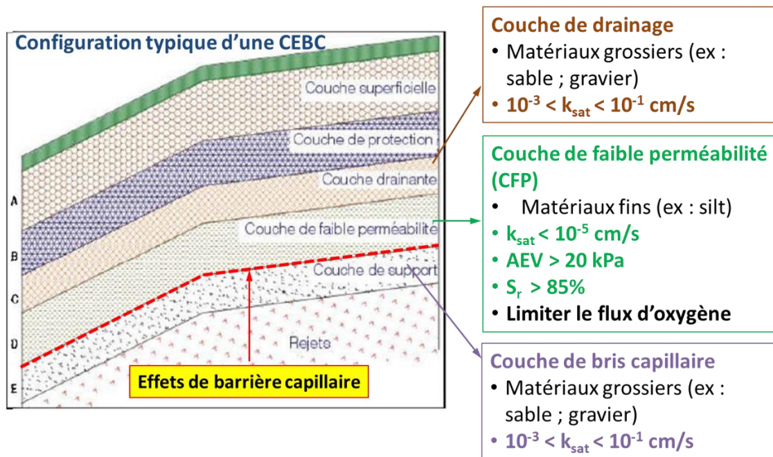
Figure 2.2-2 : Configuration typique d'un système de recouvrement multicouche CEBC (adapté de Aubertin et al. , 1999)
