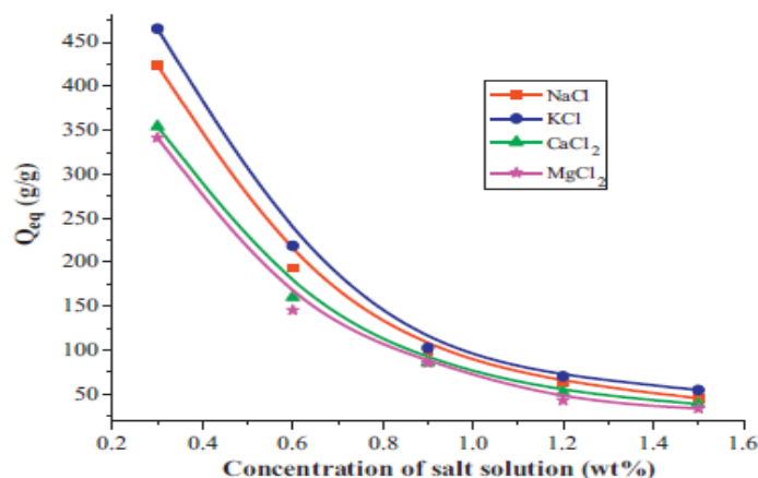
Figure 2.3-8 : Capacité d'absorption d'eau d'un hydrogel superabsorbant dans des solutions aqueuses de NaCl, KCl, CaCl 2 et MgCl 2 (d'après Bao et al. , 2011).
