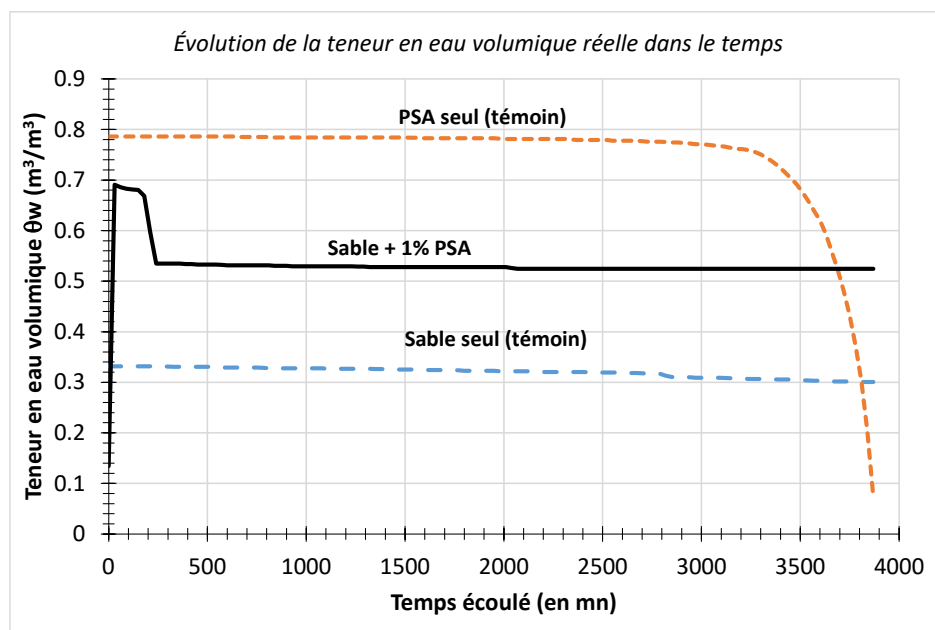
Figure 3.2-4 : Évolution de la teneur en eau volumique des matériaux de base (PSA et Sable) comparée du mélange de 1% de PSA avec le sable
