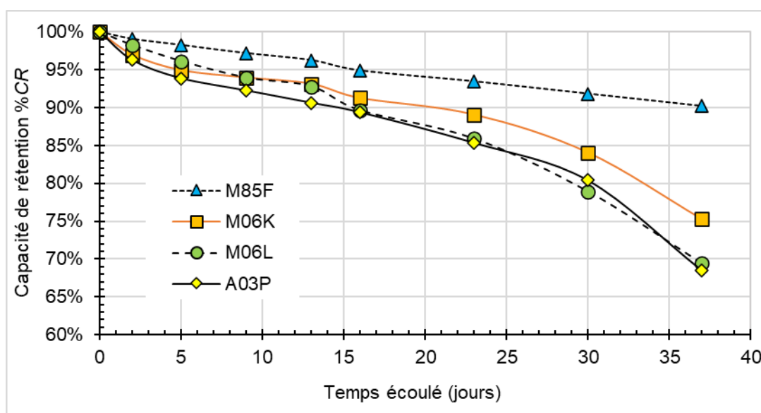
Figure 4.1-2 : Capacité de rétention de l'eau des PSA en fonction du temps écoulé
