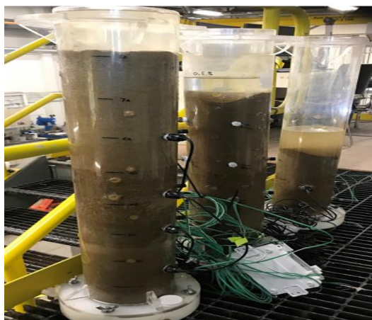
Figure 4.3-3 : Photo des colonnes instrumentées
