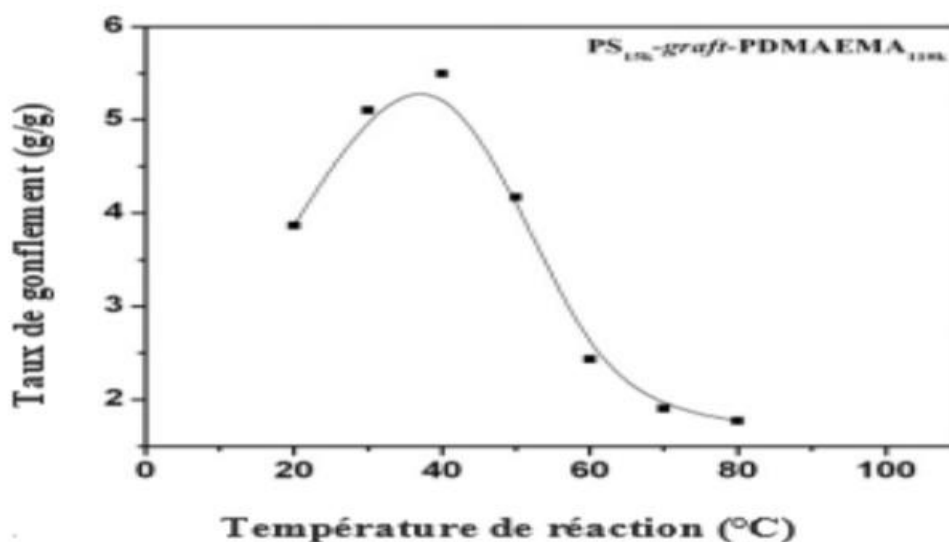
Figure 2.3-5 : Dépendance du taux de gonflement ( Q_{eq} ) dans l'eau en fonction de la température (d'après Vivek et al. , 2008)
