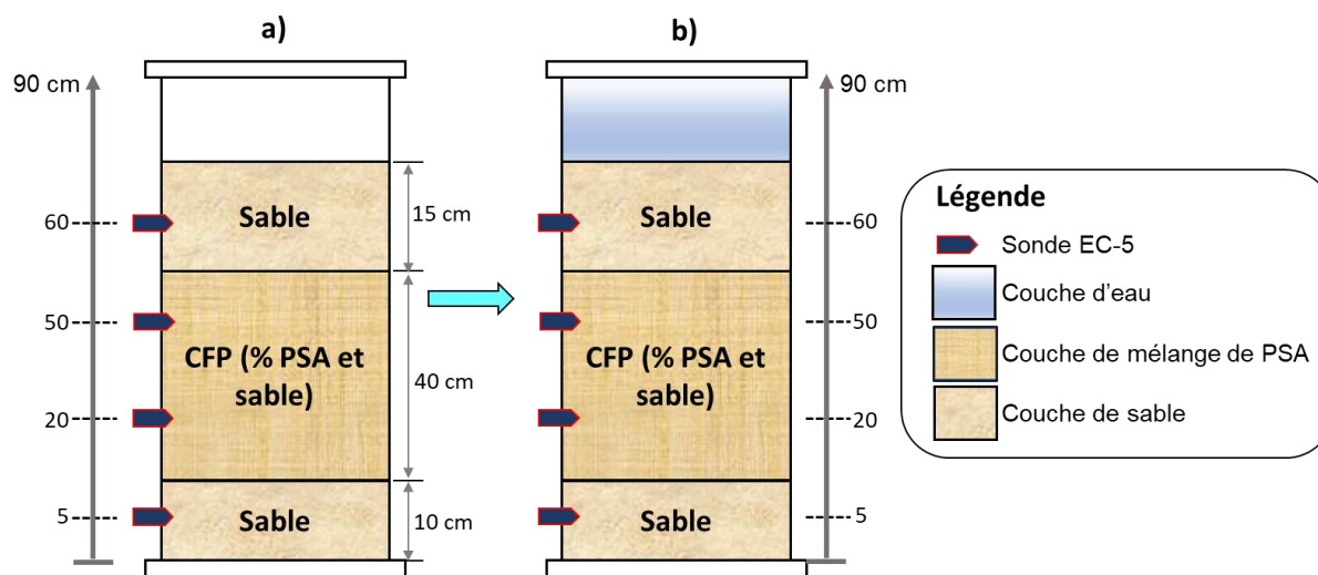
Figure 3.3-13 : Schéma de la colonne de CFP qui est un mélange sable et de 0,7% et 1% de PSA
