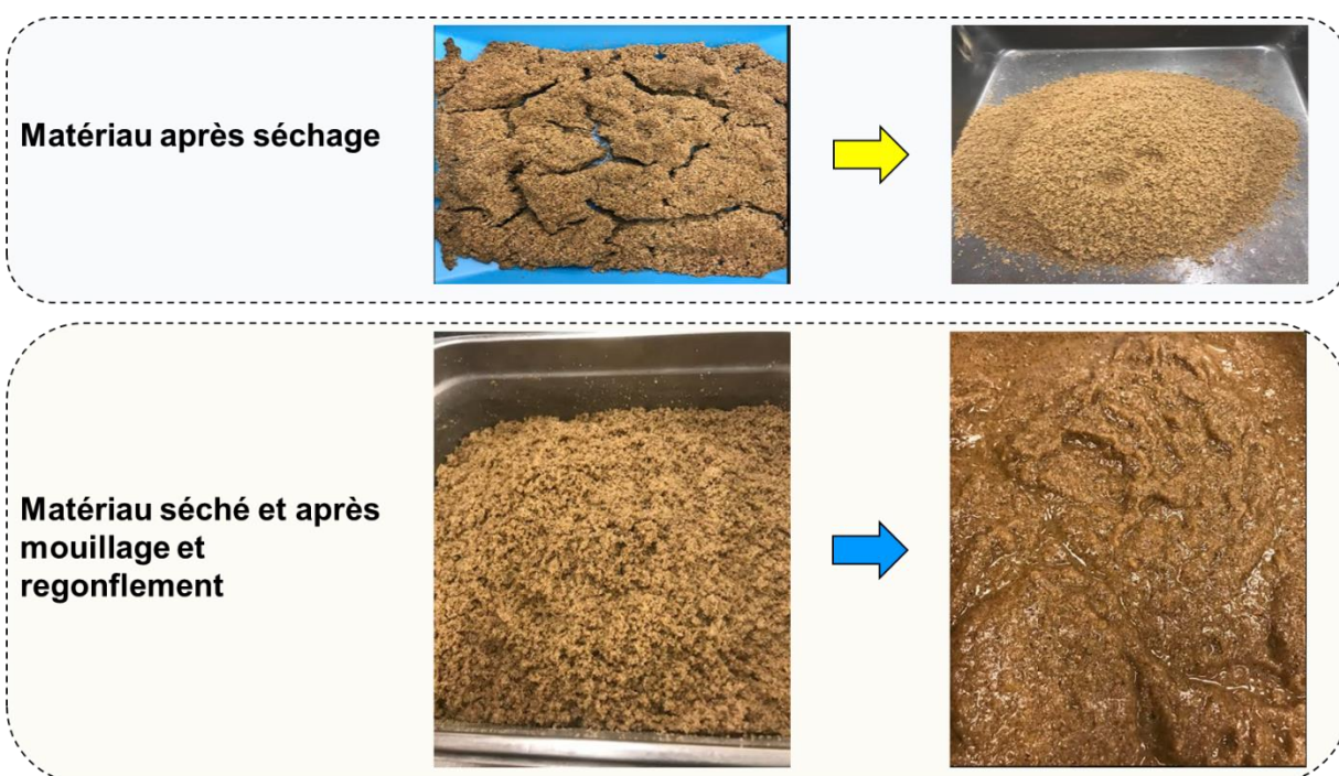
Figure 4.2-1 : Mélange de sable et 0,7% de PSA-M85F après séchage à l'étuve à 60°C pendant 3 jours et regonflement après rinçage/mouillage
