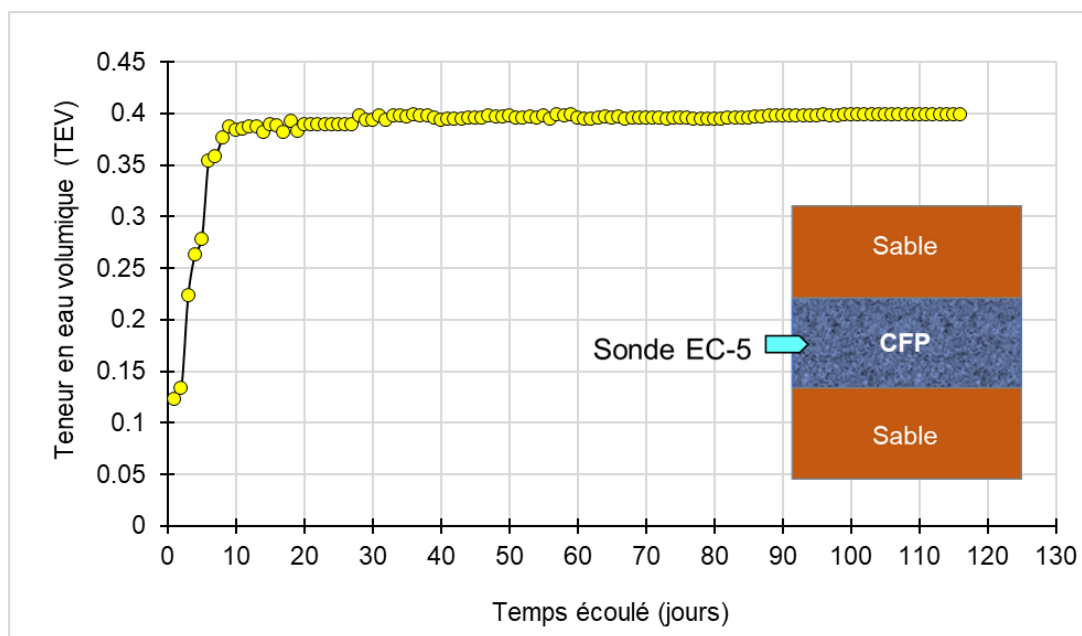
Figure 4.2-7 : Évolution de la teneur en eau volumique de la CFP faite de sable et 0,7% PSA
