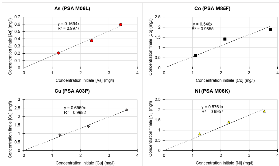
Figure 4.1-7 : Équations de régressions linéaires entre les concentrations finales [C_f] et initiales [C_i] pour les trois métaux (Co, Cu, Ni) et le métalloïde (As) testés
