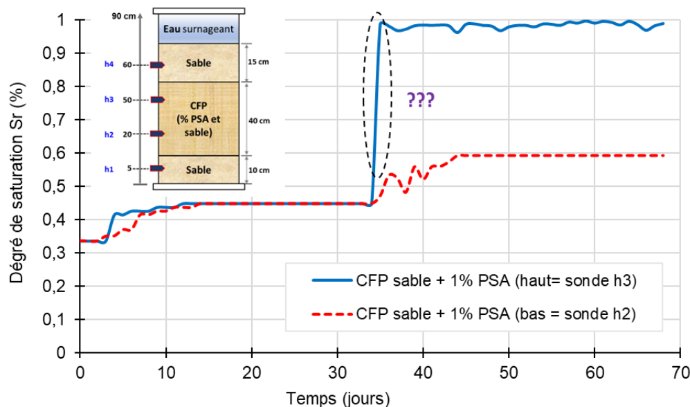
Figure 4.3-2 : Évolution du degré de saturation de la CFP faite de sable avec 1% PSA en fonction du temps écoulé (jours)
