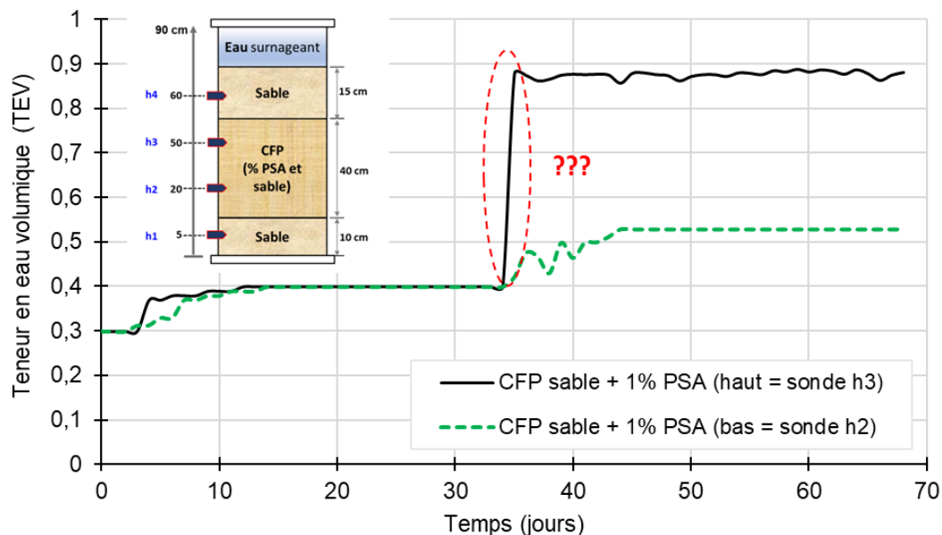
Figure 4.3-1 Évolution de la teneur en eau volumique dans la CFP avec 1% PSA-M85F en fonction du temps écoulé après deux rinçages
