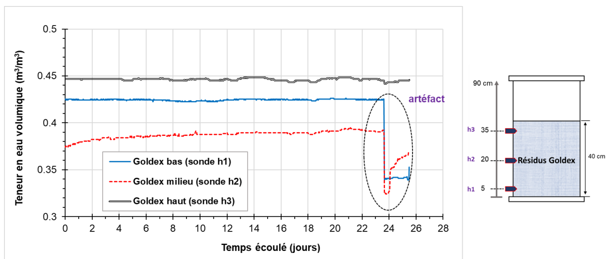
Figure 4.2-9 : Évolution de la teneur en eau volumique (TEV) des résidus miniers fins de la mine Goldex au cours du temps de l'essai
