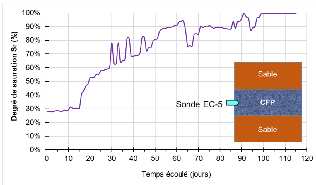
Figure 4.2-8 : Évolution du degré de saturation ( S_r ) de la couche du bris capillaire de la CFP faite de sable et de 0,7% PSA
