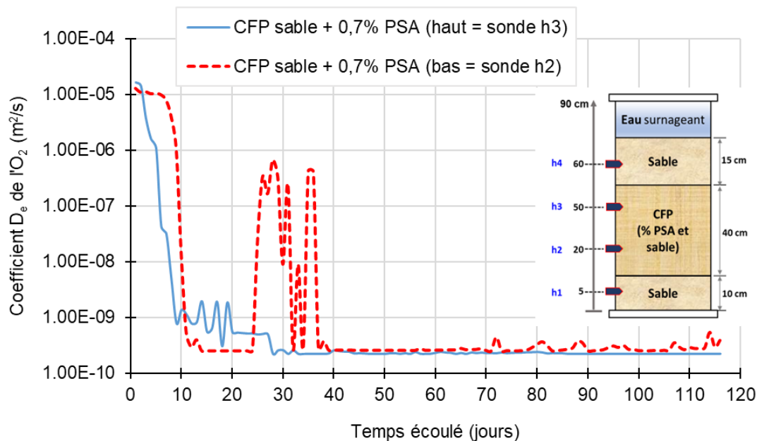
Figure 4.3-6 : Coefficient de diffusion d' O_2 à travers la CFP avec 0,7% PSA en fonction du temps écoulé
