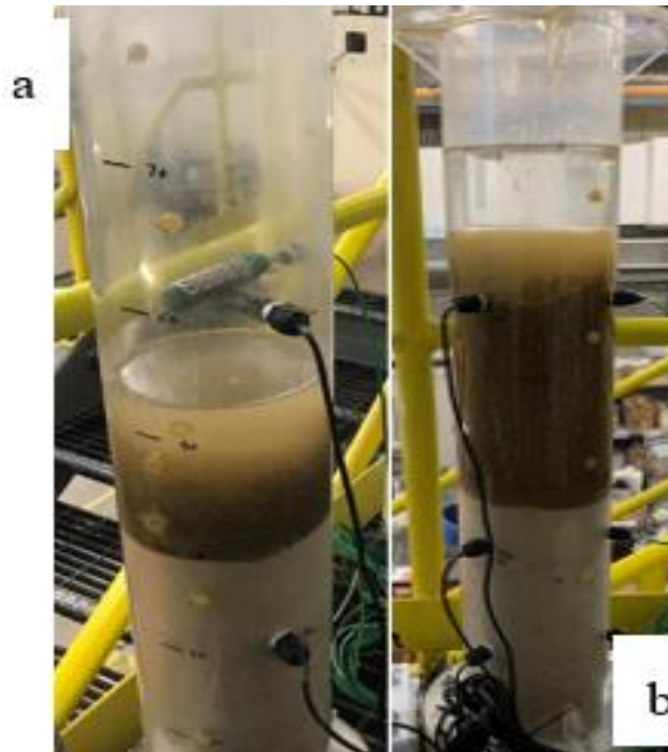
Figure 4.2-3 : Image montrant l'essai en colonne avec le mélange de sable et de 0,5% PSA-M85F : a) à trois jours après le rinçage, b) après quinze jours
