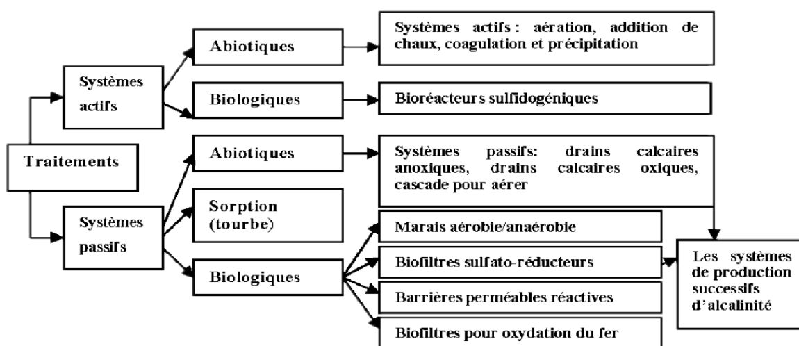
Figure 2.1-2: Stratégie biologique et abiotique de traitement du DMA tiré de (Genty, 2012)
