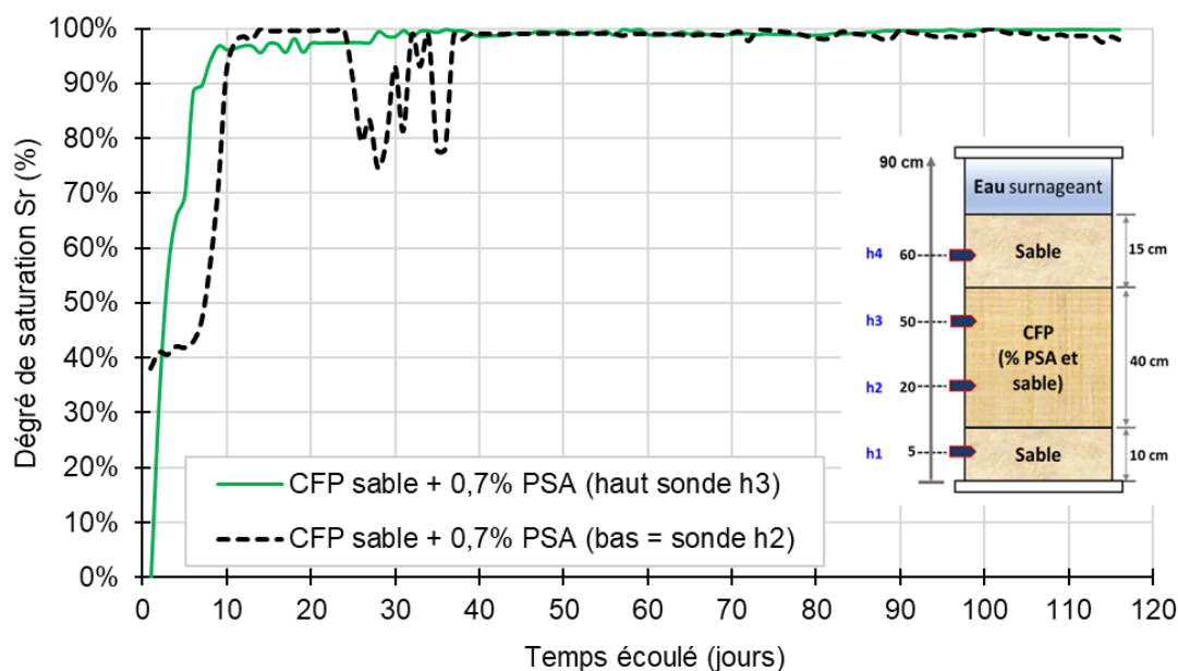
Figure 4.3-5 : Variation du degré de saturation de la CFP avec 0,7% PSA en fonction du temps
