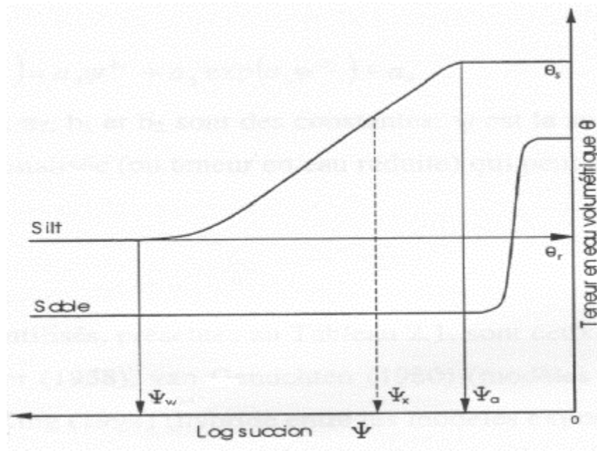
Figure 2.4-2 : Courbes de rétention d'eau typiques pour un sable et un silt (Aubertin et al. , 1995)
