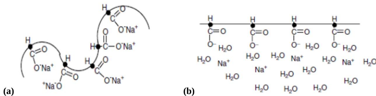
Figure 2.3-1 : Mécanisme d'absorption du polyacrylate de sodium : a) PSA à l'état sec, b) PSA dans l'eau (d'après Hu et al. , 2004)
