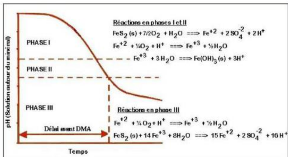
Figure 2.1-1: Étapes de formation du DMA (d'après Kleinman et al. , 1981)
