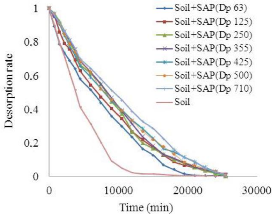
Figure 2.3-3 : Cinétique de désorption de l'eau des grains de PSA de différents diamètres ( D_p ) pré-mélangés avec le sol (d'après Casquilho et al. , 2013)
