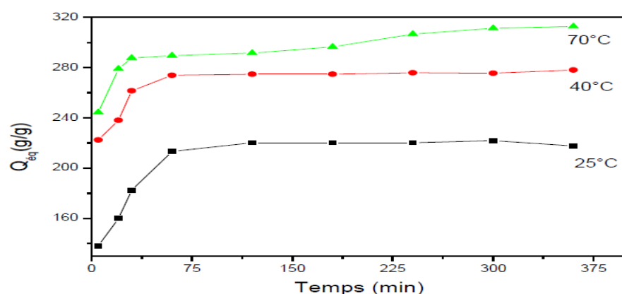
Figure 2.3-6: Effet de la température sur le gonflement du polymère en fonction du temps de contact (d'après Ismi et al. , 2015)
