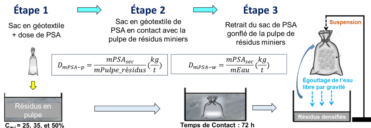
Figure 3.2-1 : Schématisation du protocole de déshumidification des résidus miniers fins en pulpe (adapté de Sahi et al. , 2019)
