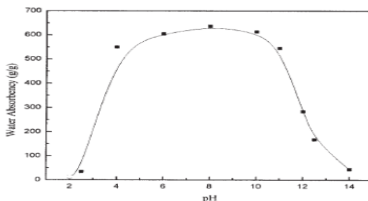
Figure 2.3-7 : Effet du pH sur la capacité d'absorption d'eau du superabsorbant Poly(acide acrylique)/20% Attapulgite (d'après Li et al. , 2004b)
