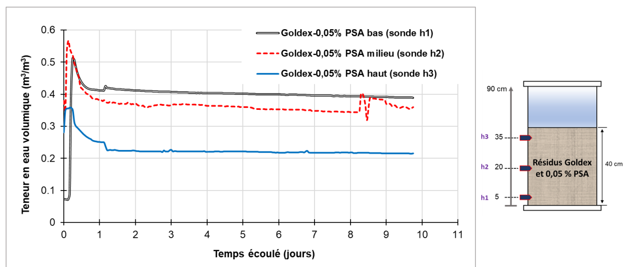
Figure 4.2-10 : Évolution de la teneur en eau volumique du mélange de résidus miniers fins de Goldex et 0,05% PSA fins M85F
