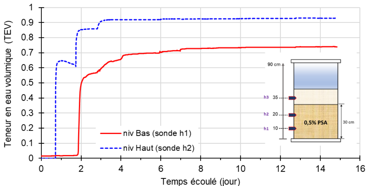
Figure 4.2-5 : Teneur en volumique de la CFP faite de sable et de 0,5% de PSA et à deux niveaux de la couche : niveau bas (sonde h1) et niveau haut (sonde h2)
