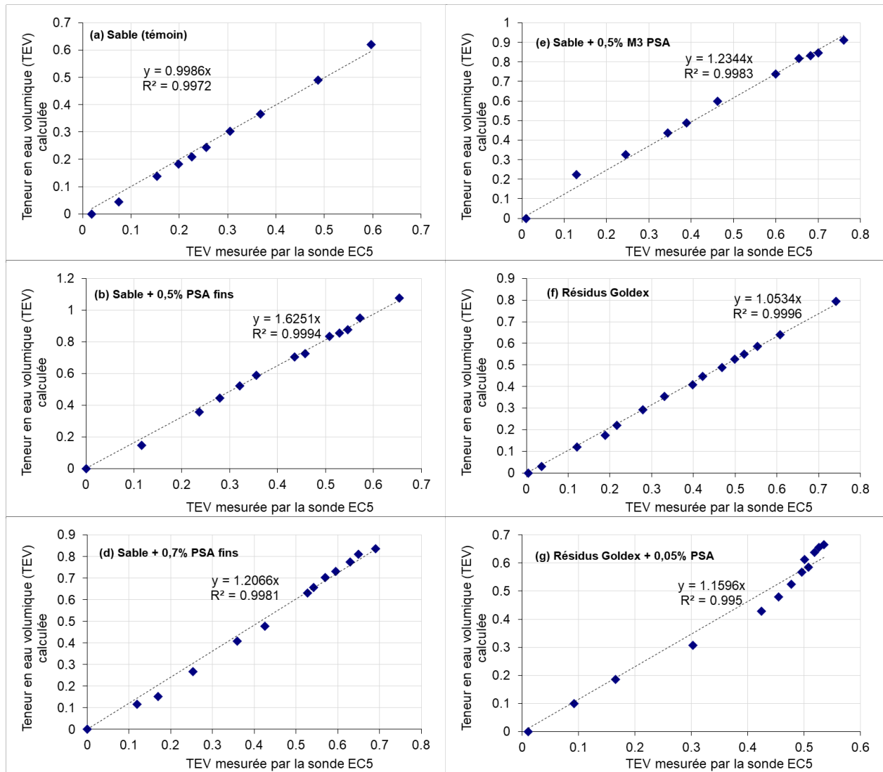
Figure 3.3-10 : Corrélation entre la TEV mesurée par la sonde EC-5 et celle réelle calculée
