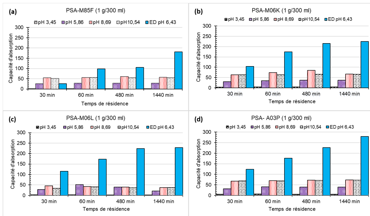
Figure 4.1-5: Capacité d'absorption des PSA en fonction du pH du fluide d'immersion et du temps de résidence
