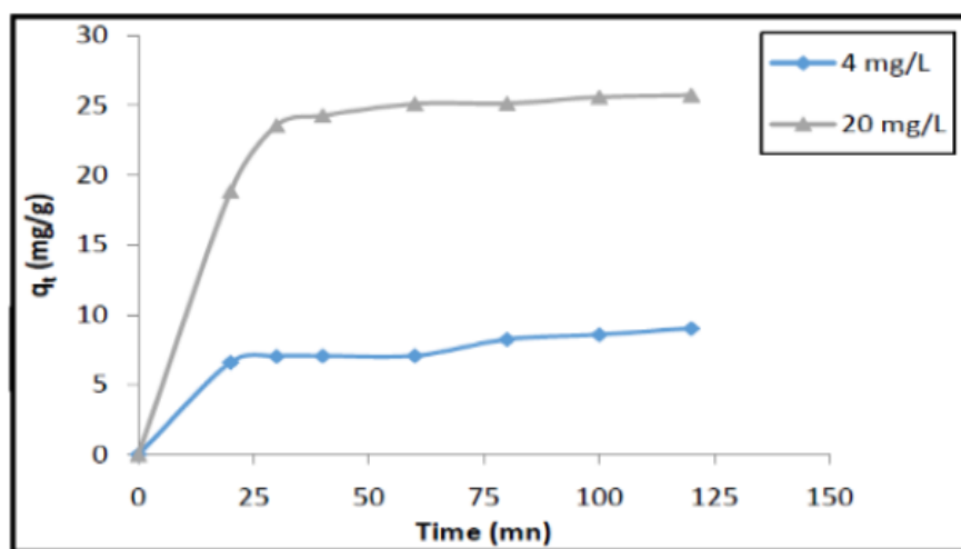
Figure 2.3-9 : Effet de la concentration initiale et du temps de contact sur l'adsorption du Cr(III) par le Polyacrylate de sodium (tiré de Ouass et al. , 2017)
