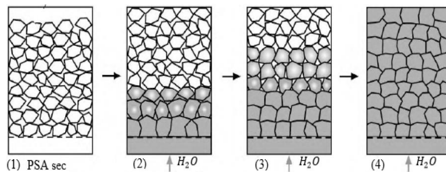
Figure 2.3-4 : Représentation schématique du mécanisme de blocage du gel ou ge-blocking (d'après Wack et al. , 2007)
