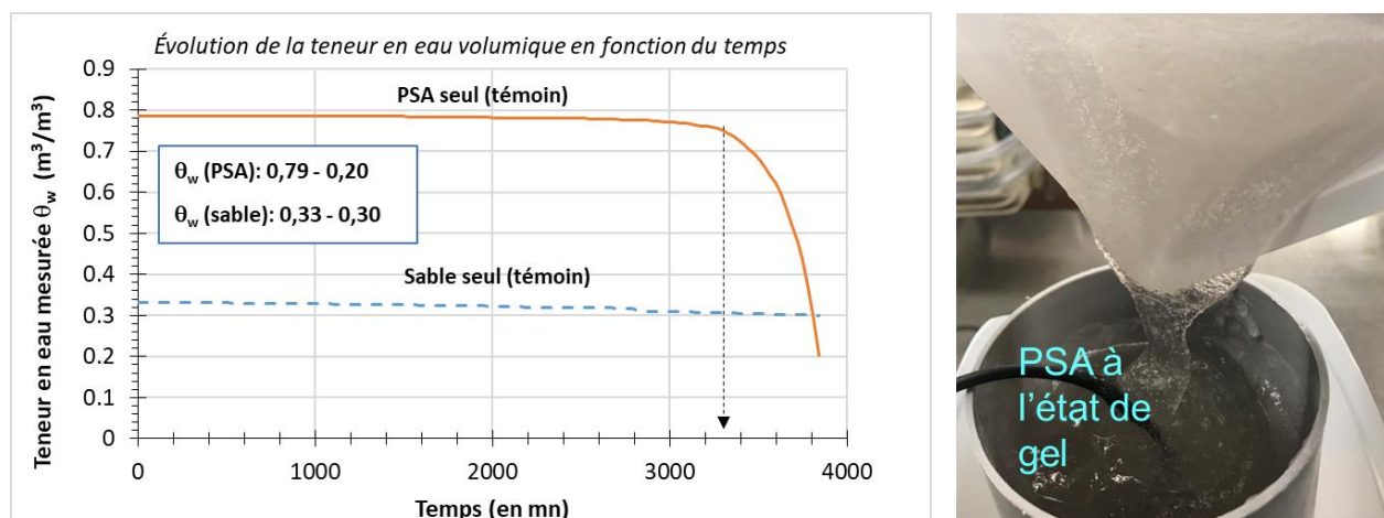
Figure 3.2-3 : Évolution de la teneur en eau volumique des matériaux de base (PSA et Sable)
